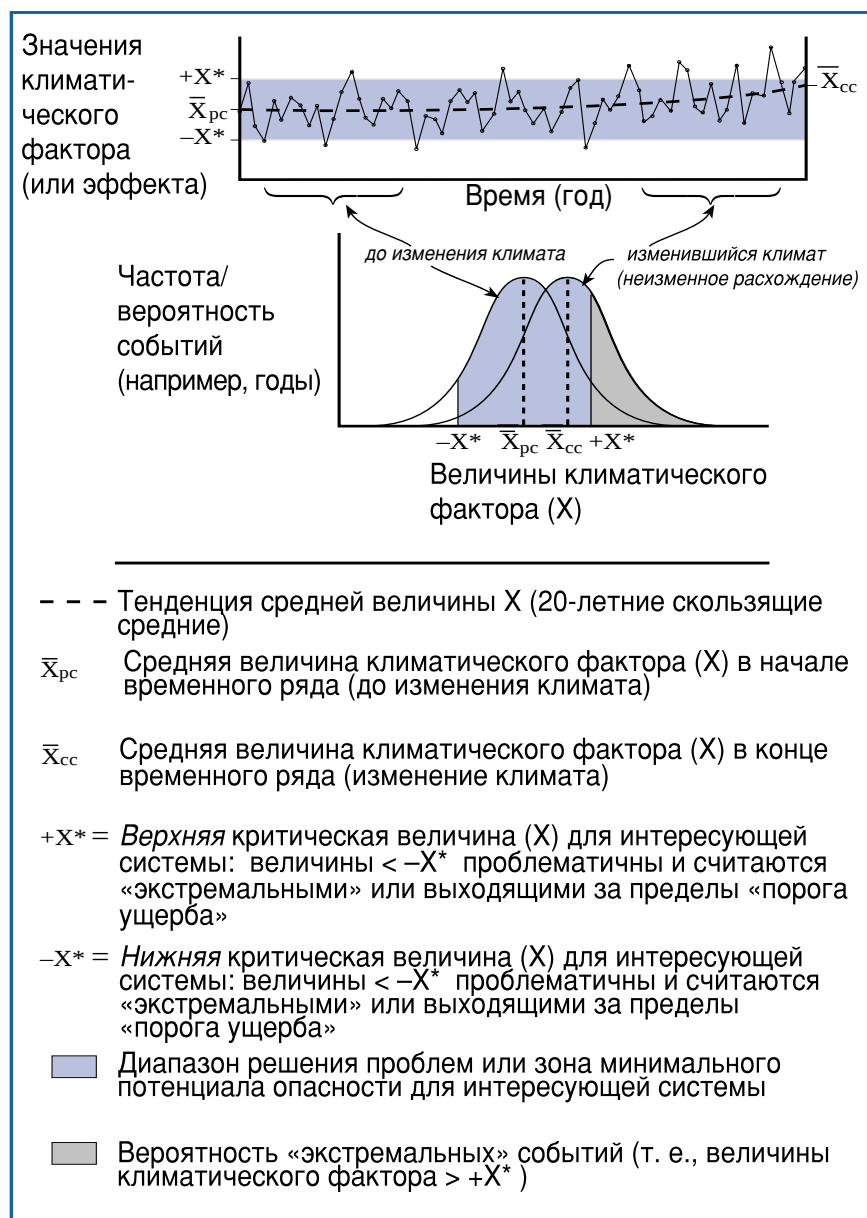
Рисунок TP-10. Изменение климата, изменчивость, экстремальные явления и диапазон допустимости
