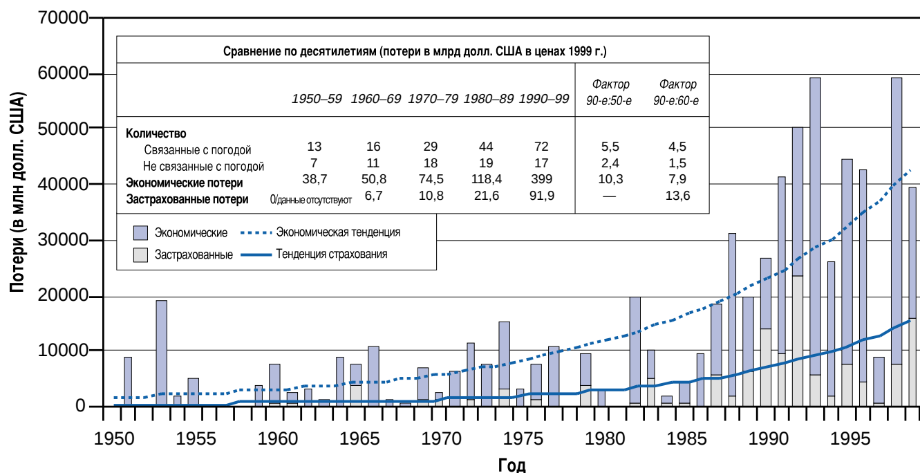
Рисунок ТР-5. Стоимость катастрофических метеорологических явлений характеризовалась быстрой повышательной тенденцией в последние десятилетия. Ежегодные экономические потери от крупномасштабных событий возросли в 10,3 раза — с 4 млрд долл. США в 1950-е годы до 40 млрд долл. США в 1990-е годы (все в долл. США в ценах 1999 г.). В этот же период застрахованная часть этих потерь возросла с незначительного уровня до 9,2 млрд долл. США ежегодно, а соотношение между суммами выплат и потерь от катастрофических событий сократилось на 2/3. Примечательно, что расходы возрастают в два раза в случае включения потерь в результате связанных с погодой явлений некатастрофического характера. Цифры, как правило, включают «захваченных» самостоятельных страховщиков, но не менее формальные виды самостоятельного страхования.
