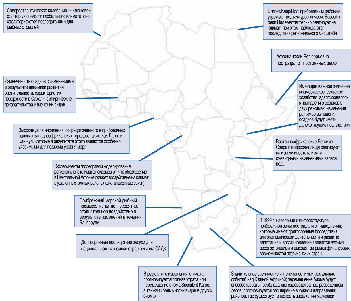
Рисунок ТР-6. Отдельные основные последствия для Африки
