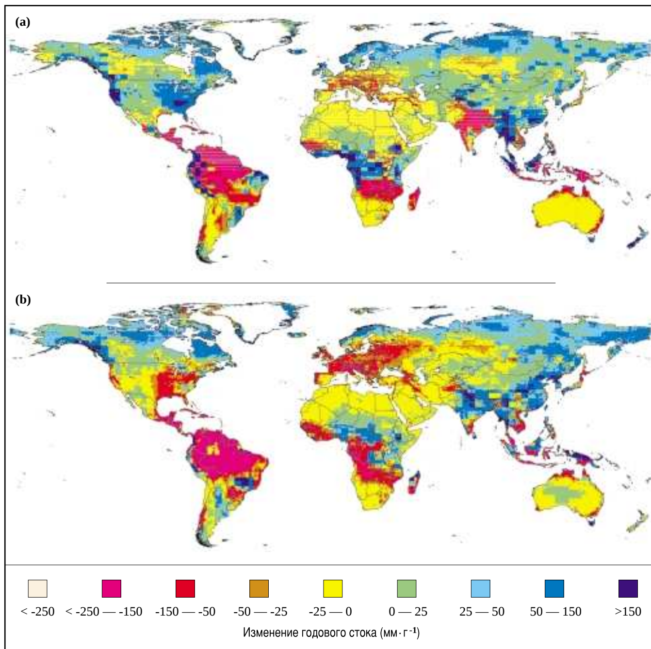
Рисунок ТР-3. Режим изменений стока в значительной мере следует режиму изменений осадков, который меняется в зависимости от климатических моделей. Моделирование увеличения стока, показанные на обеих картах [(а) среднее значение ансамбля HadCM2 и (б) HadCM3; см. раздел 4.3.6.2 главы 4 для обсуждаемых и используемых моделей и сценариев] для высоких широт и Юго-Восточной Азии, и уменьшения в Центральной Азии, в районе вокруг Средиземного моря, в южной части Африки и в Австралии в значительной мере совпадают в плане направления изменений почти во всех климатических моделях. В других районах мира изменения осадков и стока зависят от сценариев изменения климата.
