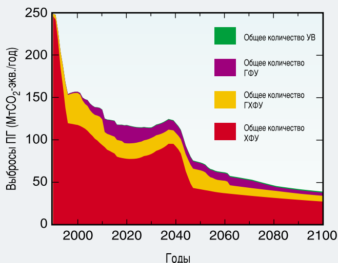
Рисунок ТР-16. Взвешенные по ПГП выбросы пенообразующих веществ в разбивке по группам (1990–2100 гг.) — сценарий обычной практики.
