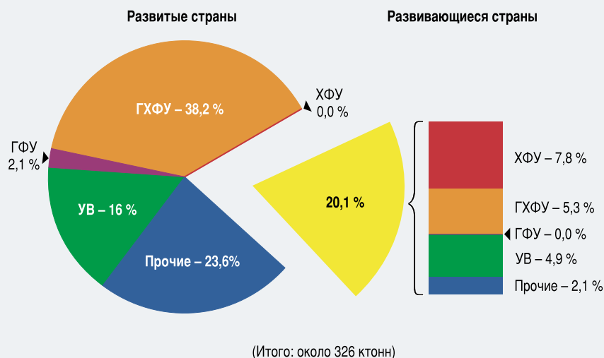
Рисунок ТР-13. Разбивка использования пенообразующих веществ по типу и странам (2001 г.).
