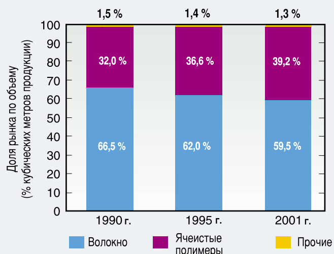
Рисунок ТР-12. Изменение объема изоляционных материалов по типу продукции (1990–2001 гг.) в Европе.
