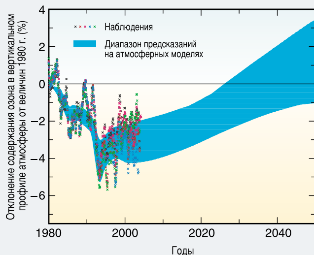
Рисунок ТР-7. Наблюдаемые и смоделированные изменения внесезонного содержания озона в вертикальном профиле атмосферы по сравнению с 1980 г. в низких и средних широтах ( 60^\circ с. ш. – 60^\circ с. ш.). Черные условные обозначения показывают наземные измерения, а цветные условные обозначения — различные комплекты спутниковых данных. Диапазон модельных прогнозов определяется благодаря использованию нескольких разных двухмерных моделей фотохимии, действующих на основе одного и того же сценария галоидоуглеводорода; некоторые модели учитывали также воздействие меняющихся количеств \text{CO}_2 на стратосферные температуры. Измерения показывают, что значения содержания озона в вертикальном профиле атмосферы между 60^\circ ю. ш. и 60^\circ с. ш. стали уменьшаться с начала 1980-х годов, и модели вполне четко зафиксировали сроки и масштабы этого уменьшения. Смоделированные газовые концентрации из галогенных источников уменьшаются в начале XXI века вследствие реакции на Монреальский протокол, поэтому смоделированные значения озона увеличиваются и восстанавливаются до значений в период до 1980 г. [Блок 1.7]
