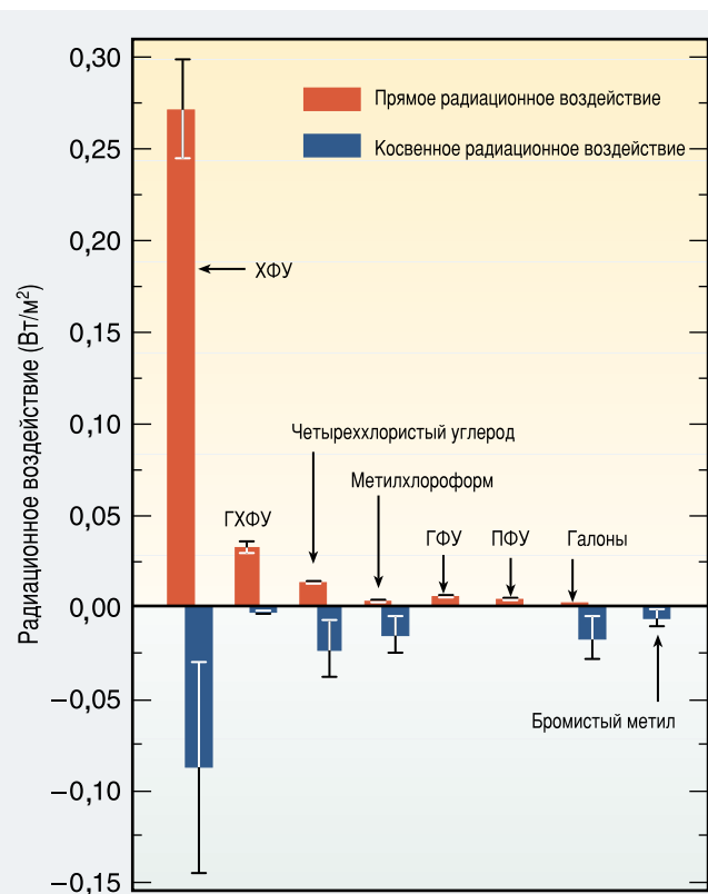
Рисунок РП-2. Прямое и косвенное радиационное воздействие (РВ) вследствие изменений содержания галоидоуглеводородов с 1750 по 2000 гг. 9 Планки погрешностей означают неопределенности величиной \pm 2 среднеквадратических отклонения. [На основе таблицы 1.1]
