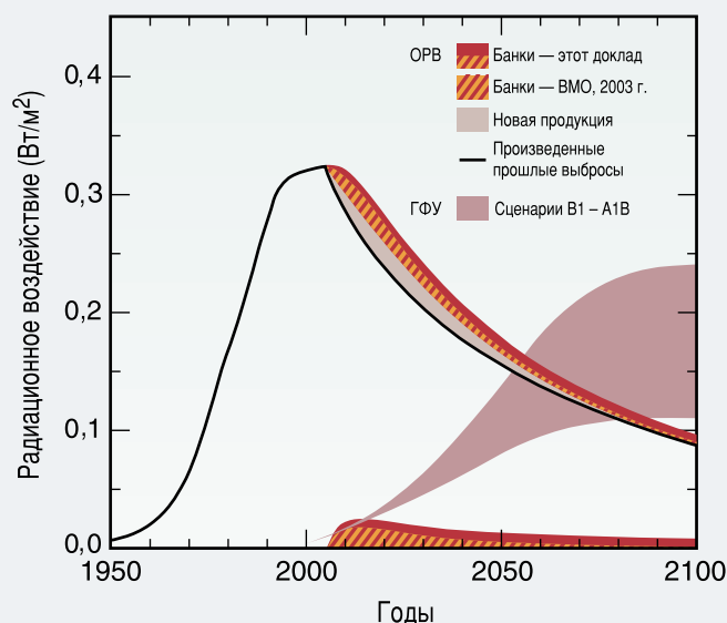
Рисунок ТР-8. Прямое радиационное воздействие всех ОРВ по сравнению с воздействием ГФУ согласно оценкам СРЕС. Прямое радиационное воздействие делится на такие составные элементы, как произведенные прошлые выбросы (сплошная черная линия), выброс разрешенной новой продукции согласно Монреальскому протоколу (серая затененная зона) и выброс банков ОРВ, существовавших в 2004 г. Две оценки приводятся для этих последних выбросов — см. главу 2. Радиационное воздействие, вызванное ГФУ, показано для сценариев В1 и А1В СРЕС (границы красной затененной зоны). Вклад в банки, образовавшийся в результате позднего выпуска ОРВ, показан отдельно и сопоставим с вкладом, который прогнозируется в результате выпуска ГФУ в последующие два десятилетия. ОРВ имеют также другие косвенные последствия для радиационного воздействия. [Рисунок 1.19]
