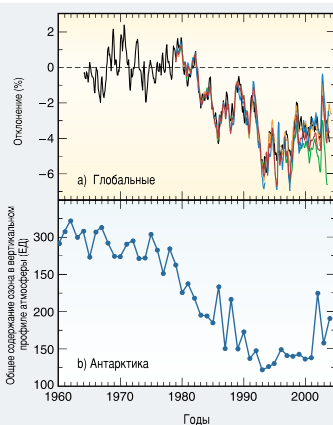
Рисунок ТР-5. Вверху: временной ряд внесезонных глобальных средних аномалий в отношении содержания озона в вертикальном профиле атмосферы, оцененных по пяти разным комплектам данных на основе наземных (черная линия) и спутниковых измерений (цветные линии). Аномалии выражены в виде процента среднего времени за период 1964–1980 гг. Внизу: среднее значение за октябрь суммарных измерений содержания озона в вертикальном профиле атмосферы при помощи спектрофотометра Добсона в Халлее, Антарктика (73,5° ю. ш., 26,7° з. д.). [Рисунки 1.4 и 1.5]
