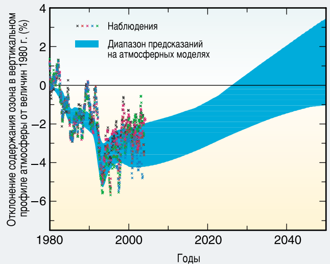
Рисунок РП-3. Наблюдаемые и смоделированные величины содержания озона в вертикальном профиле атмосферы в низких и средних широтах (60° ю. ш. — 60° с. ш.) в виде отклонения в процентах от величин 1980 г. [Блок 1.7]
