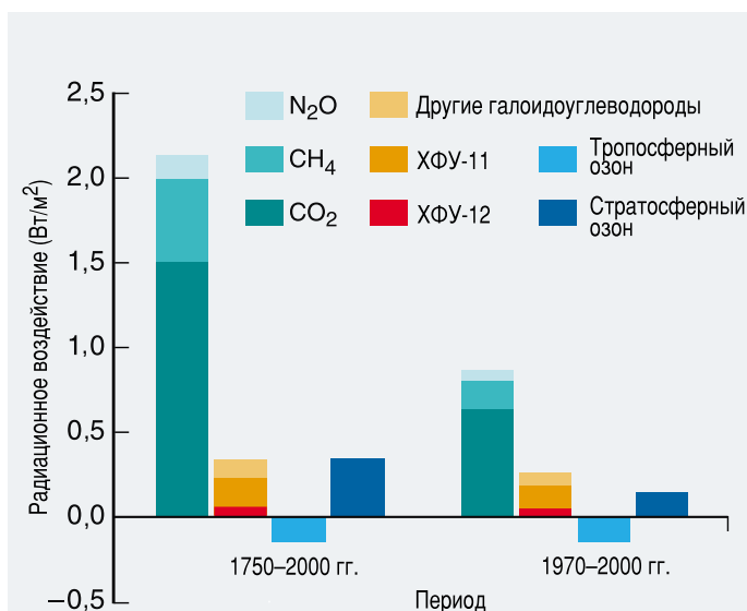
Рисунок ТР-4. Радиационное воздействие ( \text{Вт/м}^2 ), вызванное изменениями хорошо смешанных ПГ и озона во временные периоды 1750–2000 гг. и 1970–2000 гг. Негативное радиационное воздействие стратосферного озона объясняется истощением стратосферного озона в результате выбросов галоидоуглеводорода между 1970 и 2000 гг. В отличие от этого, радиационное воздействие тропосферного озона является в основном независимым от радиационного воздействия галоидоуглеводорода. [Рисунок 1.3]
