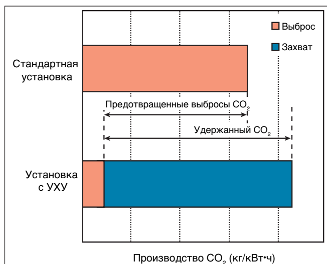
Рисунок РП.2. Улавливание и хранение \text{CO}_2 из энергоустановок. Повышенный объем производства \text{CO}_2 в результате снижения общей эффективности энергоустановок вследствие дополнительной энергии, которая требуется для улавливания, транспортировки и хранения, и любой утечки при транспортировке приводит к большему объему « \text{CO}_2 , производимого на единицу продукции» (нижняя линия) по сравнению с эталонной установкой (верхняя линия) без улавливания (рисунок 8.2).
