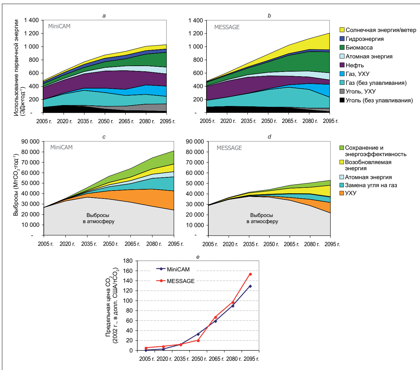
Рисунок РП.7. Эти цифры являются иллюстративными примерами глобального потенциального вклада УХУ как части портфеля мер по смягчению воздействий. Они основаны на двух альтернативных комплексных моделях оценки (MESSAGE и MiniCAM), хотя исходят из тех же самых предположений в отношении главных исходных факторов выбросов. Результаты могут в значительной мере отличаться в региональных масштабах. Этот пример основан на едином сценарии и поэтому не освещает весь диапазон неопределенностей. Секции а и б показывают глобальное использование первичной энергии, включая установку систем УХУ. Секции в и г показывают глобальные выбросы CO 2 серым цветом, а соответствующие вклады основных мер по сокращению выбросов даются в цвете. Секция д показывает расчетную предельную цену сокращений выбросов CO 2 (раздел 8.3.3, блок 8.3).
