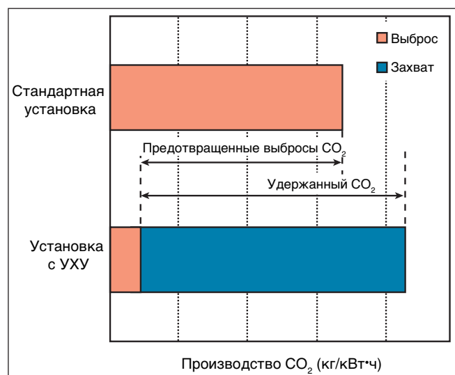
Рисунок ТР.11. Улавливание и хранение CO 2 из энергоустановок. Повышенное производство CO 2 в результате снижения общего КПД энергоустановки вследствие дополнительного расхода энергии на улавливание, транспортировку и хранение, а также любая утечка во время перевозки приводят к увеличению количества «CO 2 , произведенного на единицу продукции» (нижняя черта) по сравнению со стандартной установкой (верхняя черта) без улавливания.
