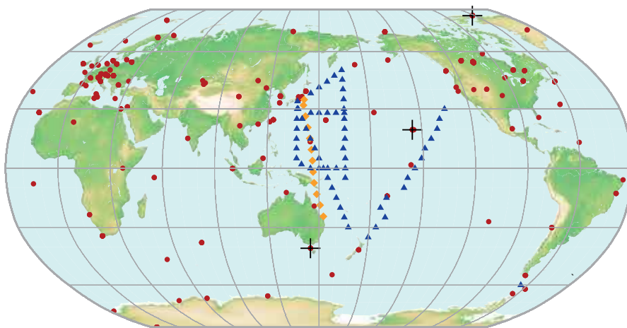
● Наземные измерения ◆ Самолетные измерения ▲ Судовые измерения + Станции сравнения данных по ПГ
