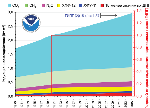
Рисунок 1. Радиационное воздействие ДПГ на атмосферу по сравнению с 1750 г. и обновленный годовой индекс содержания парниковых газов (ГИПГ) НУОА за 2015 г. [8, 9]
