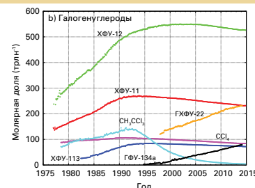
Рисунок 6. Среднемесячная молярная доля гексафторида серы ( \text{SF}_6 ) и наиболее важных галоидоуглеводородов. \text{SF}_6 и галоидоуглеводороды с низкой молярной долей (a) и галоидоуглеводороды с высокой молярной долей (b). Число станций, использованных в анализе, является следующим: \text{SF}_6 (23), ХФУ-11 (24), ХФУ-12 (24), ХФУ-113 (23), \text{CCl}_4 (21), \text{CH}_3\text{CCl}_3 (23), ГХФУ-141b (9), ГХФУ-142b (13), ГХФУ-22 (13), ГФУ-134a (9), ГФУ-152a (8).
