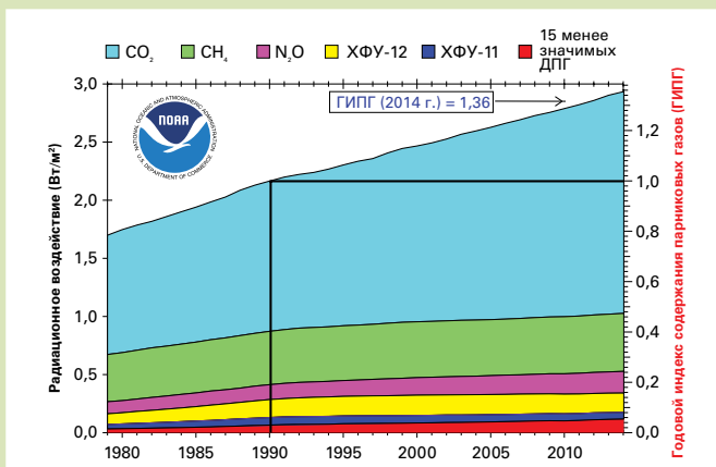
Рисунок 1. Радиационное воздействие ДПГ на атмосферу по сравнению с 1750 г. и обновленный годовой индекс содержания парниковых газов (ГИПГ) НУОА за 2014 г.
