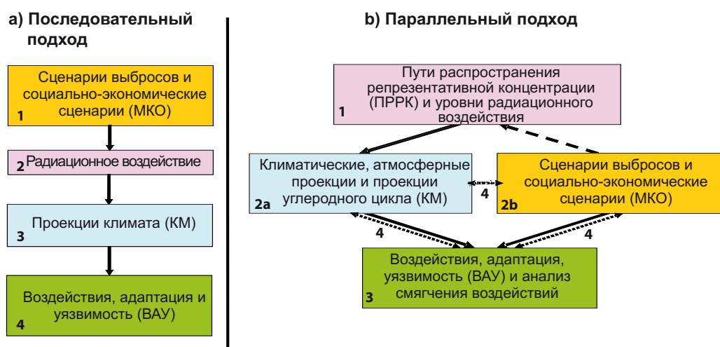
Рисунок 1. Подходы к разработке глобальных сценариев: а) предыдущий последовательный подход; б) предлагаемый параллельный подход. Номера указывают этапы аналитической работы (2a и 2b осуществляются одновременно). Стрелки указывают передачу информации (сплошная стрелка), выбор ПРРК (пунктир) и интеграция информации и обратные связи (стрелки, изображенные точками).
