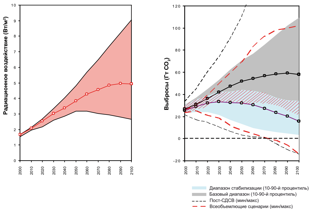
Рисунок 4. Полный диапазон и медиана путей распространения радиационного воздействия полного охвата (левая часть) и пути распространения выбросов \text{CO}_2 для различных диапазонов и медиан (правая часть). В правой части линии, соединяющие заштрихованные и незаштрихованные окружности, представляют собой диапазон соответственно базовых сценариев и сценариев стабилизации. Красные пунктирные линии обозначают полный диапазон путей распространения выбросов \text{CO}_2 предприятиями энергетики и промышленности, которые ассоциируют с всеобъемлющими сценариями в левой части. Данные, опубликованные по этим сценариям, рассчитаны лишь до 2100 г.; для ПРРК потребуется распространить данные на период до 2300 г. 9
