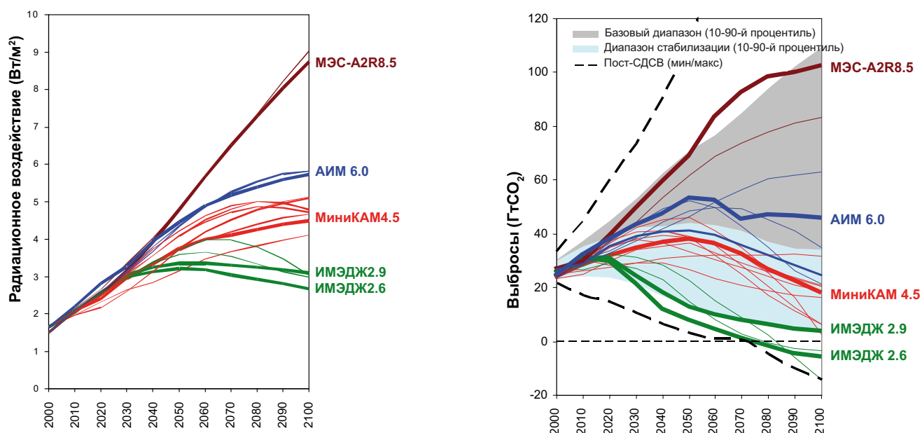
Рисунок 5. Радиационное воздействие в сравнении с доиндустриальными выбросами \text{CO}_2 (левая часть) и выбросами \text{CO}_2 энергетики и промышленности (правая часть) для ПРРК – кандидатов (цветные линии) и для максимальных и минимальных (пунктиром) значений и 10-90-го процентилей (затемненная зона), фигурирующих в литературе после СДСВ. Эти процентиля отражают частотное распределение существующих сценариев, и их нельзя рассматривать как вероятности. Голубая зона указывает на сценарии снижения остроты воздействия; серая зона – на базовые сценарии 14 .
