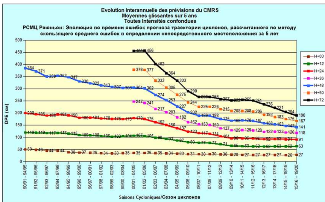
Рисунок 7. Эволюция во времени ошибок прогноза траектории циклонов в юго-западной части Индийского океана (км), рассчитанного по методу скользящего среднего за 5 лет (Метео-Франс, Реюньон, 2022)
