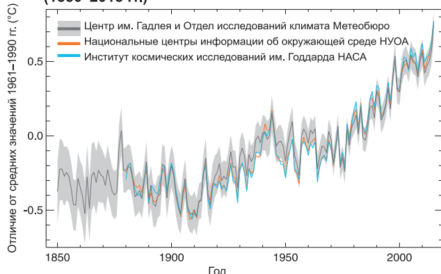
Глобальные аномалии среднегодовых температур (1850–2015 гг.)
