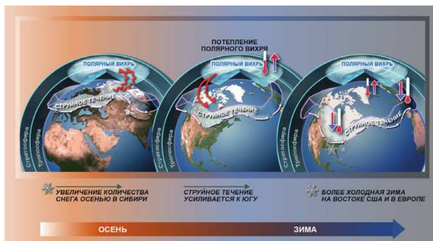
Схема взаимодействия стратосферы и тропосферы зимой. (Слева)
