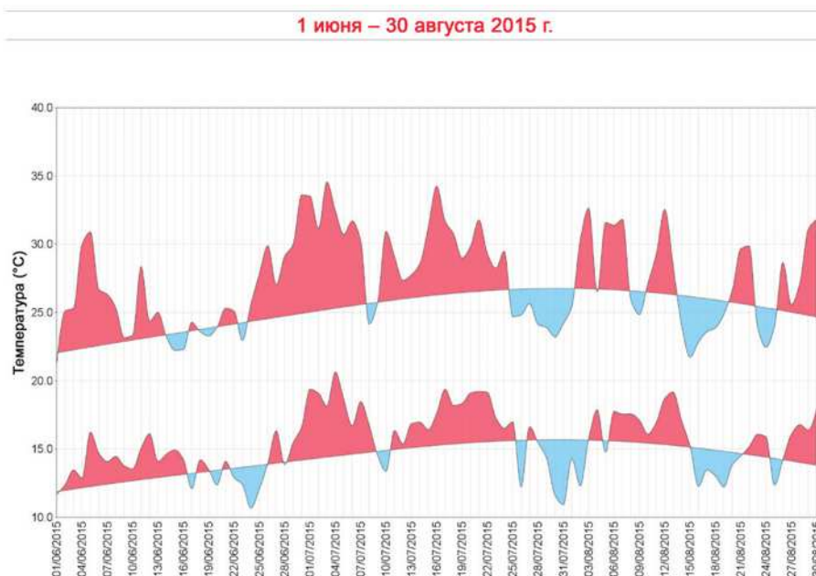
Суточные временные ряды максимальной (верхняя кривая) и минимальной (нижняя кривая) температуры во Франции (среднее значение по 30 станциям) за период с 1 июня по 30 августа 2015 г. (Источник: Метеорологическая служба Франции)
