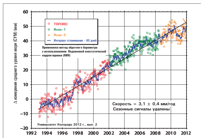
Подъем глобального уровня моря в период 1992–2012 гг. по данным наблюдений со спутников ТОПЭКС/Посейдон и Ясон
