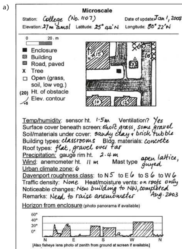
Рисунок 9.7. Информация, требуемая для описания микромасштаба окружения городской климатической станции; (а) шаблон для файла метаданных; (b) пример фотоснимка объективом типа «рыбий глаз» уличного каньона иллюстрирует закрытость горизонта и (с) полусферический рефлектор Метеорологического бюро СК, расположенный на дождемере.
