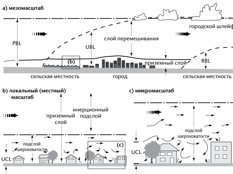
Рисунок 9.1. Схема климатических масштабов и вертикальных слоев атмосферы городских районов: планетарный пограничный слой (PBL (ППС)), городской пограничный слой (UBL (ГПС)), городской пологовый слой (UCL (ГПС)), пограничный слой сельской местности (RBL (ПСС)) (переработано по работе Оке, 1997).
