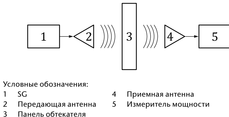
Рисунок А.20. Схема измерения потерь на пропускание обтекателя на испытательном полигоне
