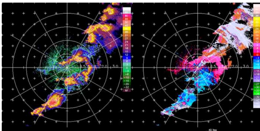
Рисунок 7.14. Для восстановления вторичного эхосигнала применяется множество методик, связанных с ЧПИ, при этом не проводится дополнительная обработка кодированного по фазе сигнала. Для пространственной локализации интенсивности эхосигнала используются сканирования с низкой ЧПИ, действующие на большой дальности. Для измерения радиальной скорости используется сканирование с высокой ЧПИ, но на малом расстоянии. Радиальная скорость привязана к элементу разрешения по дальности при наивысшей мощности.
