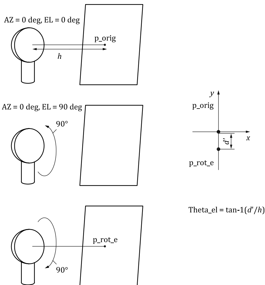
Рисунок А.31. Точность ориентации антенны (EL)
