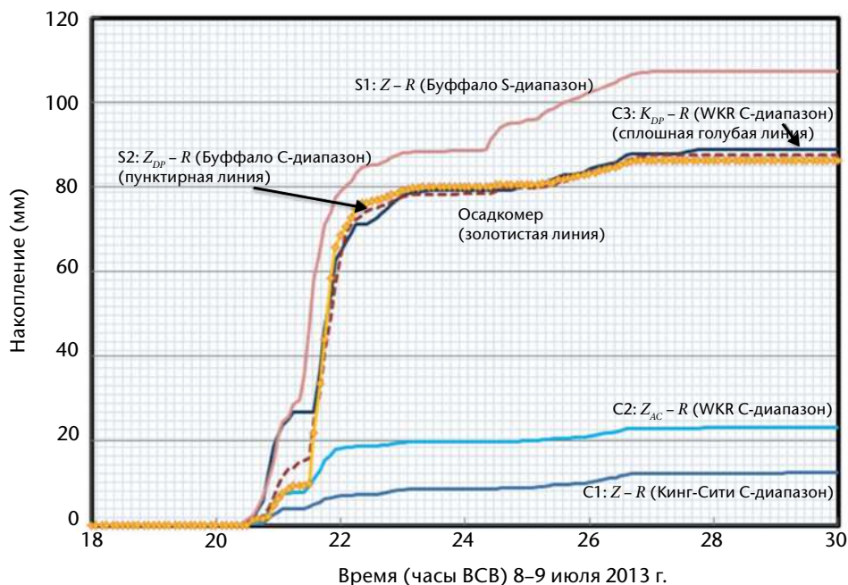
Рисунок 7.37. Метеограмма накопленных дождевых осадков, составленная по показаниям осадкомера (желтая линия с условными обозначениями), и оценки аккумулярованных осадков — три в С-диапазоне (C1, C2, C3) и две в S-диапазоне (S1, S2) — с использованием разнообразных методов разнесения в диапазонах для одного места размещения осадкомерных пунктов; пункт находится приблизительно в 7 км к юго-западу от центра (см. также рисунок 7.36, любезно предоставленный Судешом Буду из Министерства окружающей среды Канады.
