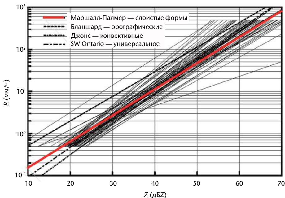
Рисунок 7.35. Графическое изображение множества соотношений Z - R из работы Battan (1973).
