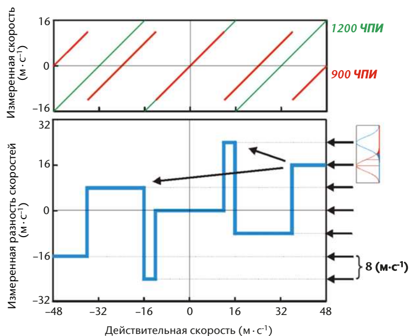
Рисунок 7.10. Это пример радиолокатора С-диапазона, работающего в импульсном режиме 900 и 1 200 \text{с}^{-1} при однозначных скоростях Найквиста 12 и 16 \text{ м} \cdot \text{с}^{-1} соответственно. В основе данного метода лежит разность между измеренными радиальными скоростями (ордината на нижнем изображении), служащая для определения кратного числа (абсцисса на нижнем изображении) и его последующего использования с соответствующей измеренной радиальной скоростью для оценки истинной радиальной скорости.
