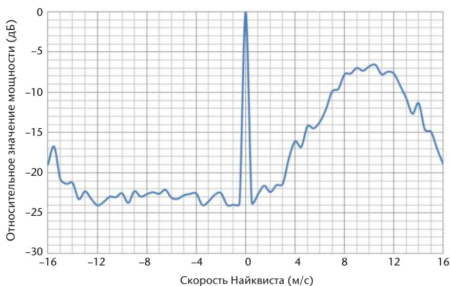
Рисунок 7.6. Этот доплеровский спектр показывает распределение мощности в пределах объема единого радиолокационного импульса как функции доплеровской скорости.
