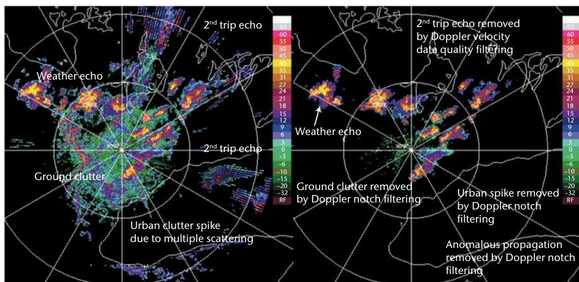
Рисунок 7.7. Современные доплеровские радиолокаторы могут фильтровать неверные данные или отражения от земли на этапе технологической цепочки, связанном с обработкой сигналов. На левом изображении показаны необработанные данные, а на правом — способность фильтрации доплеровского сигнала и обработки данных. На рисунке 7.29 показана возможность многовариантности поляризации для обеспечения качества данных.
