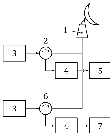
Рисунок 7.А.4 Системная схема распределительного излучателя с двойной поляризацией плюс дополнительный режим линейного коэффициента деполяризации
