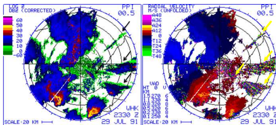
Рисунок 7.12. Пример вторичных эхосигналов, связанных с отражаемостью (слева) и радиальной скоростью (справа), для магнетронного радиолокатора.
