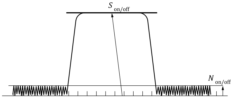
Рисунок А.15. Измерение коэффициента усиления сжатия импульсов
