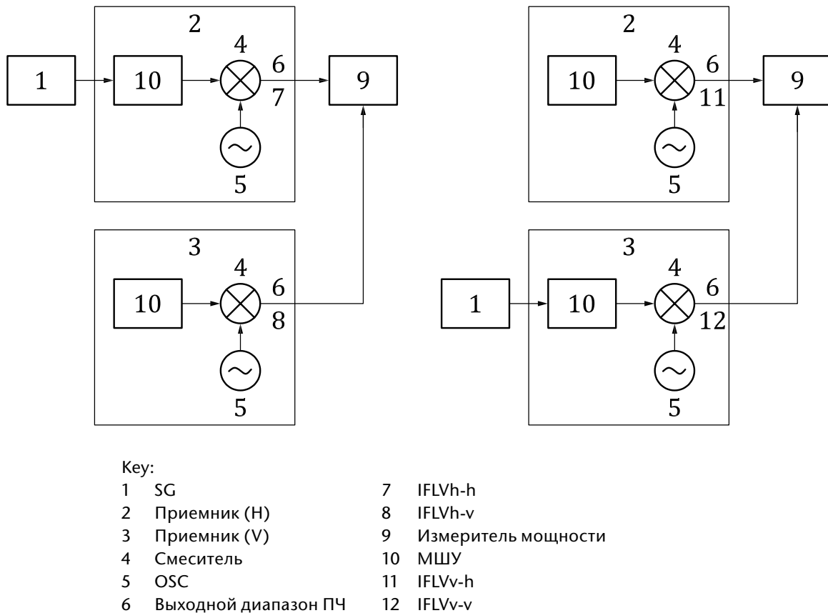
Рисунок А.8. Измерение изоляции Н/В
