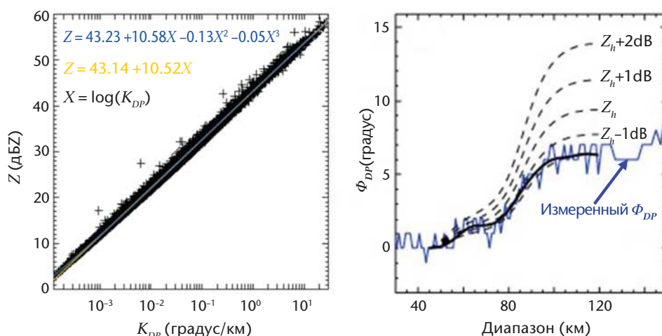
Рисунок 7.17. Существует тесная взаимосвязь между отражаемостью и конкретной дифференциальной фазой ( Z и K_{DP} ). На левом рисунке эта взаимосвязь показана по данным измерения дисдрометра. На правом рисунке показано одно радиальное направление данных со значительной дифференциальной фазой. Посредством корректировки отражаемости и перерасчета дифференциальной фазы можно осуществить последовательную калибровку радиолокатора (рисунки любезно предоставлены Isztar Zawadzki ).
