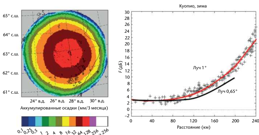
Рис. 7.33. На этом рисунке показаны аккумулярованные за зимний сезон суммы осадков, рассчитанные по данным радиолокатора. Описание годового режима осадков объясняется, в первую очередь, отсутствием заполнения луча на дальних расстояниях для приземных метеорологических систем. На изображении справа показано, каким образом это представляется в виде погрешности определения дальности путем сравнения данных датчиков радиолокатора (рисунок любезно предоставлен Даниэлем Микельсоном из Шведского метеорологического и гидрологического института, а также использованы данные, предоставленные Финским метеорологическим институтом).
