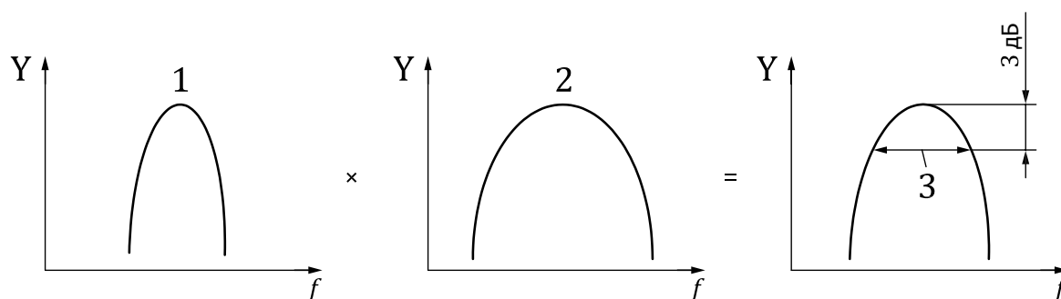
Рисунок А.12. Диаграмма измерения полосы пропускания для радиолокатора со сжатием импульсов
