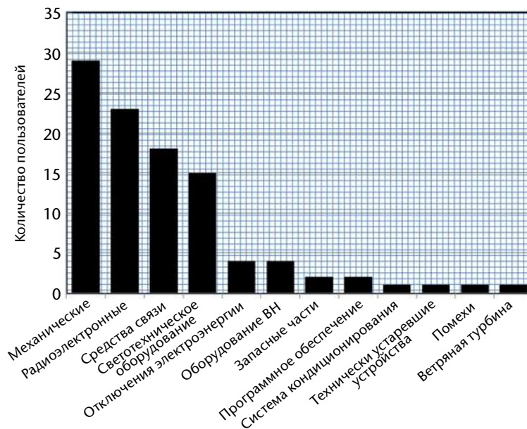
Рисунок 7.16. Результаты проведенного ВМО обзора метеорологических радиолокаторов, показывающие основные отказные режимы радиолокатора (Sireci et al, 2010); рисунок любезно предоставлен Oguzhan Sireci из Турецкой государственной метеорологической службы.
