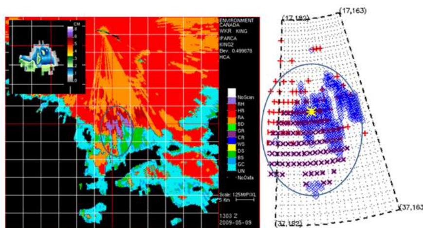
Рисунок 7.29. Приведенная иллюстрация — это отражательность, основанная на данных о размере градин, а большое изображение — продукт поляризационного разнесения для идентификации типа осадков, включая град. Изображение справа содержит подробный анализ этого примера. Рисунок любезно предоставлен Судеш Буда из Министерства окружающей среды Канады.
