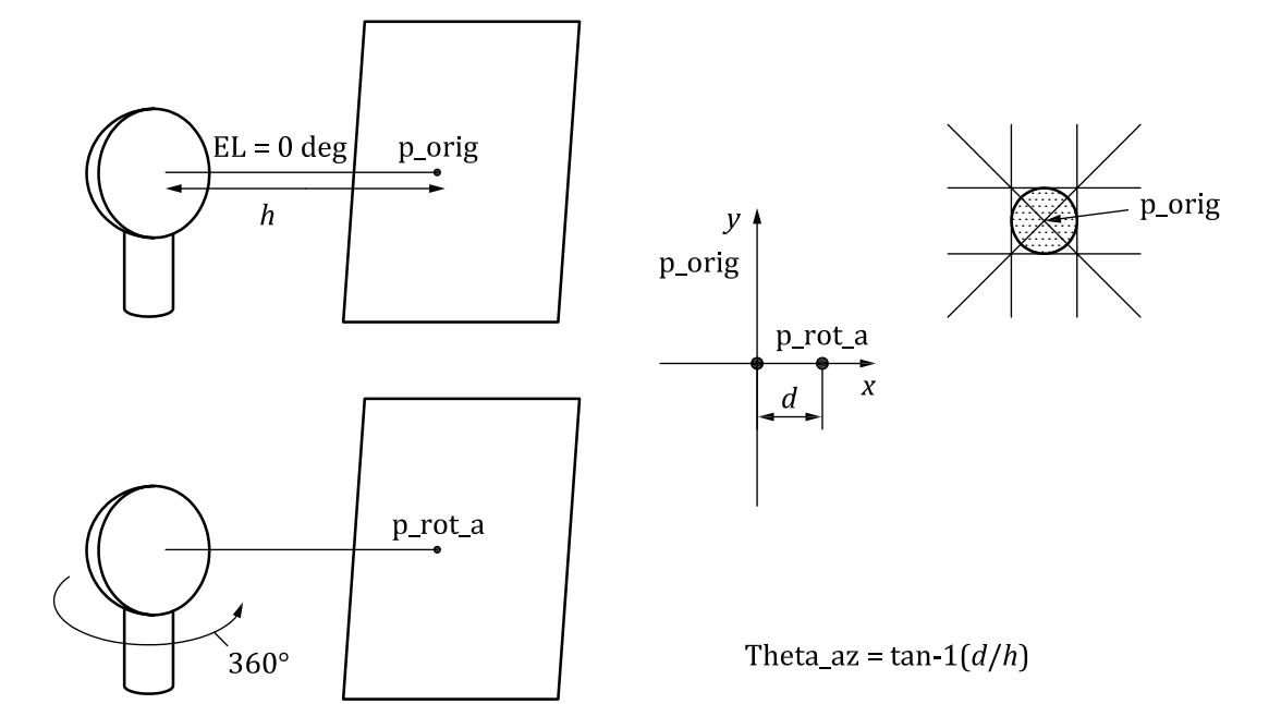
Рисунок A.30. Точность ориентации антенны (AZ)
