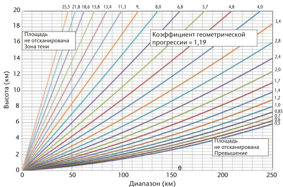
Рисунок 7.4. Диаграмма высоты луча также является полезным инструментом для интерпретации радиолокационной продукции. Высота луча вычерчивается относительно плоской Земли, что является более традиционным представлением. Последовательность углов места — это последовательность, предложенная Маршаллом и Баллантайном (1978 г.) для получения оптимальной горизонтальной продукции (CAPPI's, верхние точки эхосигналов).
