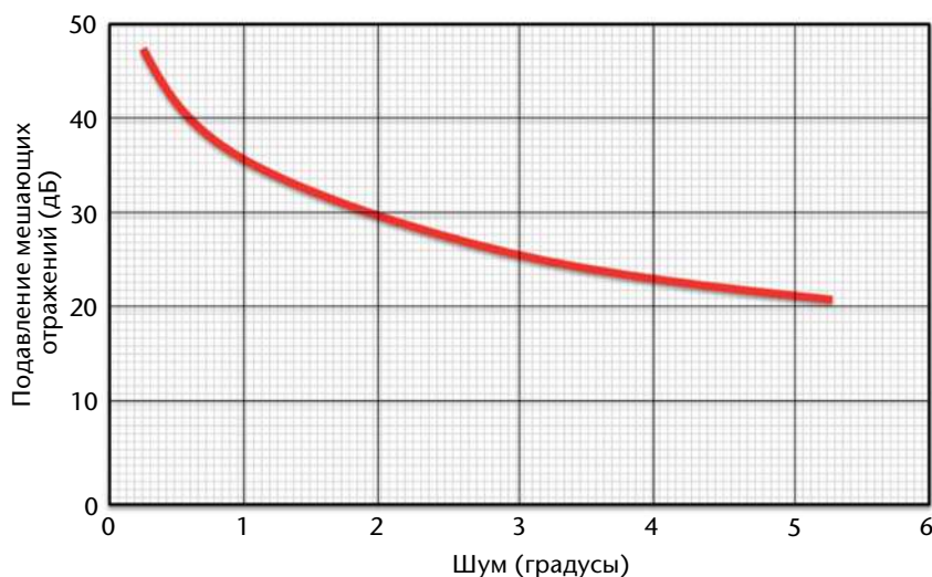
Рисунок 7.15. Когерентность (фазовый шум) — это мера качества работы доплеровского радиолокатора, и она непосредственно связана со способностью удалять помехи, вызванные отражением от земной поверхности, и способностью восстанавливать вторичные эхосигналы, используя методику кодирования по фазе.
