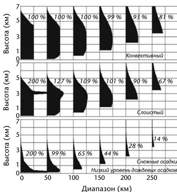
Рисунок 7.32. Сглаживание луча и характер его распространения изменяют внешний вид вертикального профиля отражаемости по мере изменения дальности. Показаны три ситуации с максимальной отражаемостью в вертикальном столбе атмосферы в виде процентной доли выпадения осадков на поверхность суши, при этом учитывается яркая полоса (заимствовано из работы Joss and Waldvogel, 1990).
