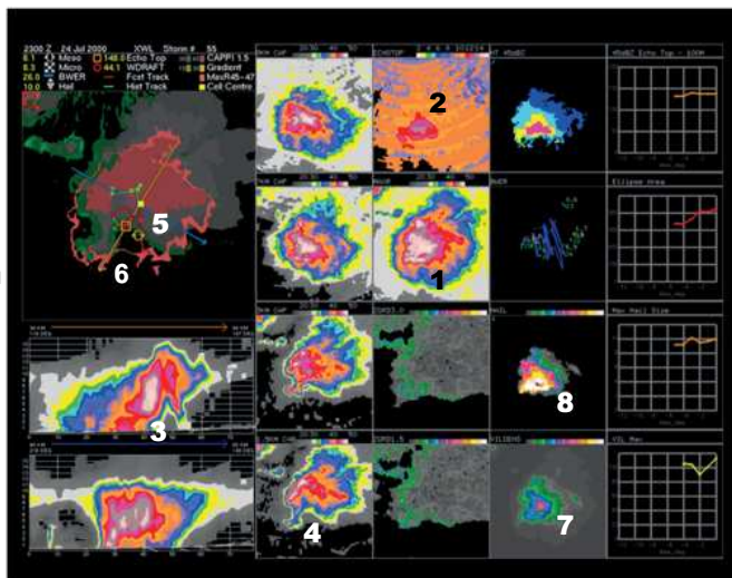
Рис. 7.24. Методики предупреждений сильных штормов перечислены слева (Lemon, 1978). Продукция вида ячейки — это изображение, в центре которого находится ячейка обнаруживаемой в автоматическом режиме грозы и которое показывает соответствующую продукцию для принятия решения (число ячейки соответствует номеру списка).
