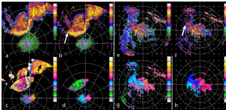
Рисунок 7.13. Пример увеличения дальности обнаружения с использованием случайной фазы: Пример слева (a-d) показывает ситуацию, при которой первичный эхосигнал является слабым, а вторичный сигнал в значительной степени может быть восстановлен. В правой части этого примера (e-h) показан сильный первичный эхосигнал, который исключает возможность восстановления вторичного эхосигнала.
