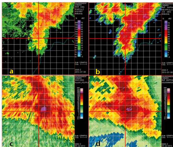
Рисунок 7.36. На верхних рисунках показано ослабление сигнала радиолокатора С-диапазона (а) по сравнению с радиолокатором S-диапазона (b) в фиксированный момент времени. На нижних рисунках представлены аккумуляции осадков равномерно в течение всего периода явления и продемонстрировано поразительное сходство после введения поправок с использованием метода поляризационного разнесения (см. также рисунок 7.37, любезно предоставленный Судешом Буду из Министерства окружающей среды Канады).
