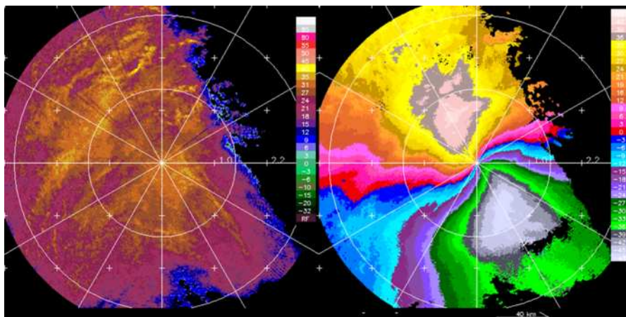
Рис. 7.11. На этом рисунке показана необходимость и способность увеличения скорости радиолокатором С-диапазона по меньшей мере до 48 \text{ м} \cdot \text{с}^{-1} . Речь идет в данном случае об урагане/внетропическом переходном участке траектории и скоростях порядка 48 \text{ м} \cdot \text{с}^{-1} . В подобной ситуации соблюдаются допущения, предусмотренные методом использования частоты повторения двойных импульсов (две измеренные расчетные скорости на разных ЧПИ являются производной той же самой радиальной скорости), и результат характеризуется незначительным шумом (изображение справа, сравнить с рисунком 7.20).
