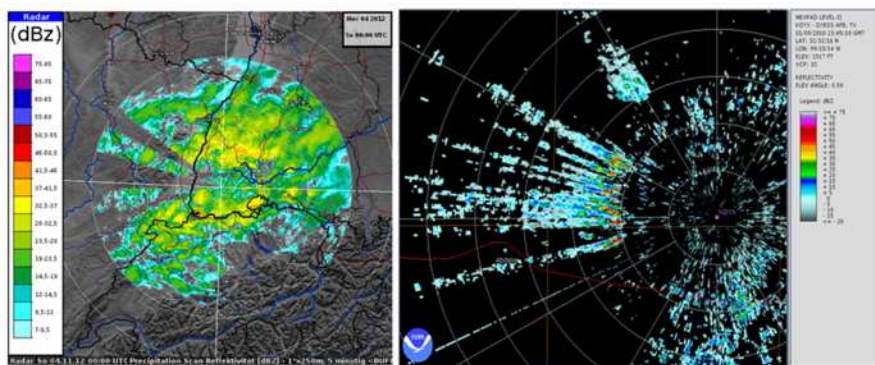
Рисунок 7.23. На изображении слева (любезно предоставлено Метеорологической службой Германии) показано затенение (к западу от радиолокатора) ветряными турбинами, а на изображении справа показаны помехи и эффекты множественного рассеяния ветряными турбинами (любезно предоставлено Национальным управлением по исследованию океана и атмосферы).
