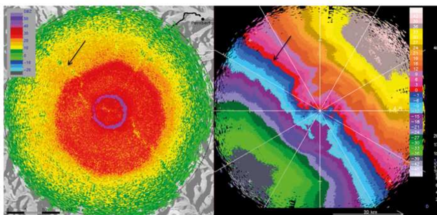
Рисунок 7.9. Режекторная доплеровская фильтрация может удалять слишком много эхосигналов, когда доплеровский спектр метеосигналов узок и при почти нулевой доплеровской скорости (см. стрелку). Эта проблема является незначительной по сравнению с другими ложными сигналами, показанными на рисунке 7.2.
