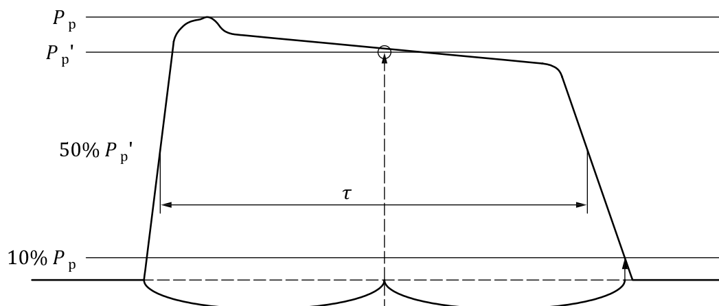
Рисунок А.2. Определение ширины импульса
