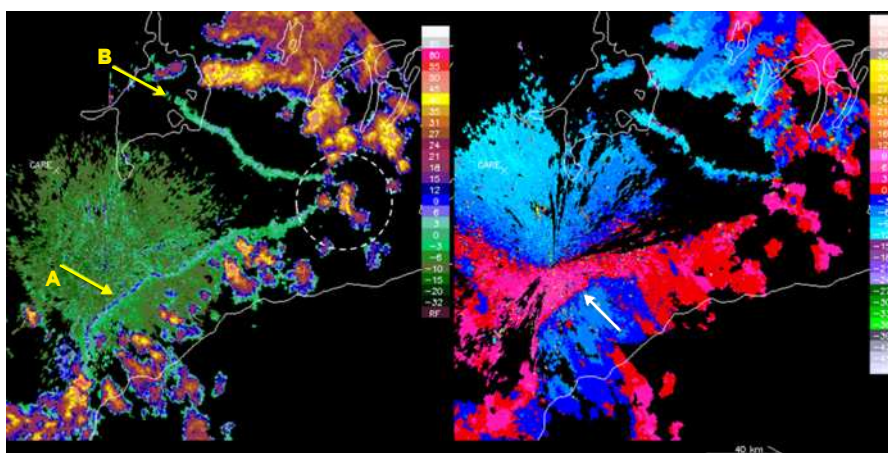
Рисунок 7.31. Современные радиолокаторы достаточно чувствительны для того, чтобы видеть озерный бриз и оттоки воздуха из зоны грозы (А и В соответственно, изображение слева). Точки взаимопересечения являются местами ускоренного подъема и соответственно местами потенциального развития конвективных образований (см. явление образования шторма внутри штрихового круга белого цвета).
