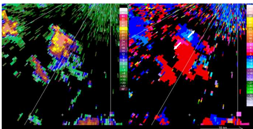
Рисунок 7.27. Нисходящий микровихрь (микро- или макро-) наблюдается в виде пары радиальных скоростей в обратном/прямом направлении, выравненных вдоль радиального вектора (см. стрелки на правом изображении). Это представляет собой быстро меняющуюся характеристику гроз и может быть следствием самых обычных и небольших гроз.
