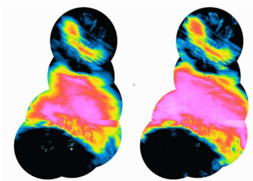
Рисунок 7.34. Этот рисунок показывает случай стационарного атмосферного фронта, ориентированного по направлению восток-запад. На изображении слева показано резкое снижение по мере увеличения дальности (см. рисунок 7.33). На изображении справа показана внесенная в данные корректировка дальности (рисунок любезно предоставлен Ярмо Коистиненом, Финский метеорологический институт).
