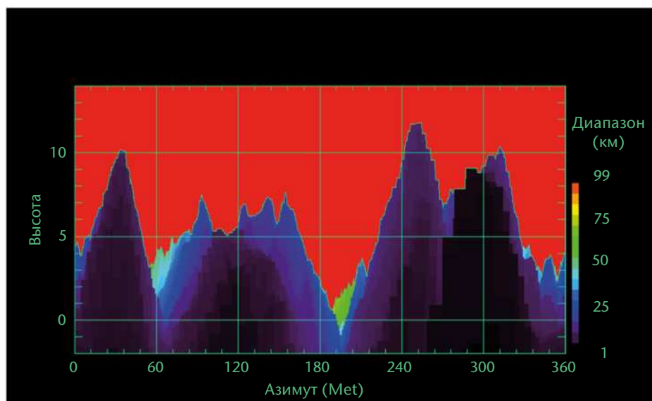
Рисунок 7.18. Глобальные данные цифровой модели рельефа (ЦМР) имеются и являются достаточно точными для их использования с целью оценки и определения места установки метеорологического радиолокатора. Изображение показывает расстояние, на котором могут быть собраны полезные данные, при этом учитываются азимут и угол места.
