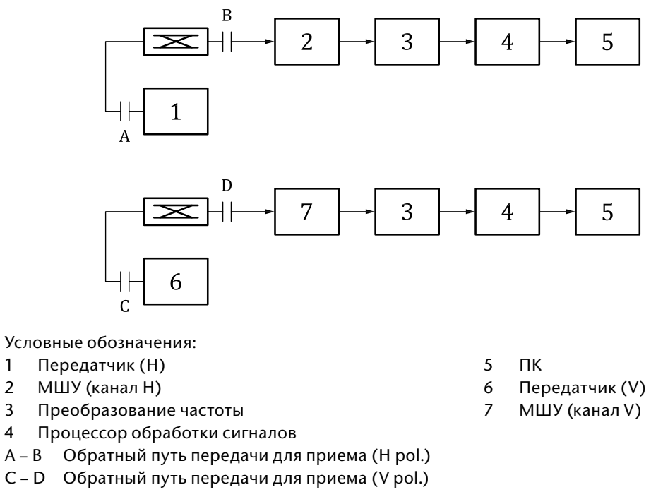
Рисунок А.22. Схема измерения потерь передающего и приемного трактов в случае независимого передатчика с двойной поляризацией
