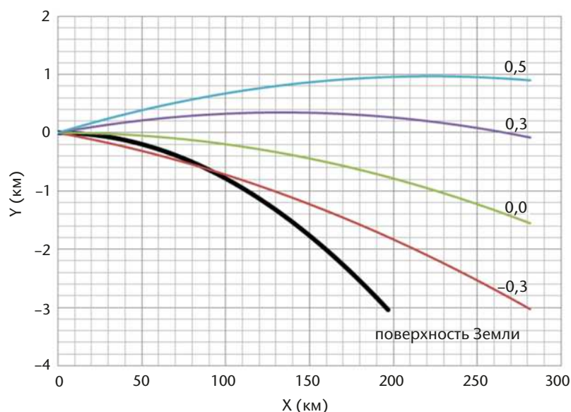
Рисунок 7.3. Схематическая диаграмма высоты луча для отдельных углов возвышения ( -0,3 ; 0 ; 0,3 и 0,5 ) над поверхностью Земли для стандартного индекса профиля рефракции в атмосфере, вычерченная в физическом пространстве с кривизной земной поверхности, эквивалентной радиусу Земли.
