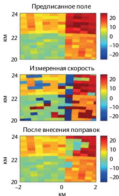
Рисунок 7.20. Метод двойной ЧПИ предполагает, что измерения производятся по объему с одинаковой радиальной скоростью. Изображения показывают предписанное поле, измеренные и скорректированные данные. (Рисунок адаптирован из работы Joe and May, 2003).
