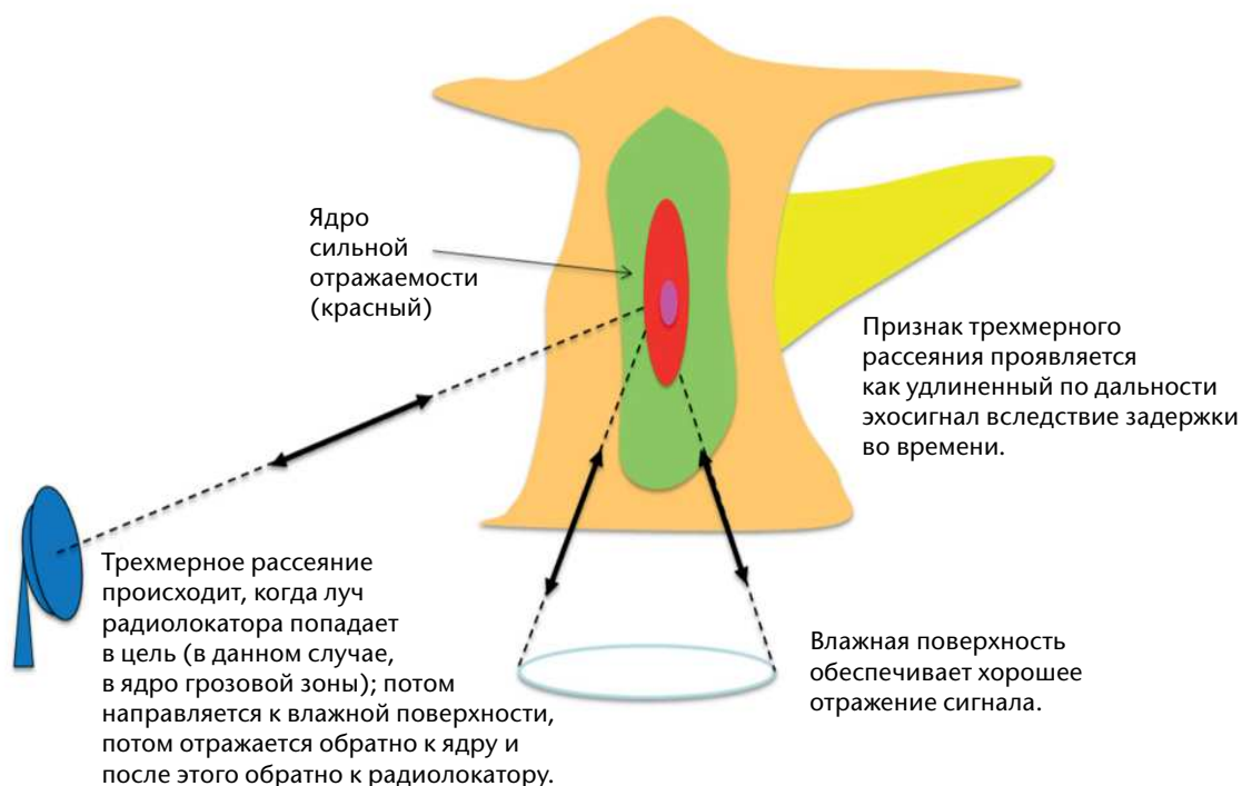
Рисунок 7.22. На этой схеме дается описание того, как происходит трёхмерное рассеяние. Эхосигнал, распространяющийся вправо (яркий желтый цвет), является артефактом, вызванным трехмерным рассеянием.
