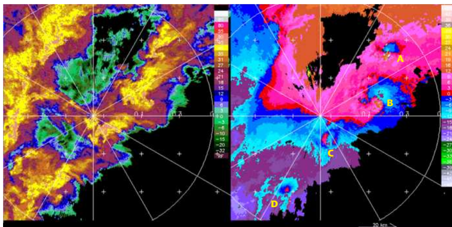
Рисунок 7.25. Многочисленные мезоциклоны (A-D) наблюдаются по линии шквалов и идентифицируются как пары относительных скоростей в обратном и прямом направлениях при постоянной дальности. Симметричные признаки скорости, наблюдаемые в ходе шторма, не являются очевидными или были исключены.
