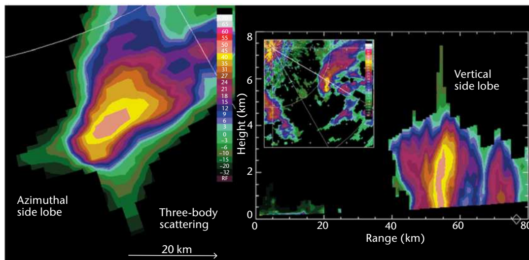
Рисунок 7.21. Эффекты боковых лепестков и множественного рассеяния приводят к появлению в некоторой степени похожих артефактов. Артефакты боковых лепестков наблюдаются на постоянной дальности, а множественное рассеяние — при постоянном азимуте.
