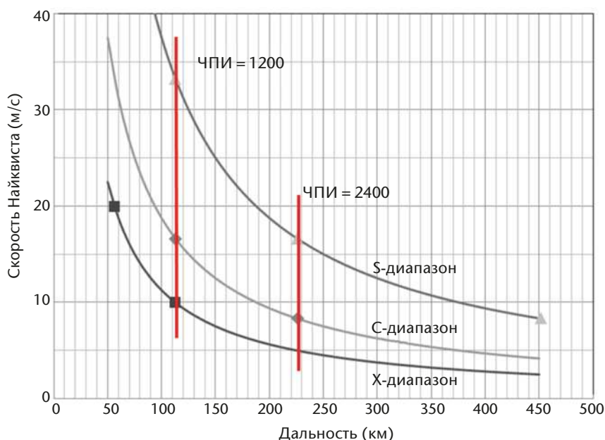
Рисунок 7.5. Это иллюстрация доплеровской дилеммы для трех частотных диапазонов обычных радиолокаторов (X, C, S). Эта дилемма возникает потому, что один из параметров, а именно частота повторения импульсов, т. е. время между излучаемыми импульсами, определяет максимальную однозначную скорость и максимальную однозначную дальность в противоположных направлениях. Маркеры и красные линии показывают общепринятые установочные параметры.
