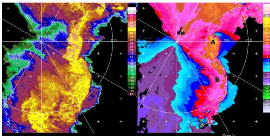
Рисунок 7.28. Другой признак весьма интенсивных опасных ветров может наблюдаться в качестве линейной или нелинейной характеристики в данных об отражаемости (слева) или радиальной скорости (справа).
