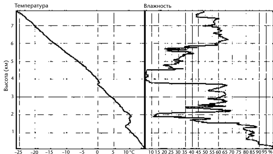
б) пример температуры и относительной влажности летом в 0600 UTC в Соединенном Королевстве (50° с. ш.), демонстрирующий неглубокий слой 100-процентной относительной влажности в тумане вблизи поверхности земли и очень резкое падение относительной влажности в слоях температурной инверсии между 1,5 и 2 км и на высоте 3,8 км.
