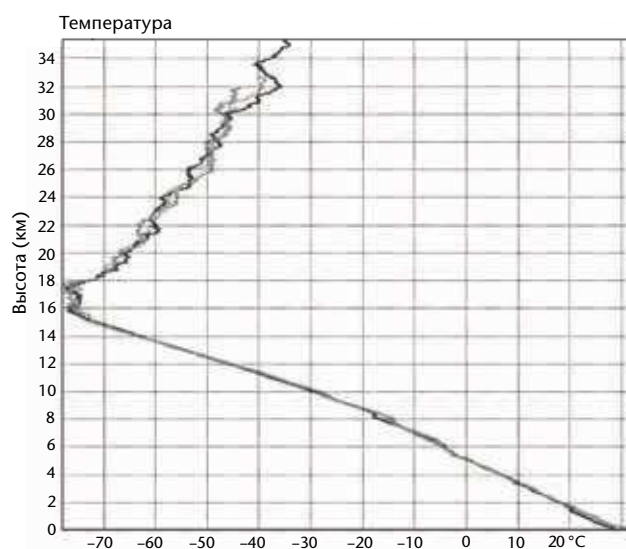
(а) июль, Янцзян, Китай (3 подъема за 8 ч)
