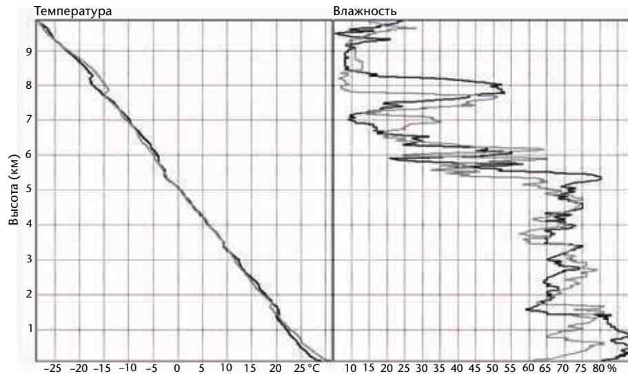
а) пример профилей дневной температуры и влажности, полученных в ходе взаимного сравнения высококачественных систем радиозондирования ВМО в Янцзяне, Китай (22° с. ш.). Зондирование, представленное серым цветом, было осуществлено через 8 часов после зондирования, которое изображено черным цветом. Относительно небольшие сдвиги в скорости изменения температуры по вертикали были связаны с быстрым падением относительной влажности (в районе 0,7, 1,6, 3,5, 5,5 и 8 км).
