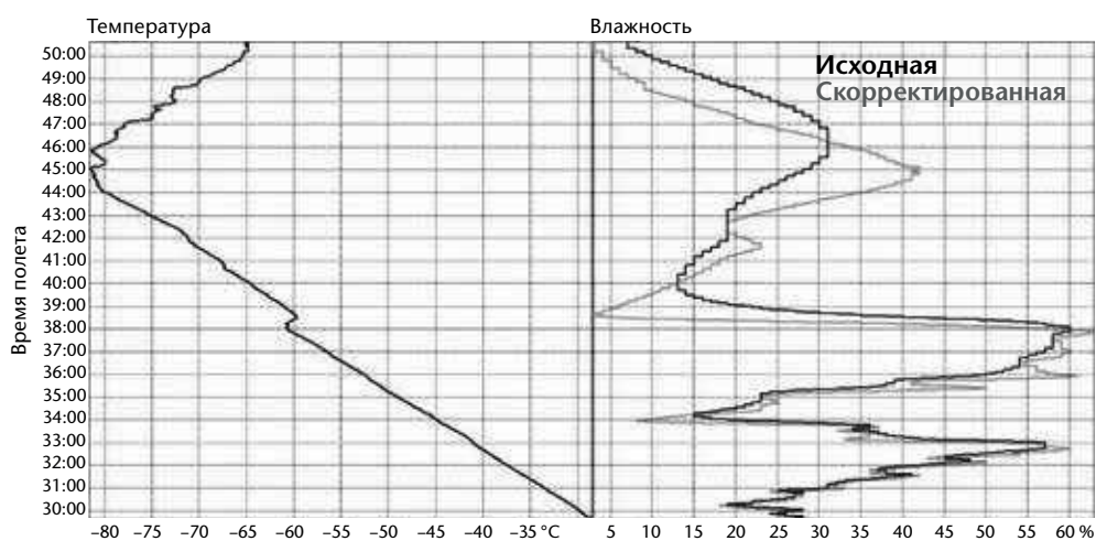
Рисунок 12.6. Измерения при помощи двойного тонкопленочного емкостного датчика в верхней тропосфере в ночное время в Янцзяне, Китай, представлены как функция времени от начала полета, при этом профиль влажности измерялся напрямую датчиком (черная кривая), а затем вносились поправки, учитывающие погрешности, обусловленные инерционностью датчика (серая кривая).
