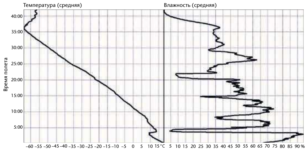
Рисунок 12.5. Средние значения параллельных измерений в первых интервалах двумя радиозондами, подвешенными вместе под одной оболочкой; измерения проводились в ночное время.
