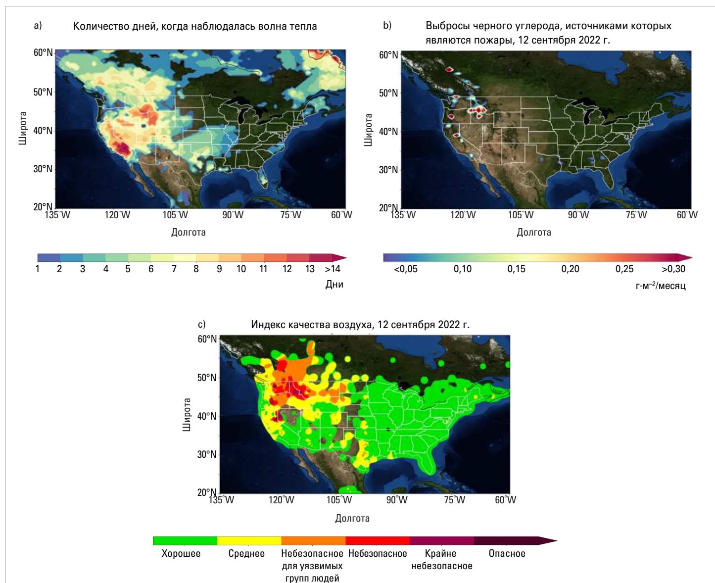
Рисунок 4. а) Реанализ атмосферных данных MERRA-2 NASA позволяет обнаружить высокую частоту волн тепла в западной части США в сентябре 2022 года. б) Волны тепла, наблюдаемые на северо-западе США, связаны с высоким уровнем выбросов в результате природных пожаров. в) Эти условия привели к загрязнению воздуха в большей части региона, о чем свидетельствуют данные, предоставленные AQIC США. Источник: Центр космических полетов НАСА им. Годдарда, Управление глобального моделирования и ассимиляции (УГМА); AQIC США
