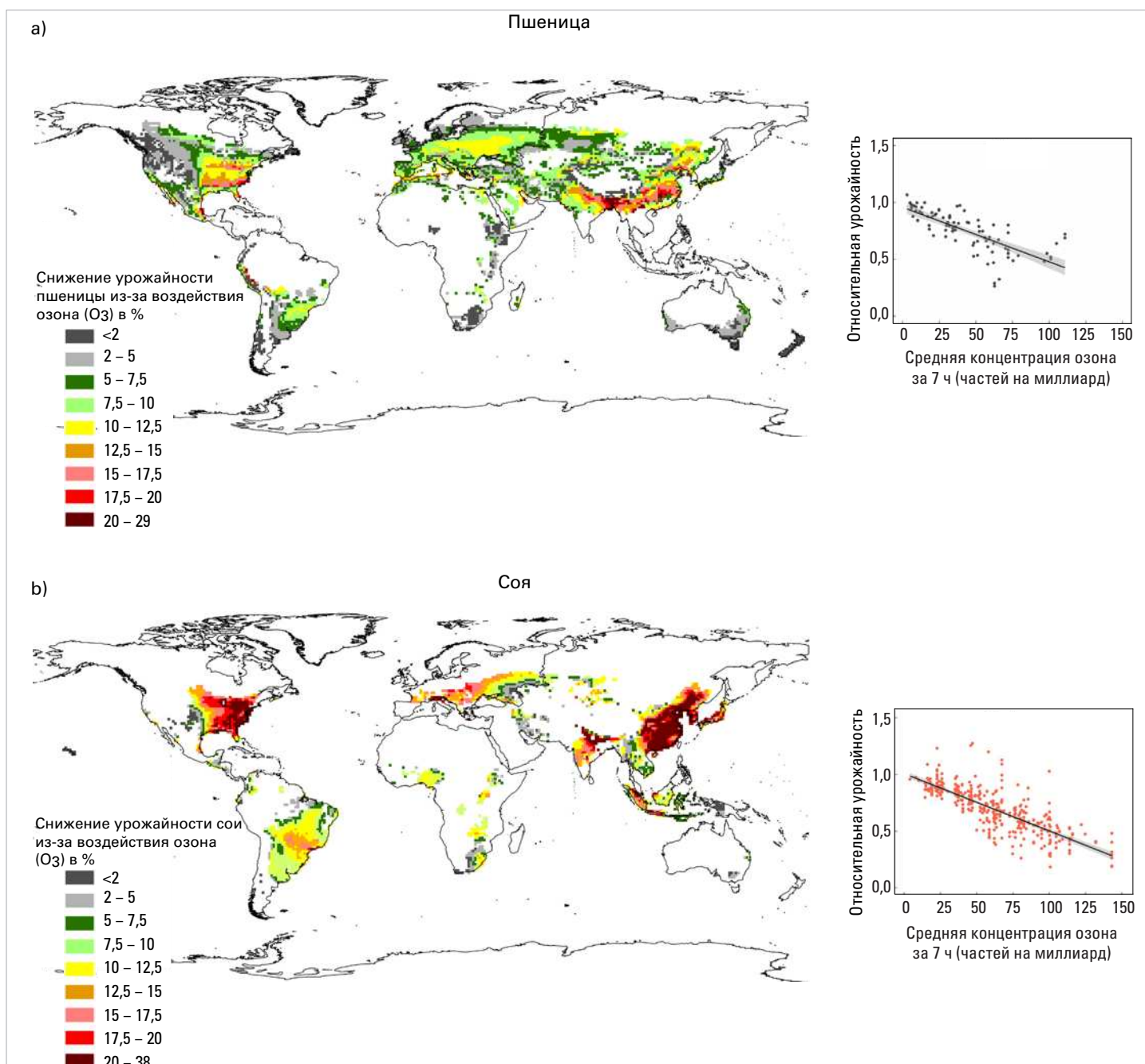
Рисунок 10. Снижение урожайности (в %) пшеницы (верхняя карта) и сои (нижняя карта) из-за воздействия озона в 2010–2012 годах. На диаграммах рассеяния показано снижение урожайности пшеницы (вверху) и сои (внизу) в зависимости от средней концентрации озона, измеряемой за 7-часовой период (в частях на миллиард, среднее значение за 90 дней, представляющее основной вегетационный период для каждой сельскохозяйственной культуры). Данные были объединены на основе результатов экспериментов с 18 сортами пшеницы и 52 сортами сои, проведенных в Азии, Северной Америке и Европе.
