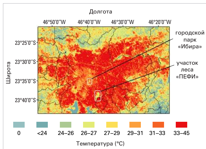
Рисунок 11. Приземная температура (°C) в столичном регионе Сан-Паулу 23 сентября 2015 года в 13:04 по местному времени Источник: Институт астрономии, геофизики и наук об атмосфере, Университет Сан-Паулу
