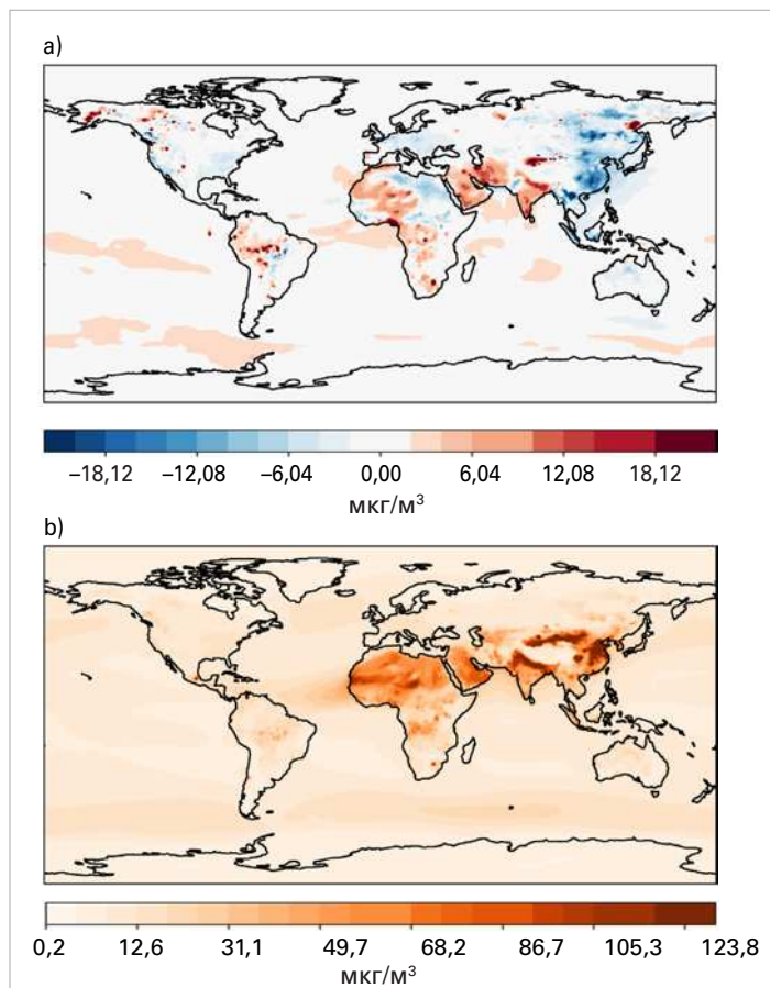
Рисунок 2. а) Аномалия (абсолютная разница) средних приземных концентраций \text{PM}_{2.5} ( \text{мкг}/\text{м}^3 ) в 2022 году по данным реанализа СМАК в сравнении с б) средним значением за 2003–2022 годы. Низкие концентрации \text{PM}_{2.5} в мировом океане в значительной степени обусловлены наличием частиц морской соли природного происхождения. В системе реанализа СМАК собраны данные об оптической плотности аэрозоля (ОПА), полученные со спутника с помощью спектро радиометра для получения изображений среднего разрешения (MODIS) и усовершенствованного радиометра с траекторным сканированием (AATSr). Кроме того, был использован набор данных о выбросах во время природных пожаров Глобальной системы ассимиляции данных о пожарах (ГСАДП).
