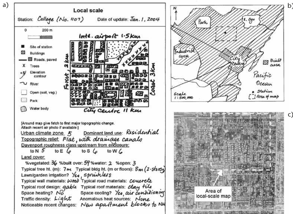
Рисунок 9.6. Минимальная информация, необходимая для описания локального (местного) масштаба окружающей среды городской станции, содержит а) шаблон для документирования местных условий; б) схематическую карту расположения станции в более крупной городской зоне и в) аэрофотоснимок.
