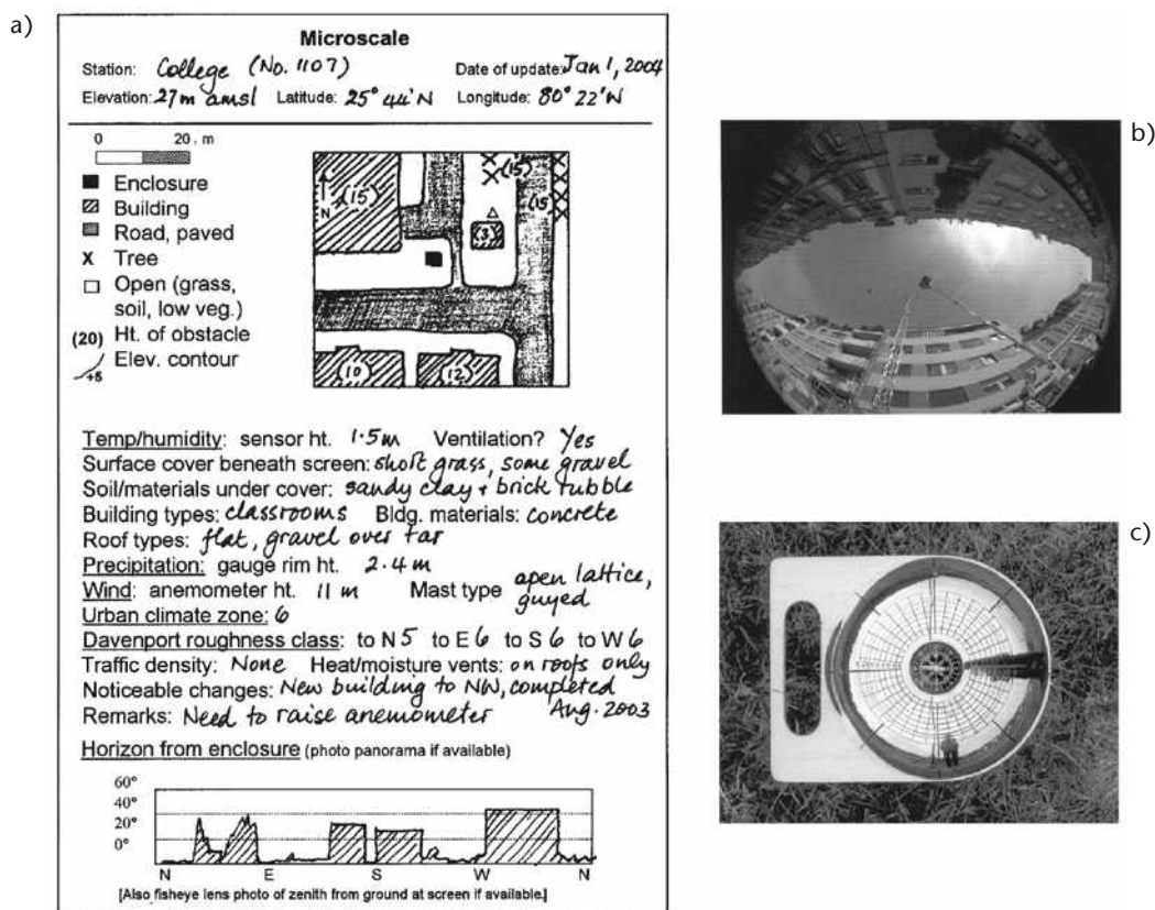
Рисунок 9.7. Информация, требуемая для описания микромасштаба окружения городской климатической станции; а) шаблон для файла метаданных; б) пример фотоснимка объективом типа «рыбий глаз» уличного каньона иллюстрирует закрытость горизонта и с) полусферический рефлектор Метеорологического бюро СК, расположенный на дождемере.
