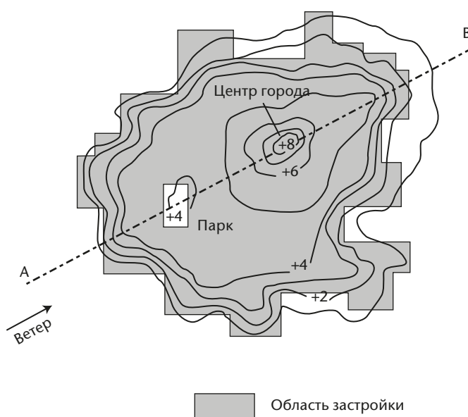
Рисунок 9.3. Типичная пространственная картина изотерм в большом городе ночью при безветренной ясной погоде, иллюстрирующая влияние эффекта «теплового острова» (Oke, 1982).
