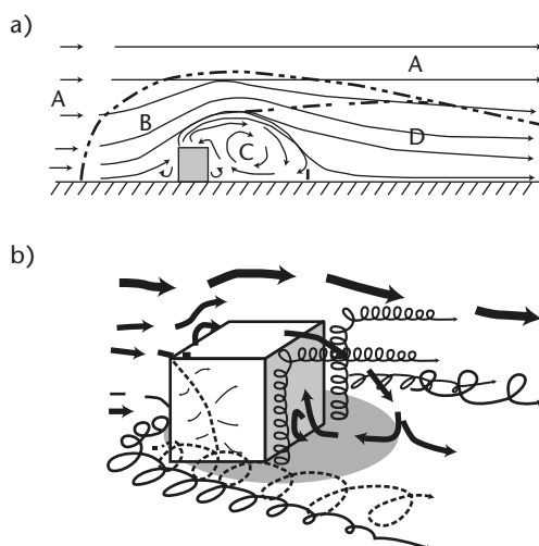
Рисунок 9.5. Типичный двумерный поток, огибающий здание, стоящее против набегающего потока (а): направления потока и его зоны; А представляет невозмущенный поток, В — возмущенный поток, С — впадину, D — след возмущенного потока (по Halitsky, 1963), и (b): поток и структуры вихрей (упрощение по Hunt et al., 1978).
