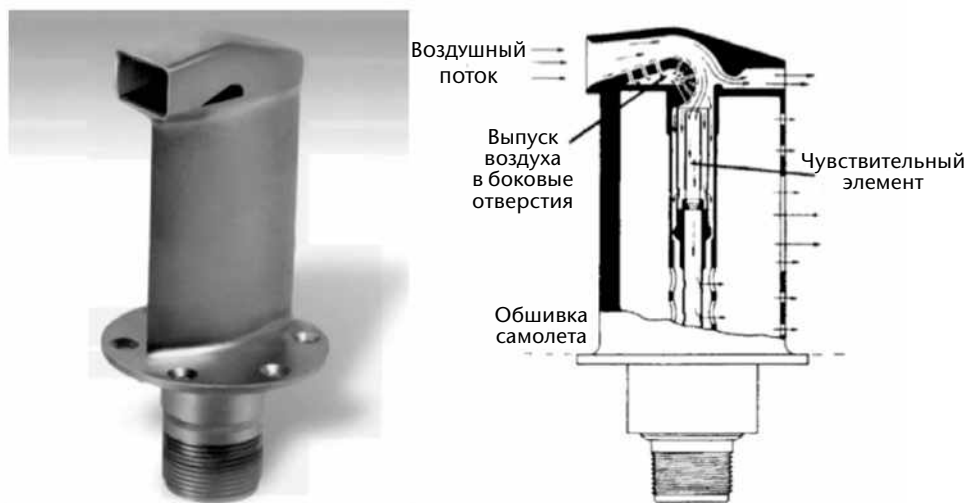
Рисунок 3.4. Типичный пример датчика температуры воздушного судна — датчика полной температуры воздуха (см. Stickney et al., 1990). Внутренняя аэродинамика проектируется таким образом, чтобы торможение потока происходило до момента соприкосновения с датчиком. Соответствующий внутренний пограничный слой сохраняется достаточно малым и, вместе с тем, в стороне от сенсорного элемента, с тем чтобы торможение воздушного потока постоянно происходило в виде чисто адиабатического процесса. Искривление потока используется для сепарации частиц.
