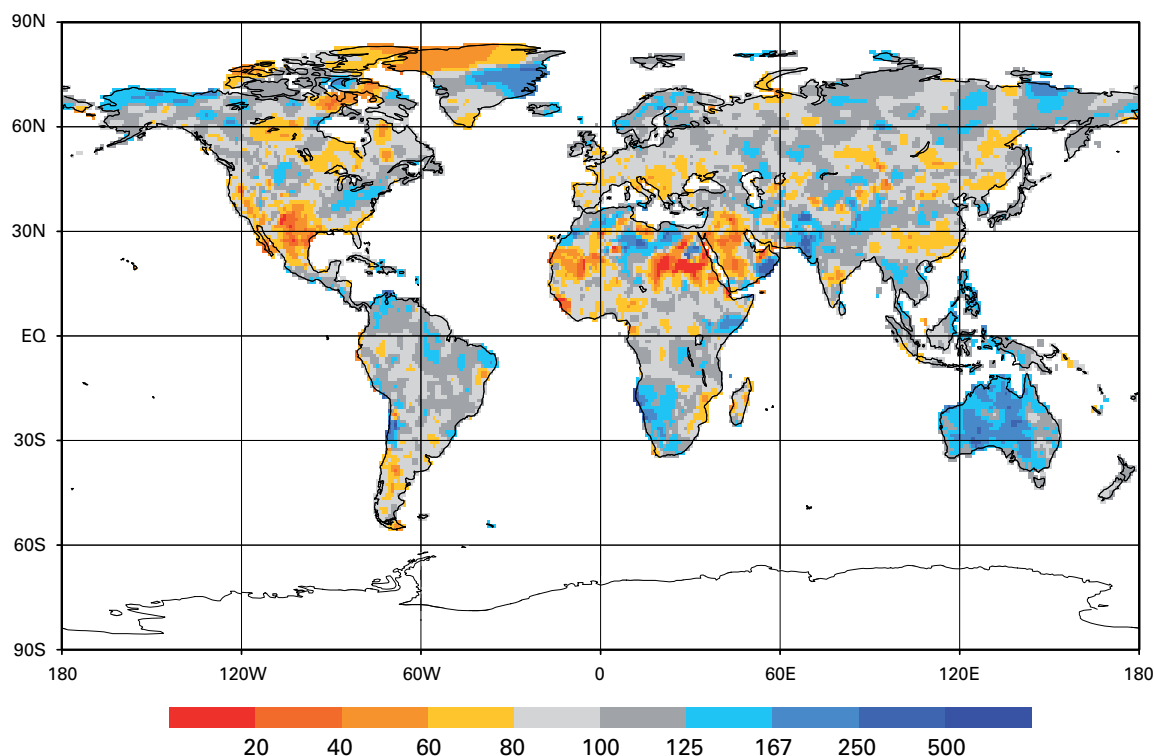
Рисунок 6. Аномалии годовых атмосферных осадков для районов суши в глобальном масштабе за 2011 год; анализ распределения измеренных дождемерами осадков по данным в узлах сетки с шагом в 1° в виде процентной доли от среднего значения с ориентацией на базовый период 1951–2000 гг.
