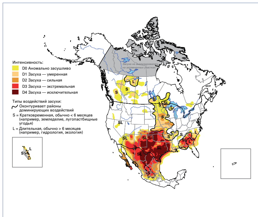
Рисунок 11. Засуха в Северной Америке по состоянию на конец октября 2011 г.
