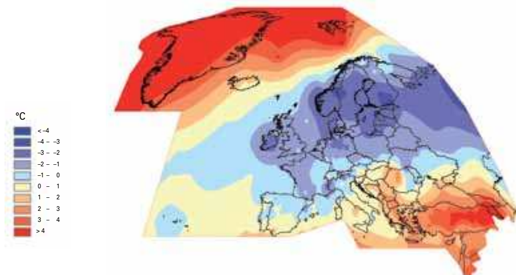
Рисунок 6. Месячные аномалии температуры (°C) на территории Европы относительно базового периода 1961–1990 гг. для декабря 2009 г. – февраля 2010 г. (слева) и для декабря 2010 г. (справа) (Источник: Региональный климатический центр Региональной ассоциации VI (Европа) ВМО по мониторингу климата, Метеорологическая служба Германии)
