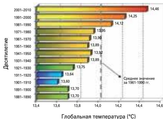
Рисунок 3. Десятилетняя глобальная средняя совокупная температура над поверхностью суши — поверхности океана (°C) на основе трех глобальных комплектов данных по температуре (Источник: Центр Гадлея Метеобюро СК и Отдел исследований климата Университета Восточной Англии, Соединенное Королевство)
