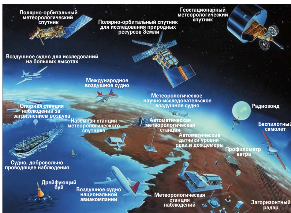
Рисунок 2.1. Иллюстрация некоторых из многочисленных систем наблюдений, используемых на поверхности суши, в море, атмосфере и космосе для мониторинга и исследования климатической системы
