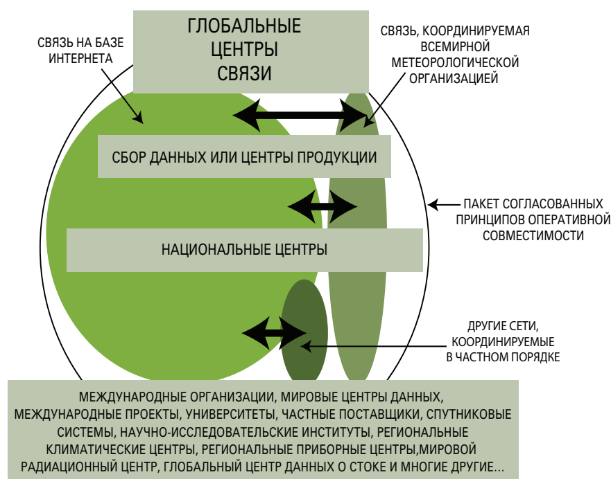
Рисунок 2.8. Схематическая иллюстрация возможной Информационной системы климатического обслуживания, которая включает Информационную систему Всемирной Метеорологической Организации и другие сети на базе Интернета и частные сети, работающие в рамках пакета функциональной совместимости.
