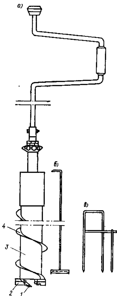
Рис. 18.1. Керноотборник.
