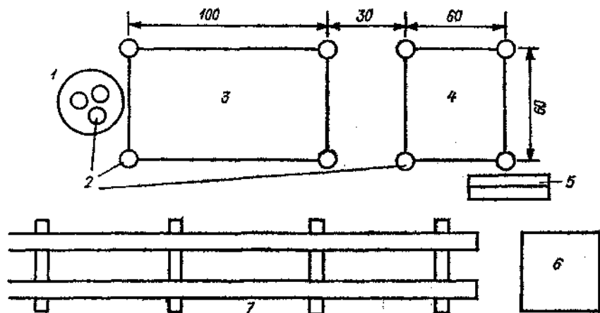
Рис. 23.2. Схема размещения фильтрационного оборудования на площадке.
