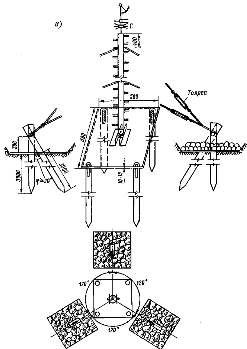
Рис. 19.1. Установка и крепление металлической (а) и деревянной (б) мачт а) Диаметр мачты и
