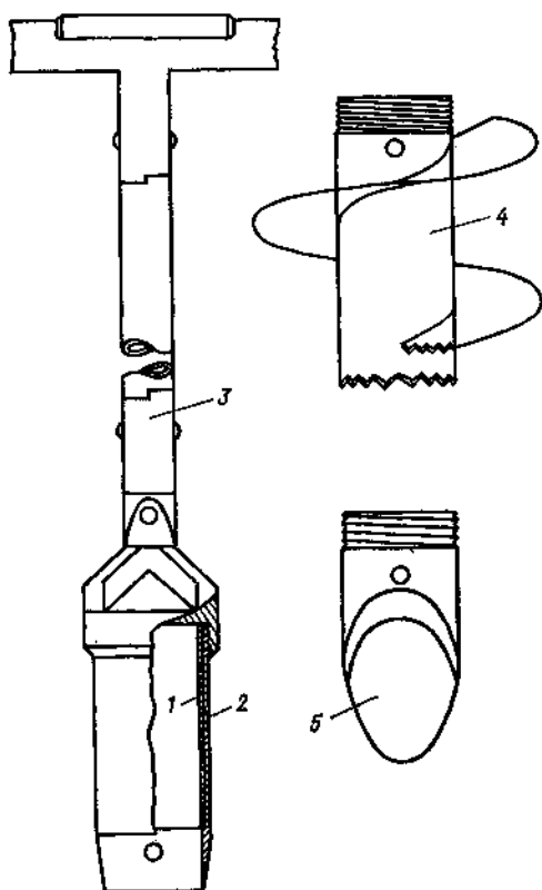
Рис. 14.1. Пробоотборник со сменными резцами.
