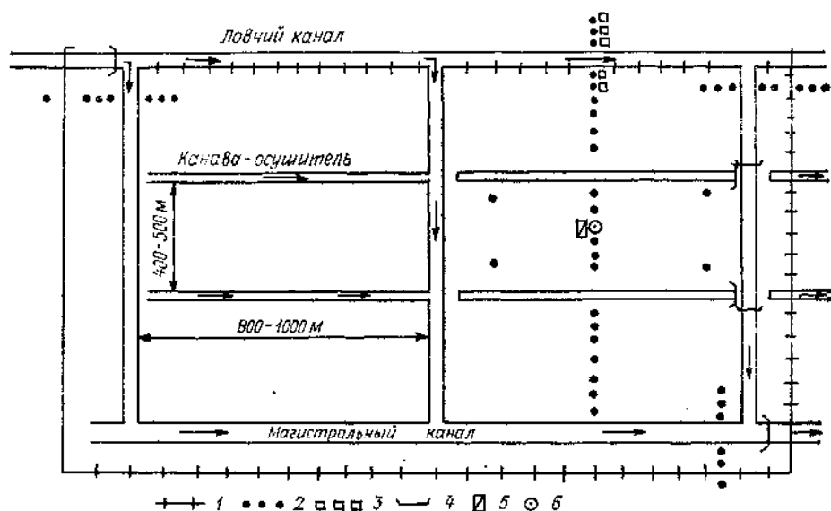
Рис. 7.2. Схема размещения наблюдательных пунктов на осушенном болоте, используемом под лесные угодья. Усл. обозначения как на рис. 7.1.
