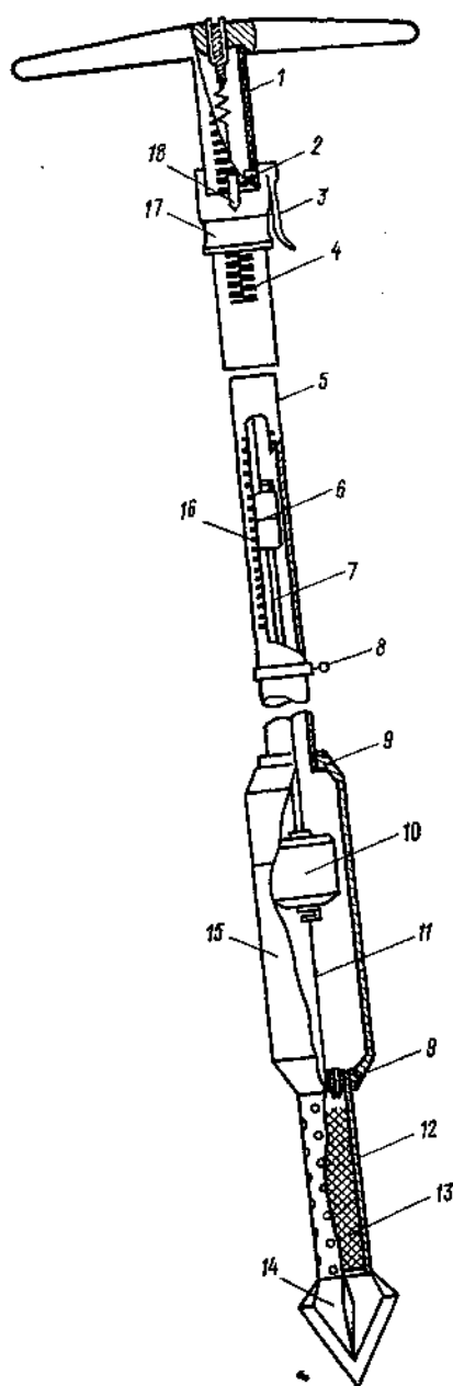
Рис. 5.3. Устройство таксационной опоры-пьезометра.
