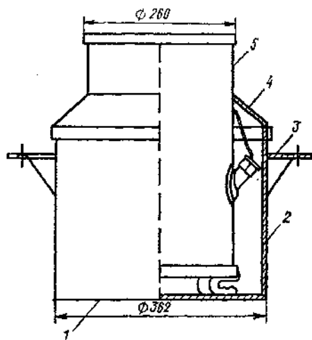
Рис. 11.2. Модернизированный почвенный дождемер.
