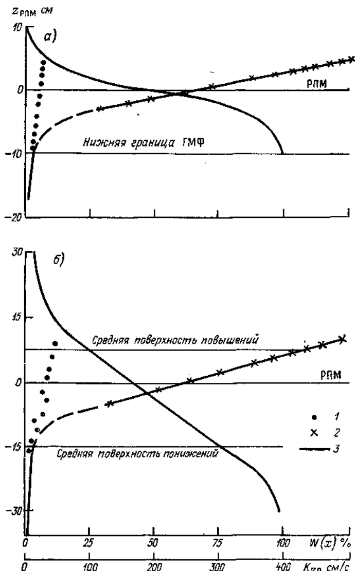
Рис. 23.4. Совмещение кривых K_{z_{cp}} = f(z) (1), K_{z_n} = f(z) (2) и W(x) (3) для мохово-травяных (а) и лесных и облесенных (б) микроландшафтов.
