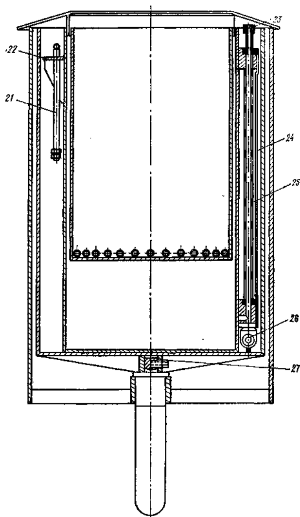
испаритель ГГИ-Б-1000М.
