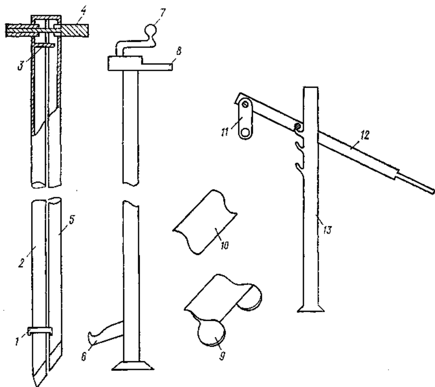
Рис. 15.3. Комплект пробоотборника Метса Л. Я.
