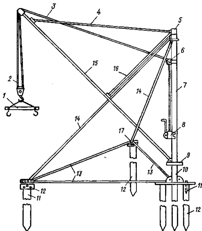
Подъемное устройство ГР-22.
