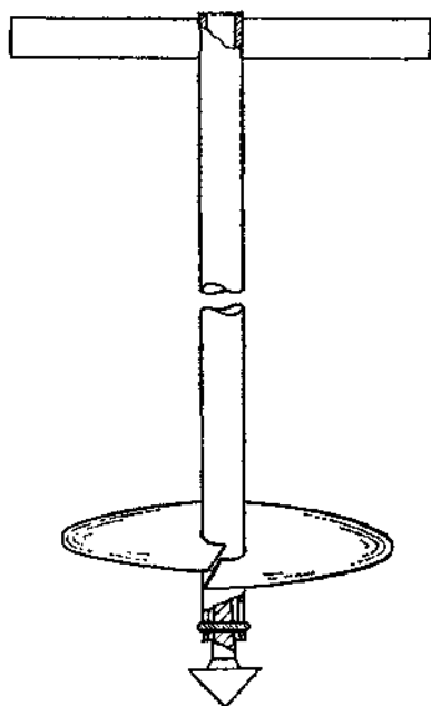
Рис. 11.5. Тарелочный торфяной бур.
