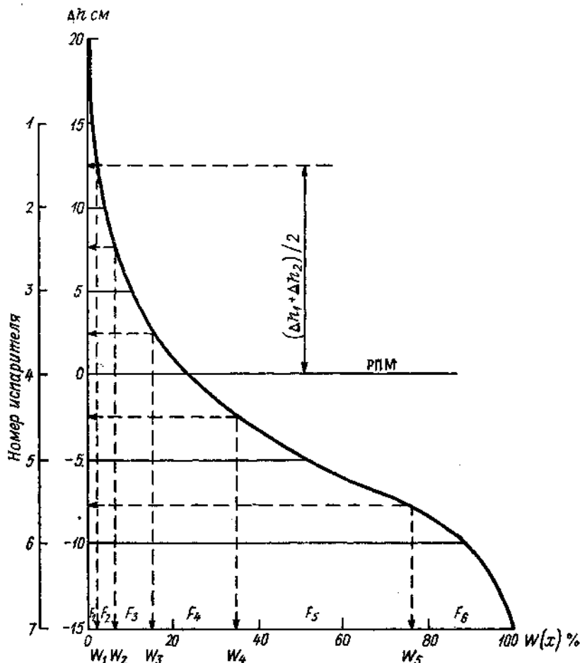
Рис. 11.3. Интегральная кривая распределения высот микрорельефа.
