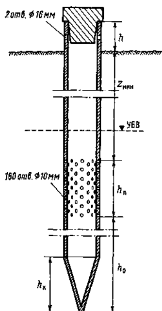
Рис. 21.1. Схематичное изображение скважины-трубы для отбора проб болотных вод на химический анализ.
