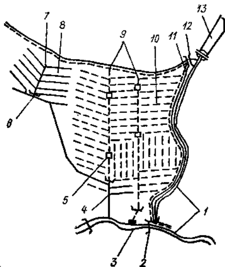
Рис. 7.3. Схема самотечной осушительной системы.
