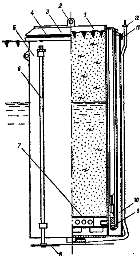
Рис. 11.6. Универсальный болотный испаритель (общий вид).
