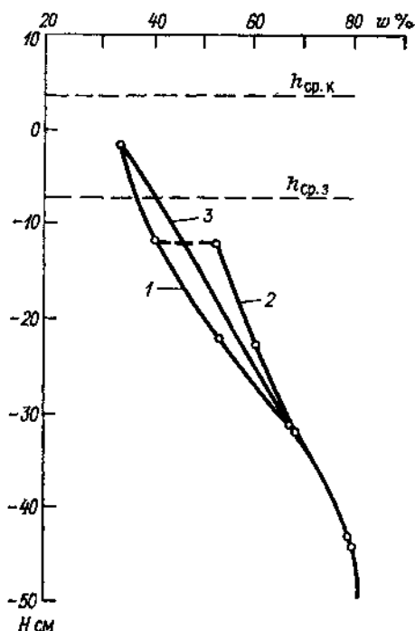
Рис. 15.4. Профили влажности в зоне аэрации торфяной залежи на участке № 3, 17.08.85 г., z_{\text{РПБ}} = -63 см.
