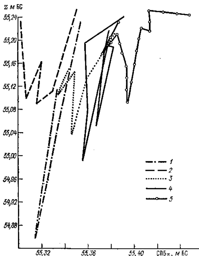
Рис. 6.1. Зависимость высотной отметки СПБ z от уровня болотных вод z .
