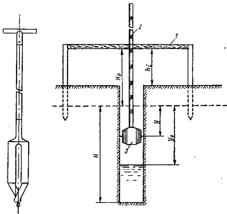
Рис. 23.5. Бур Розанова.
