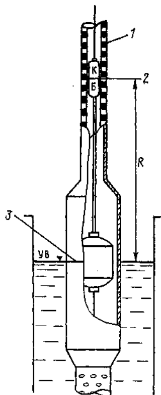
Рис. 5.4. Схема контроля расстояния R .
