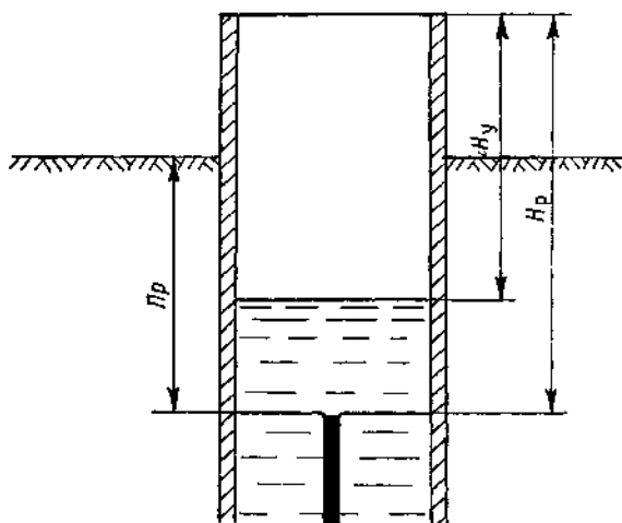
Рис. 12.3. Схема определения приводки нуля водомерной скважины.
