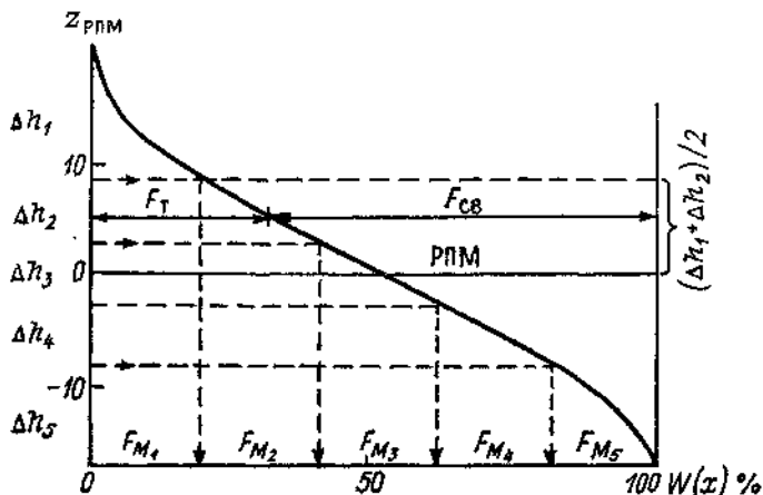
Рис. 26.2. Определение значений F_M , F_T , F_{св} по интегральной кривой распределения высот микрорельефа.
