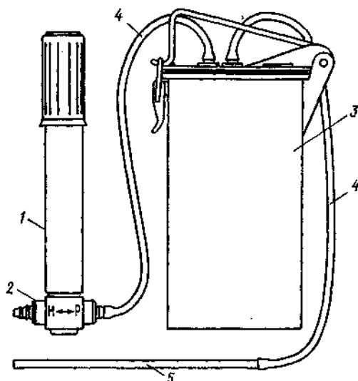
Рис. 11.7. Полевой вакуумный насос с промежуточной емкостью.
