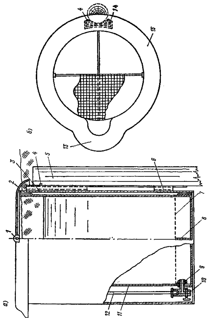
Рис. 11.4. Весовой испаритель ГГИ-Б-1000 (а) и его вид сверху (б).
