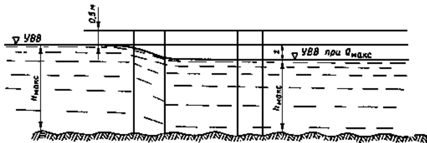
Рис.1. Схема к расчету степени сужения потока
