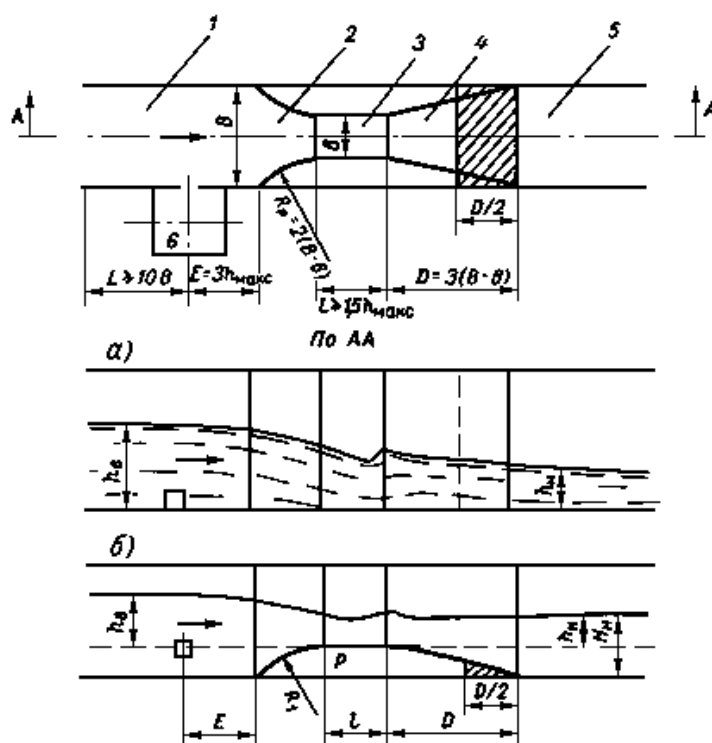
Рис.VII.3. Лоток Вентури
