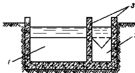
Рис. I.1. Комбинированный тонкостенный водослив для учета малых и больших расходов воды 1 - водослив большой; 2 - водослив малый; 3 - несущая конструкция
