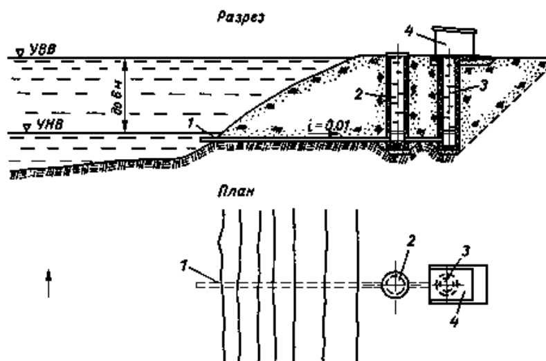
Рис. III.10. Нормальная компоновка установки СУВ берегового типа с промежуточным незатопляемым поплавковым колодцем
