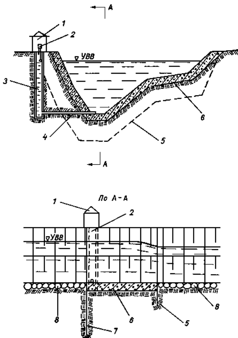
Рис.VI.4. Контрольное русло со сплошным бетонным креплением смоченного периметра 1 - измерительный павильон; 2 - СУВ; 3 - поплавковый колодец; 4 - соединительное устройство (труба); 5 - граница низового шпунтового ряда; 6 - бетонное покрытие; 7 - верховой шпунтовый ряд (применяется в случае водопроницаемых грунтов в русле); 8 - каменная одиночная мостовая
