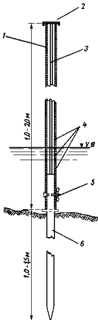
Рис.III.16. Максимальная рейка в металлической трубе
