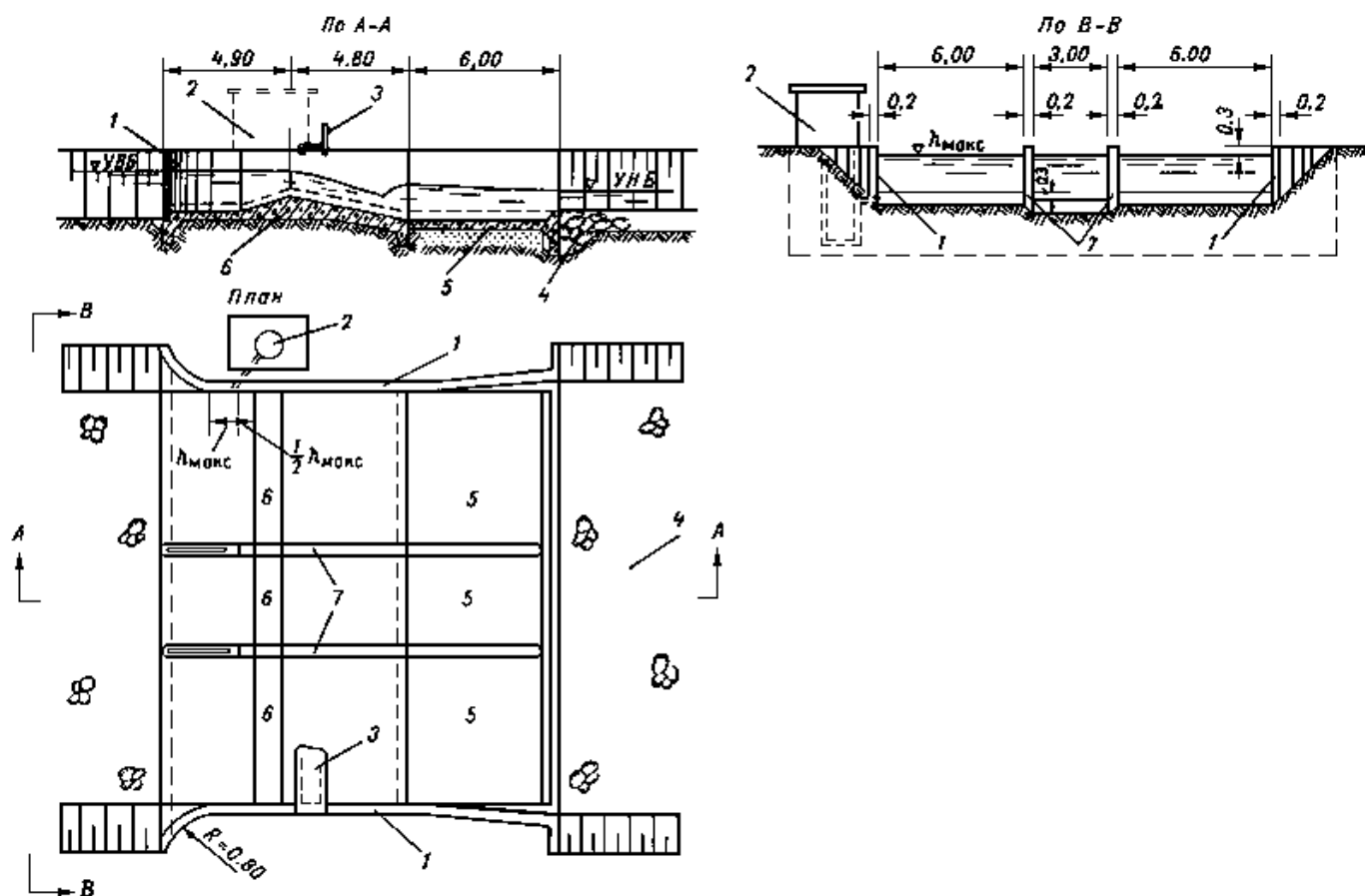
Рис.VIII.2. Водослив с треугольным профилем порога для измерения расхода до 50 м³/с
