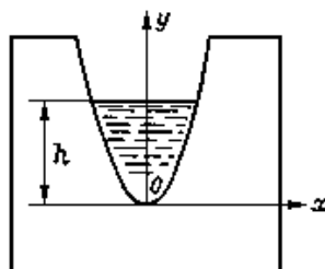
Рис.IX.8. Параболический водослив
