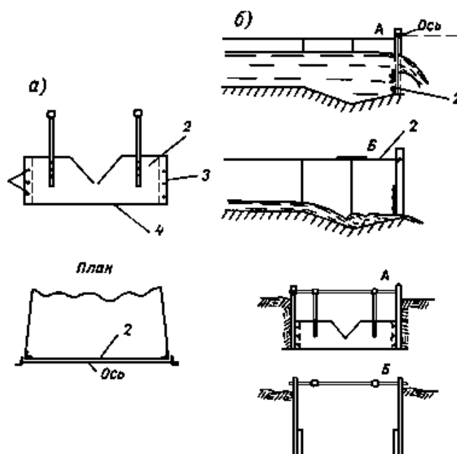
Рис.XI.3. Способы установки временной водосливной рамки для тарирования гидрометрического лотка
