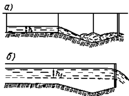
Рис.XI.2. Схема установки временной водосливной рамки для тарирования гидрометрического лотка
