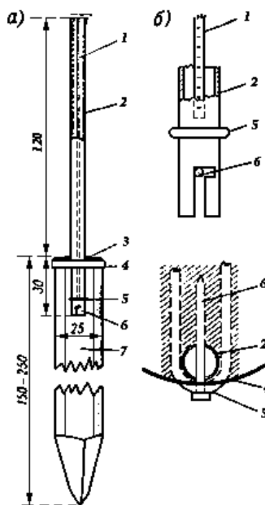
Рис.III.17. Водомерный пост с максимальной рейкой
