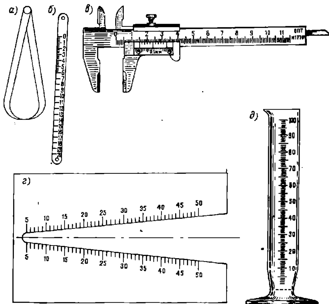
Рис. 19. Инструменты для измерения отложения.
