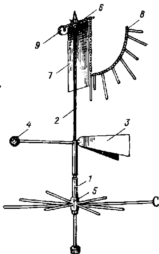
Рис. 15. Флюгер.
