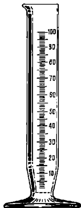
Рис. 4. Измерительный стакан осадкомера.
