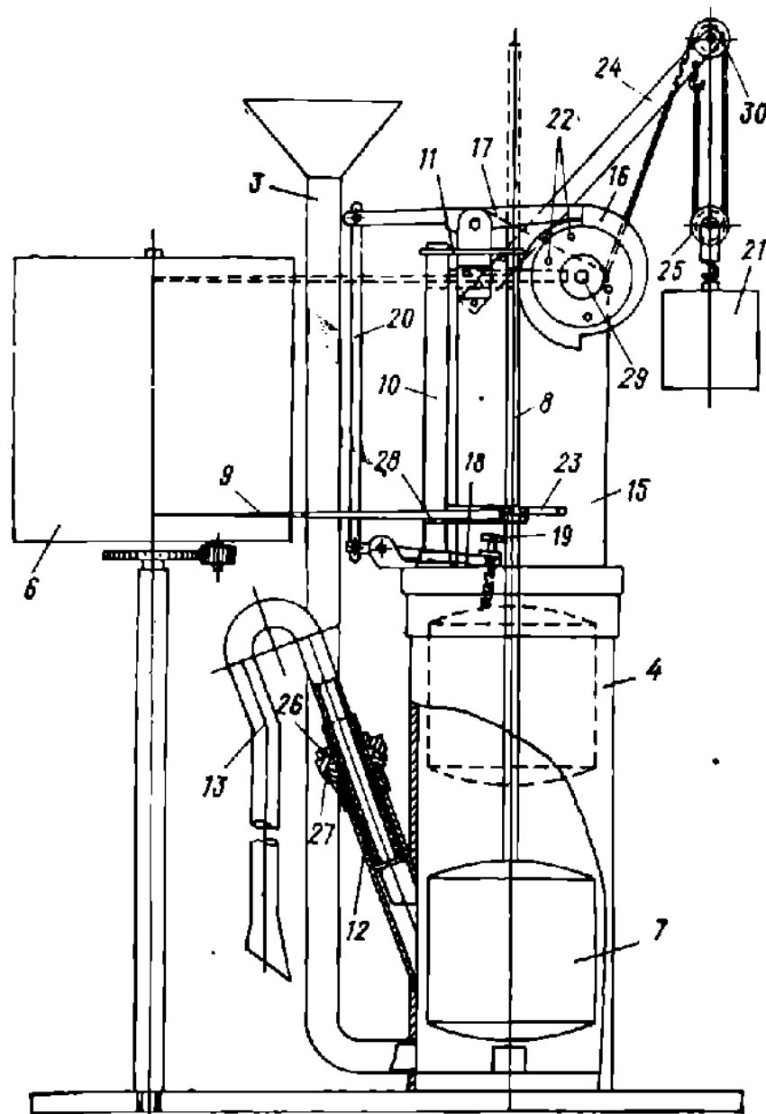
Рис. 6. Устройство механизма принудительного слива pluviографа.
