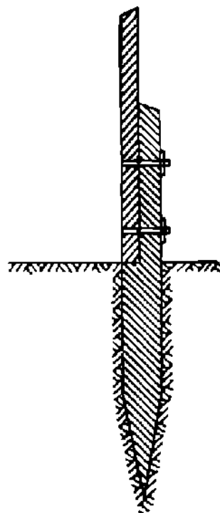
Рис. 4.1. Крепление стационарной снегомерной рейки
