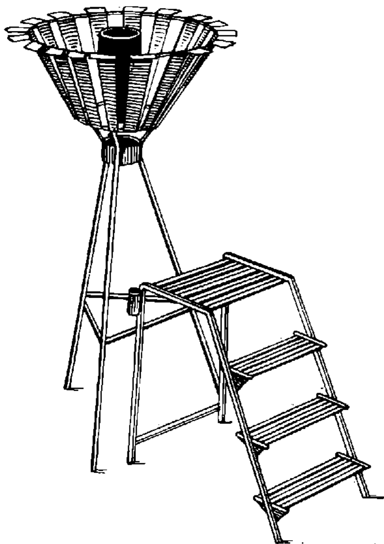
Рис. 1. Осадкомер О-1.
