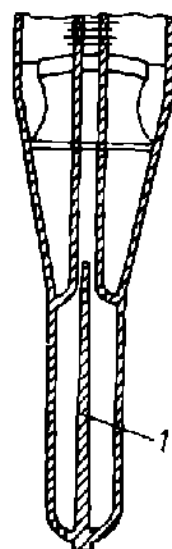
Рис. 12. Разрез резервуара максимального термометра.
