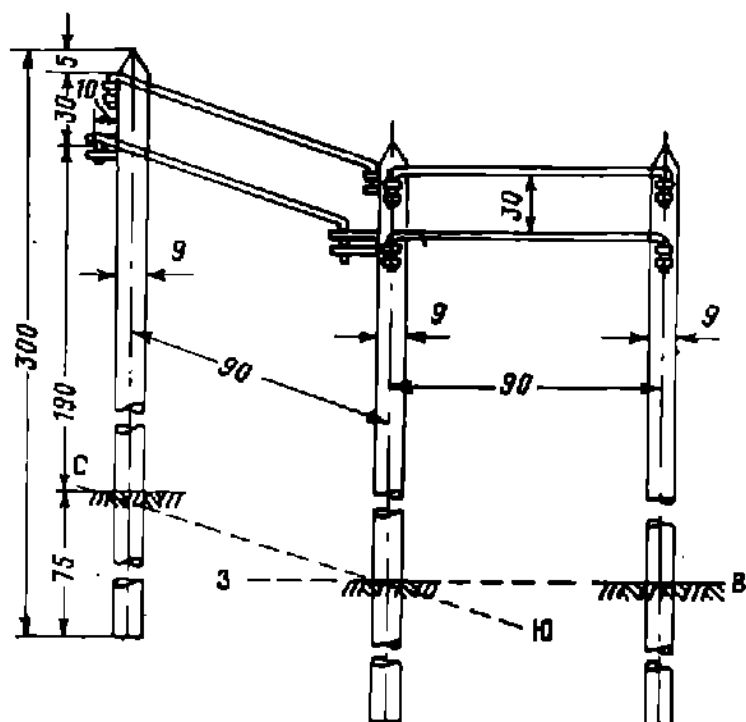
Рис. 16. Чертеж гололедного станка (размеры указаны в сантиметрах).
