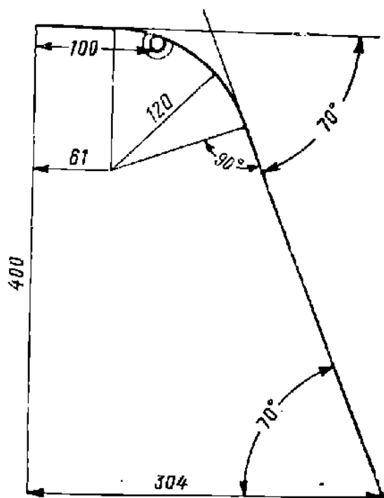
Рис. 3. Шаблон для проверки изгиба планок защиты осадкомера.
