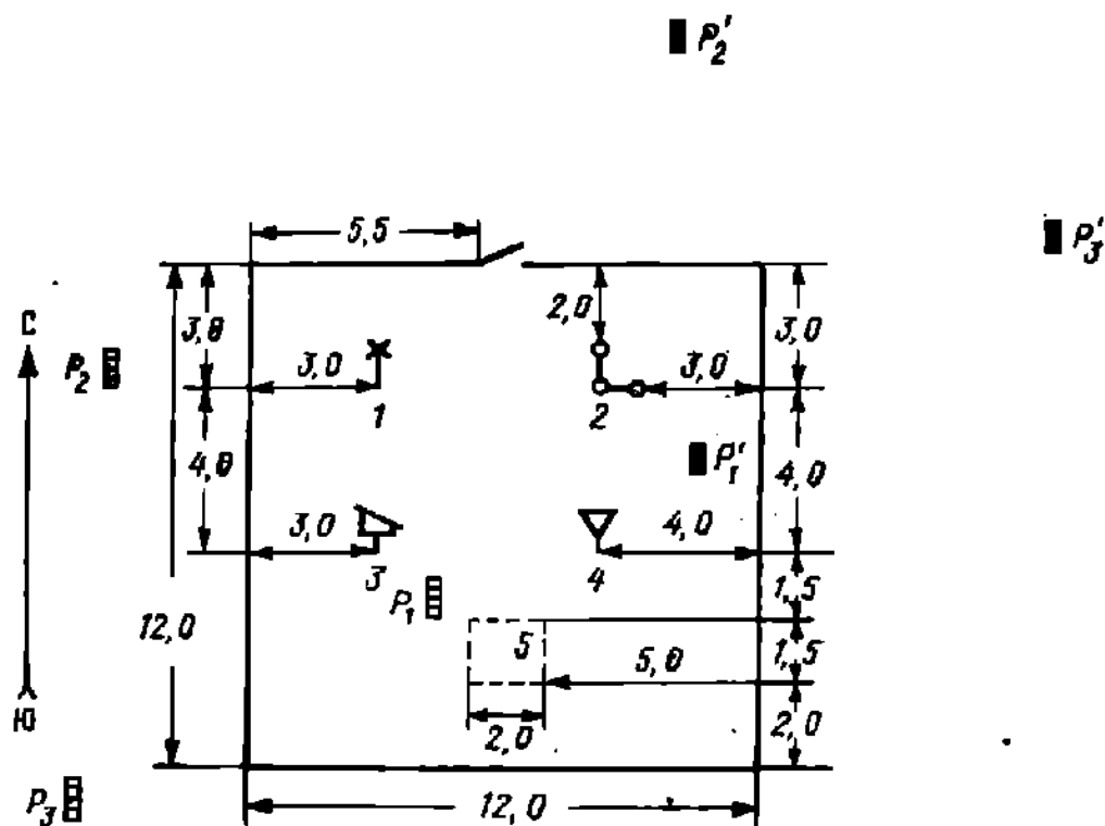
Рис. 1.1. Схематический план размещения приборов и установок на гидрометеорологическом посту с полным объемом наблюдений.
