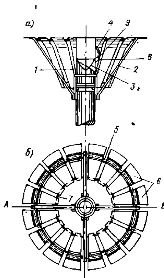
Рис. 2. Разрез осадкомера О-1.
