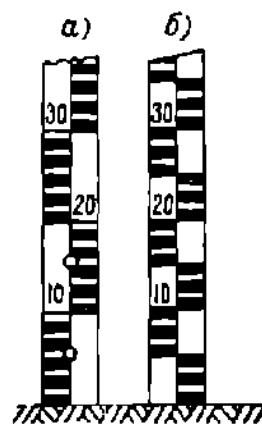
Рис. 7. Рейки снегомерные стационарные.
