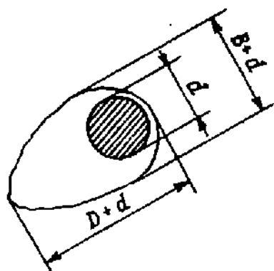
Рис. 6.3. Схема измерений диаметра и толщины отложения.
