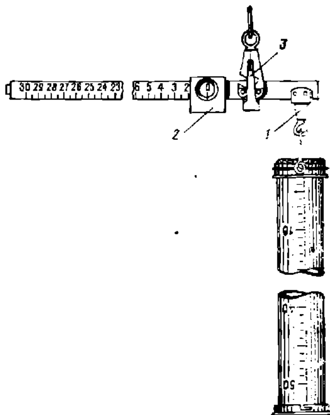
Рис. 9. Снегомер весовой.
