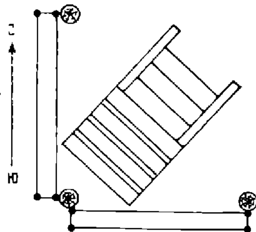
Рис. 17. Схема установки гололедного станка относительно стран света.
