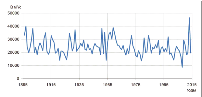
Рисунок Б.1 – Хронологический ход значений максимальных расходов воды, м³/с, по г/ст. р. Амур – г. Хабаровск за период с 1896 по 2014 год
