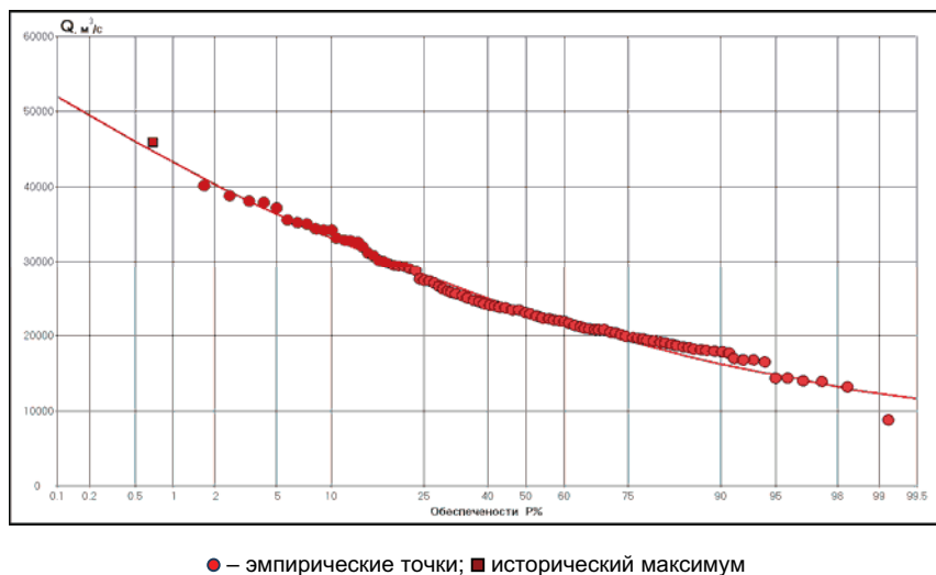
Рисунок Б.2– Эмпирическая и аналитическая кривые распределения максимальных расходов воды, м³/с, по г/ст. р. Амур – г. Хабаровск с учетом исторического максимума
