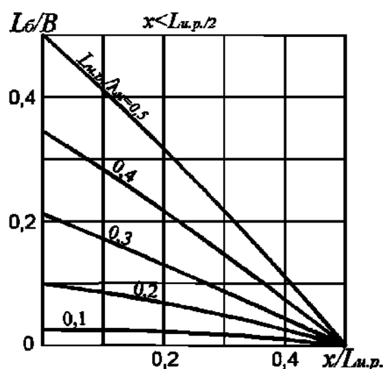
Рисунок 10.4 — Графики относительного размыва выпуклого берега в зависимости от расстояния проектного створа до вершины излучины при различных темпах смещения излучины
