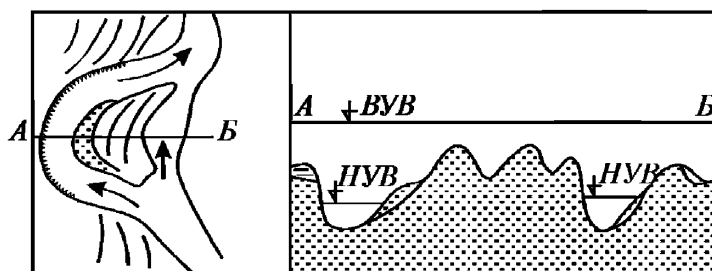
Рисунок 5.3 — Типичный план и поперечный разрез поймы при незавершенном меандрировании — крупно-грависто-песчаная пойма
