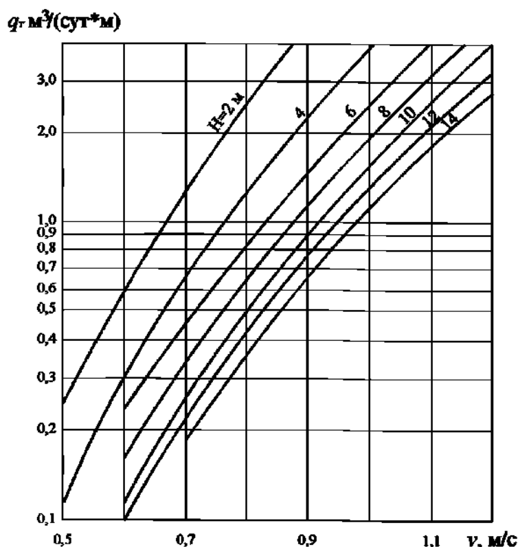
Рисунок 9.3 — Номограмма для расчета q_T по формуле q_T = 18 \frac{V^3}{H}
