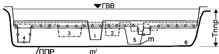
Рисунок 11.3 — Прогнозируемый поперечный профиль размыва русла (6) на участках рек с пойменной многорукавностью.
