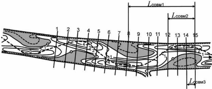
Рисунок 9.5 — Участок русла с побочным типом руслового процесса
