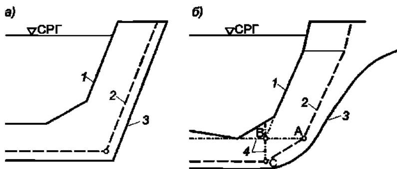
а) — при трассировке трубопровода с кривой искусственного гнутья, б) — при трассировке трубопровода по радиусу упругого изгиба; 1 — линия естественного дна, 2 — линия прогнозируемого размыва русла, 3 — дно траншеи, 4 — вспомогательные кривые построения прогнозируемого ППР.
