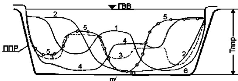
Рисунок 11.2 — Прогнозируемый поперечный профиль размыва русла (6) на участках рек с ленточно-рядовым и осередковым типами руслового процесса
