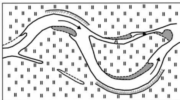
Рисунок 8.3 — Незавершенное меандрирование
