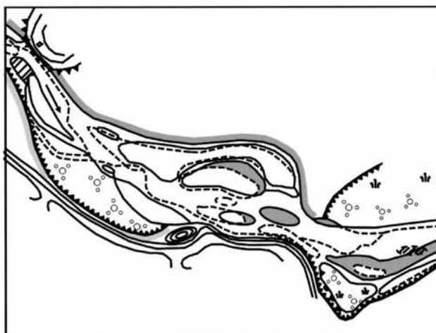
Рисунок 8.5 — Русловая многоруканность
