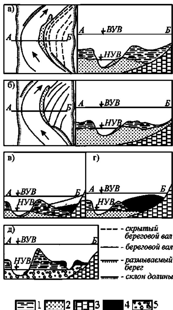
Рисунок 5.5 — Типичные поперечные разрезы пойм ограниченно меандрирующей реки
