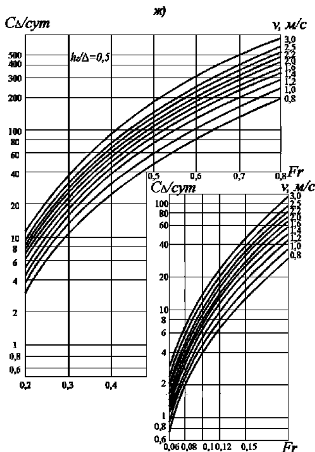
Рисунок 9.4 — Номограммы для определения скорости движения русловых мезоформ с учетом различных значений относительных высот микроформ h_0/\Delta :
