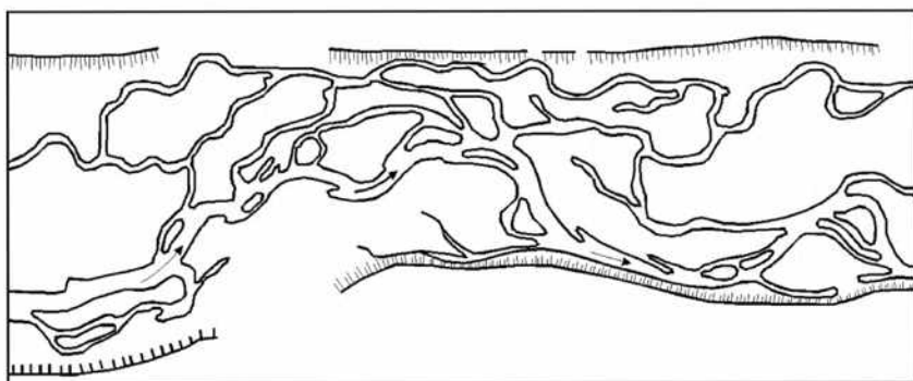
Рисунок 8.4 — Пойменная многоруканность
