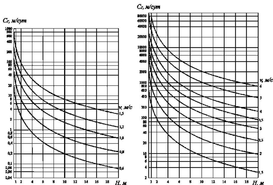
Рисунок 9.2 — Номограммы для определения скорости движения русловых микроформ
