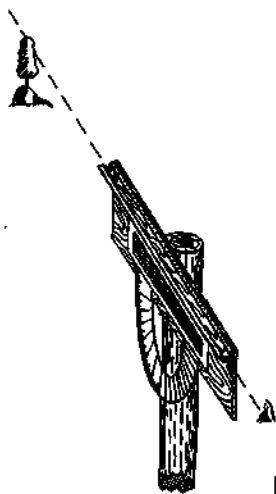
Рисунок А.3 – Упрощённый эклиметр
