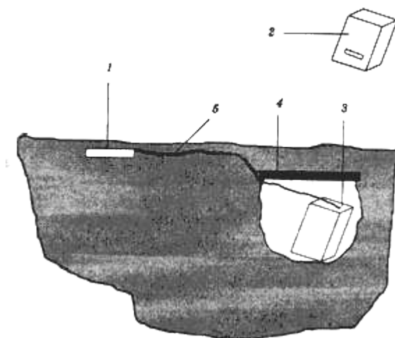
1 - датчик температуры; 2 - ПСИ; 3 - БИР; 4 - крышка; 5 - соединительный жгут
