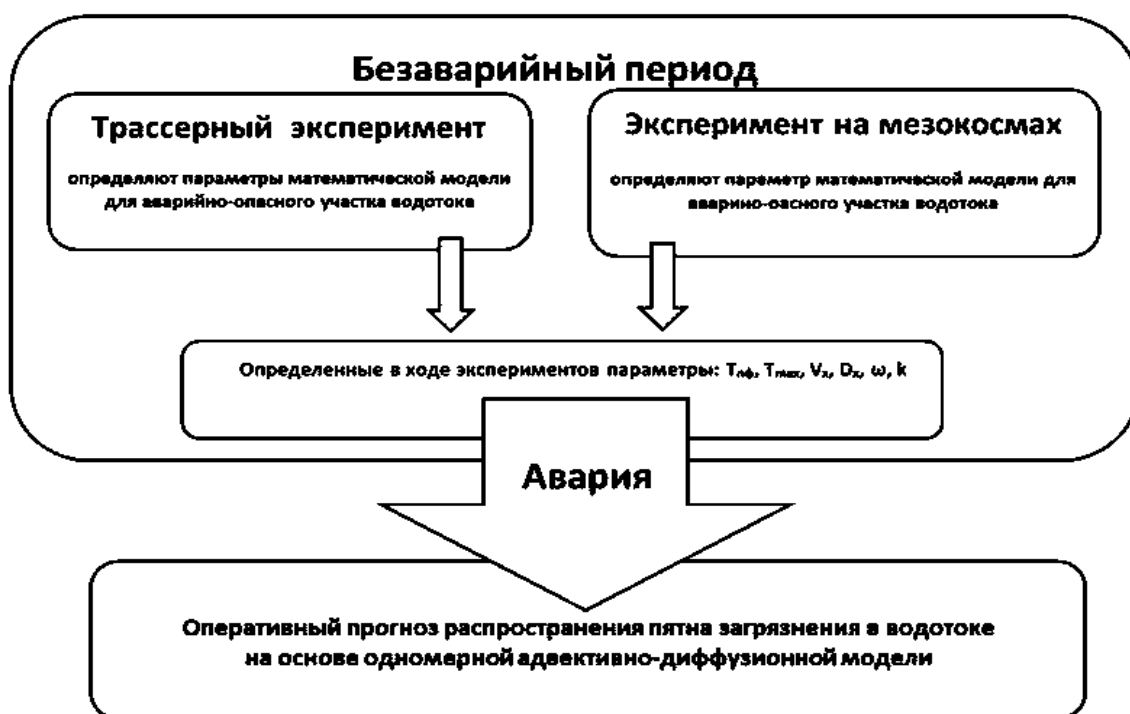
Рисунок 1 – Общая схема оперативного мониторинга аварийного загрязнения водотока
