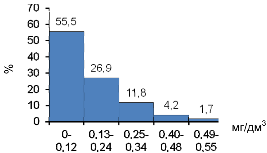
Рисунок А.1 – Гистограммы частотей концентраций азота аммонийного в воде р. Дон (г. Константиновск)
