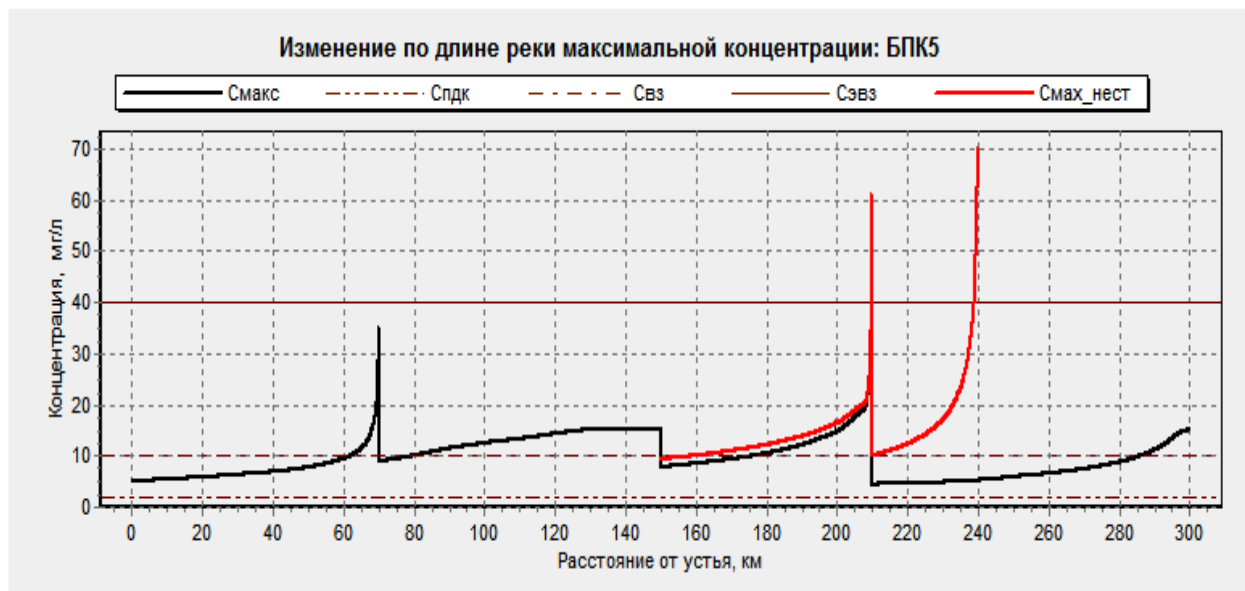
Рисунок А.18 – Иллюстрации результата расчета влияния нестационарного поступления ЗВ со склоновым стоком
