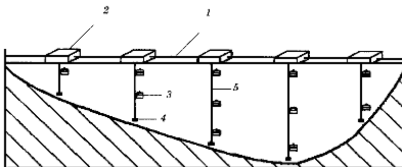
1 - капроновый трос; 2 - пенопластовый плотик; 3 - емкость (бутылка) для отбора проб; 4 - груз; 5 - вертикальный шнур
