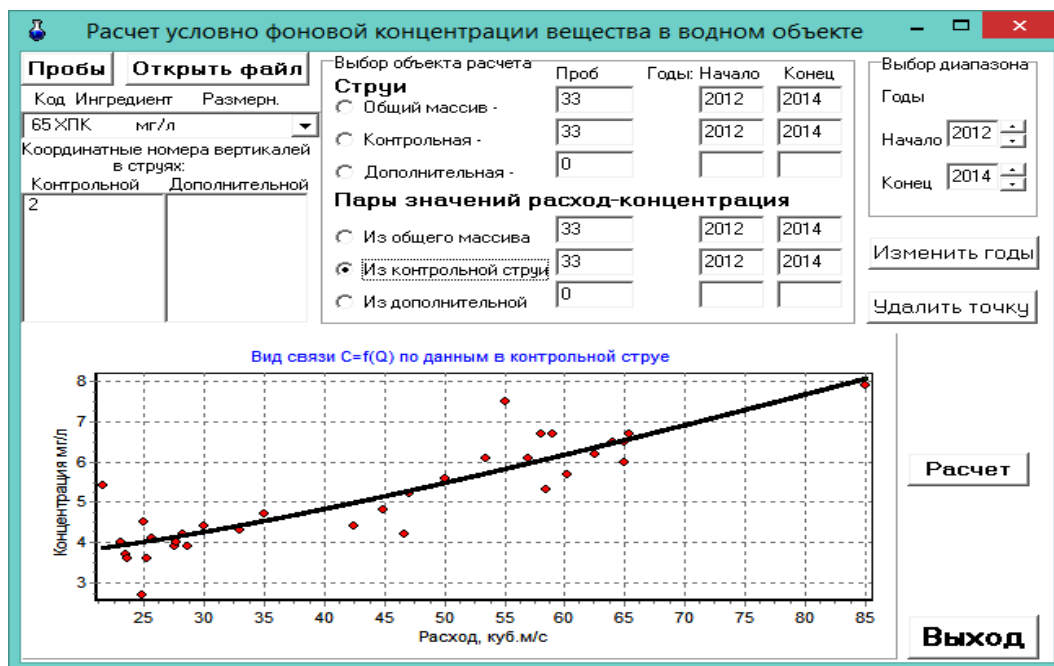
Рисунок Г.2 – Зависимость изменения значений ХПК от расхода воды в реке Б в створе М
