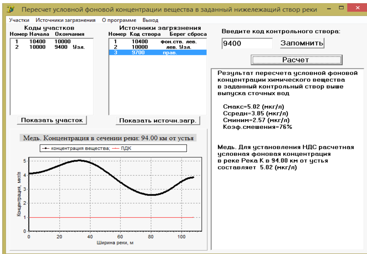
Рисунок Г.17 – Вид экранной формы представления результата перерасчета условной фоновой концентрации меди в створ G реки K
