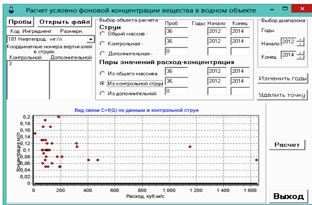
Рисунок Г.3 – Зависимость изменения содержания нефтепродуктов от расхода воды в створе G реки В
