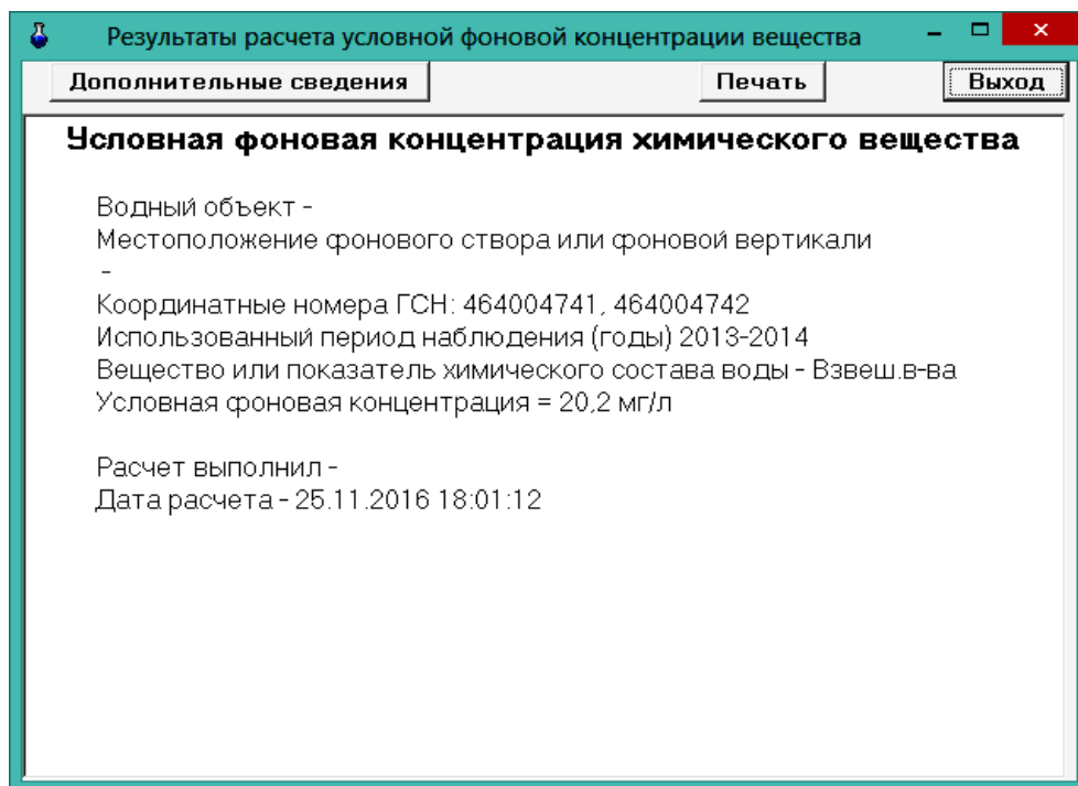
Рисунок Г.10 – Пример представления результата расчета условной фоновой концентрации химического вещества (взвешенных веществ)
