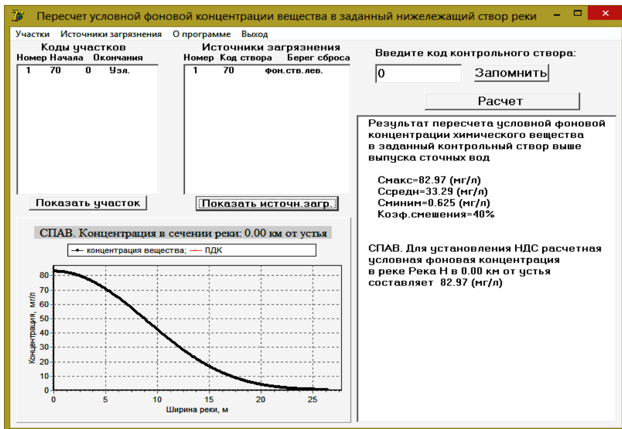
Рисунок Г.20 – Форма представления результата перерасчета условной фоновой концентрации СПАВ в створ М реки Н
