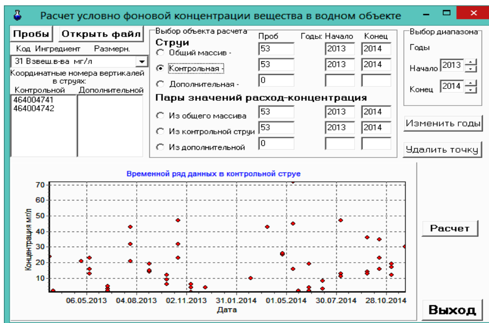
Рисунок Г.8 – Зависимость содержания взвешенных веществ от времени в створе В реки В
