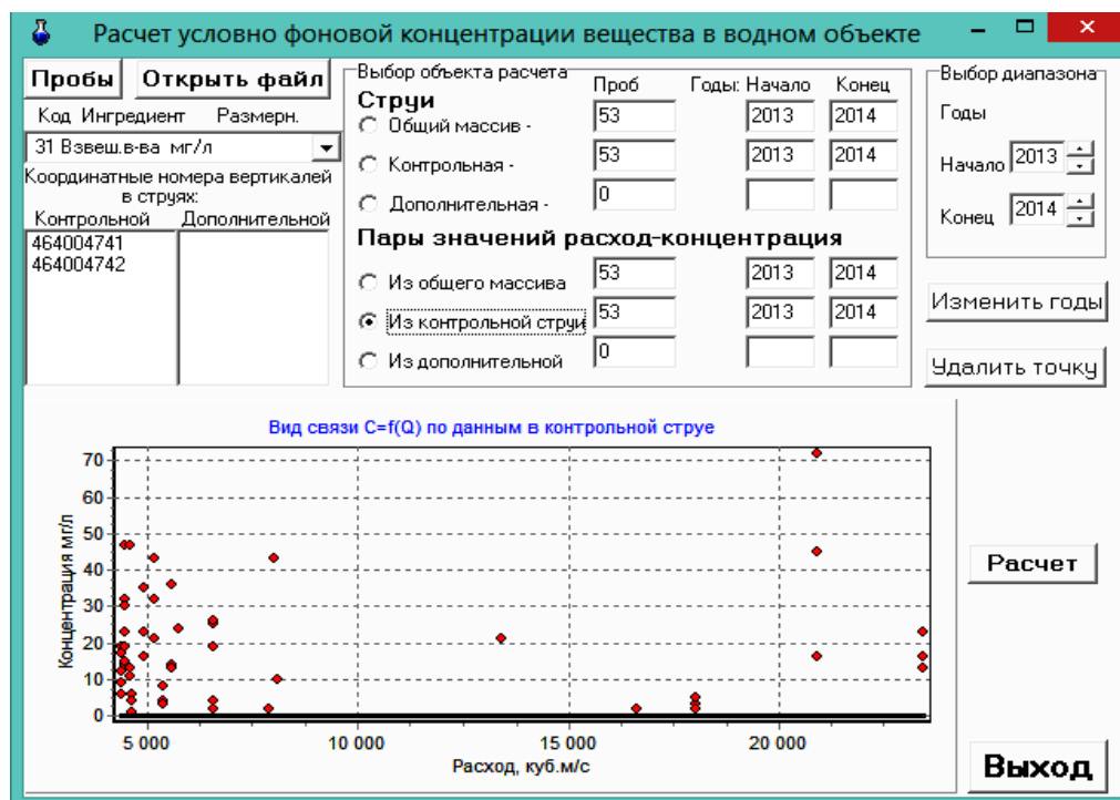
Рисунок Г.9 – Зависимость изменения содержания взвешенных веществ от расхода речной воды в створе В реки В
