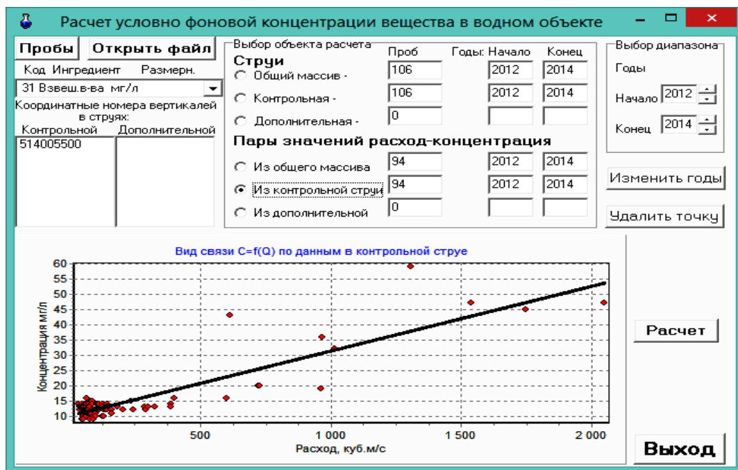
Рисунок Г.5 – Зависимость изменения содержания взвешенных веществ от расхода речной воды в створе О реки У
