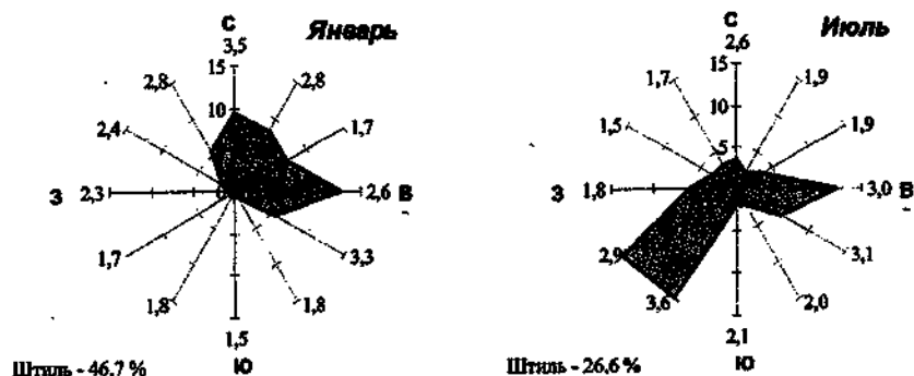
Рисунок 3 - Повторяемость, %, направлений ветра (роза ветров): на концах осей цифрами даны средние скорости ветра; направление ВПП с ЮВ на СЗ
