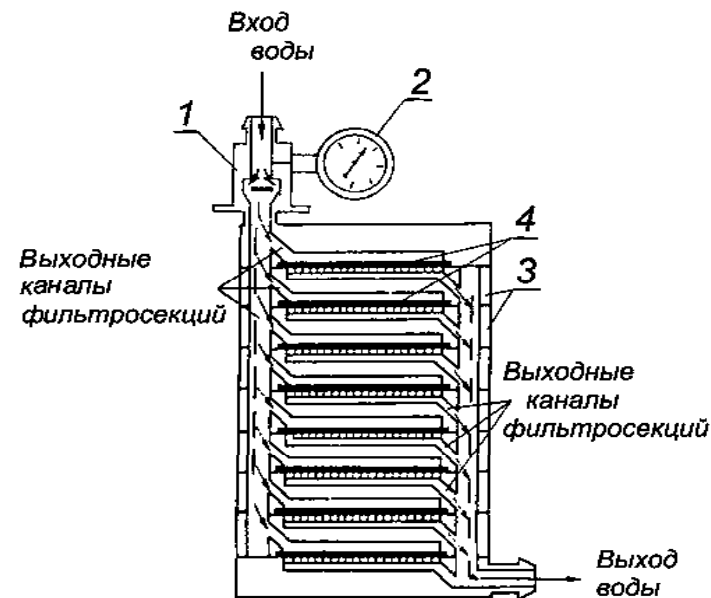
1 – обратный клапан; 2 – манометр; 3 – фильтрующие секции; 4 – фильтры
