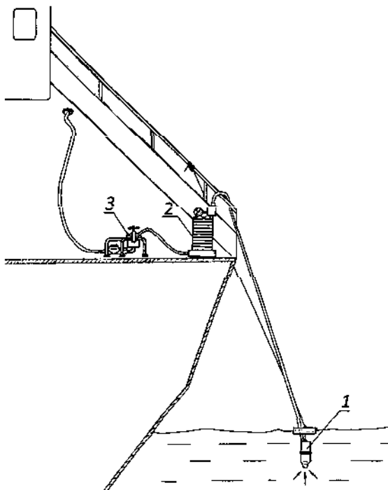
1 – погружной насос; 2 – установка фильтрующая «Мидия»; 3 – абсорбер «Морской»
