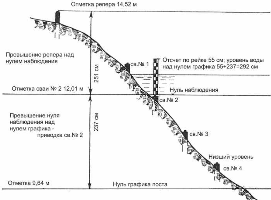
Рисунок 2 – Схема высотной основы гидрологического поста
