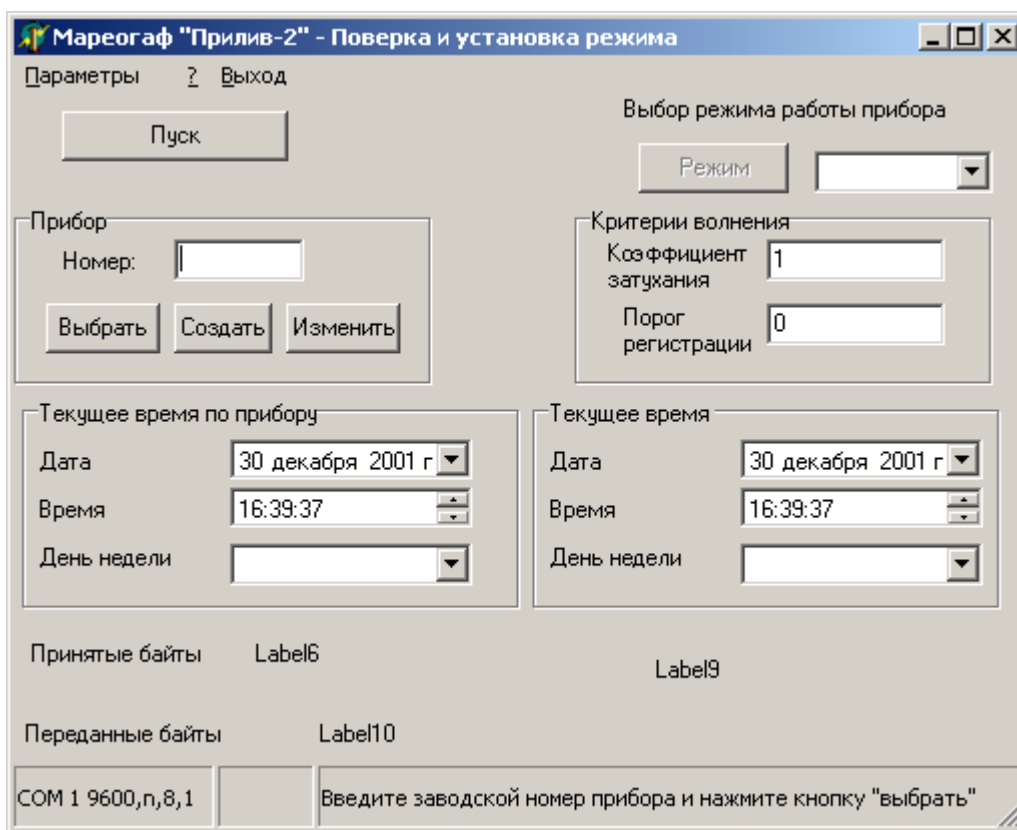
Рисунок 2 – Диалоговое окно "Поверка и установка режима". Пуск
