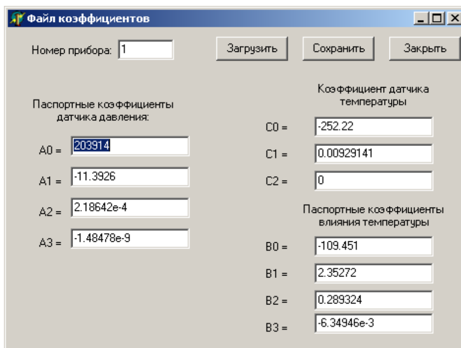
Рисунок 4 - Диалоговое окно "Файл коэффициентов". Файл коэффициентов
