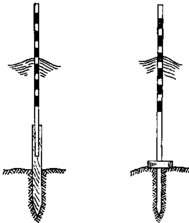
Рисунок 8.2 – Волномерные деревянные рейки
