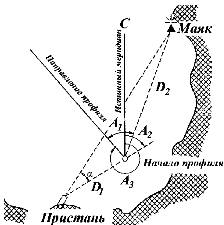
Рисунок 9.9 – Прокладка ледовых профилей
