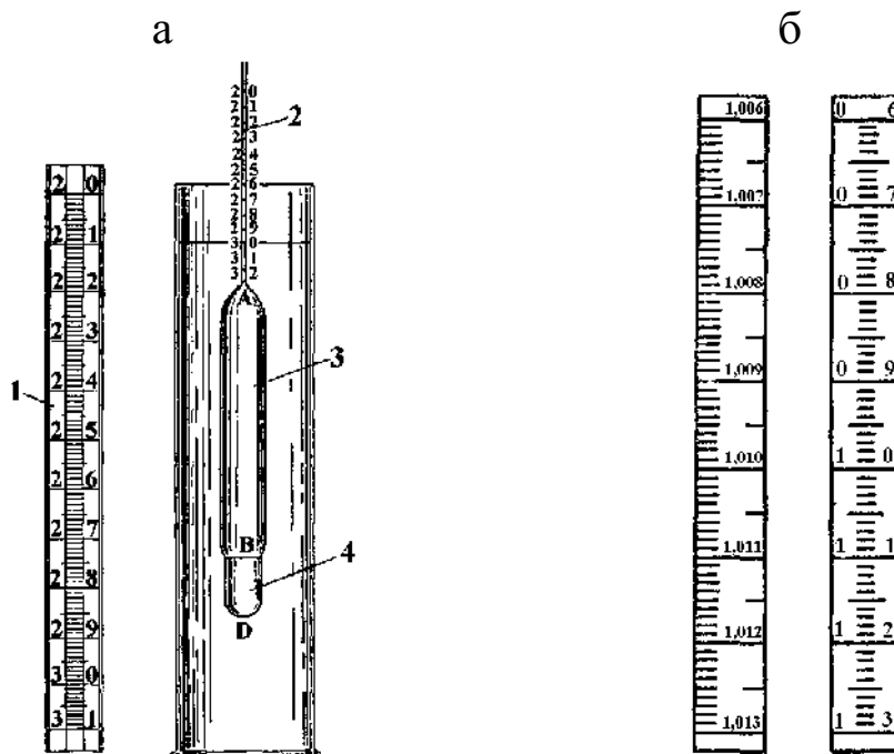
а – ареометр со шкалой; б – шкала ареометра; 1 – шкала; 2 – шейка ареометра; 3 – полый цилиндр (ареометр); 4 – шарообразный резервуар, заполненный дробью или ртутью.
