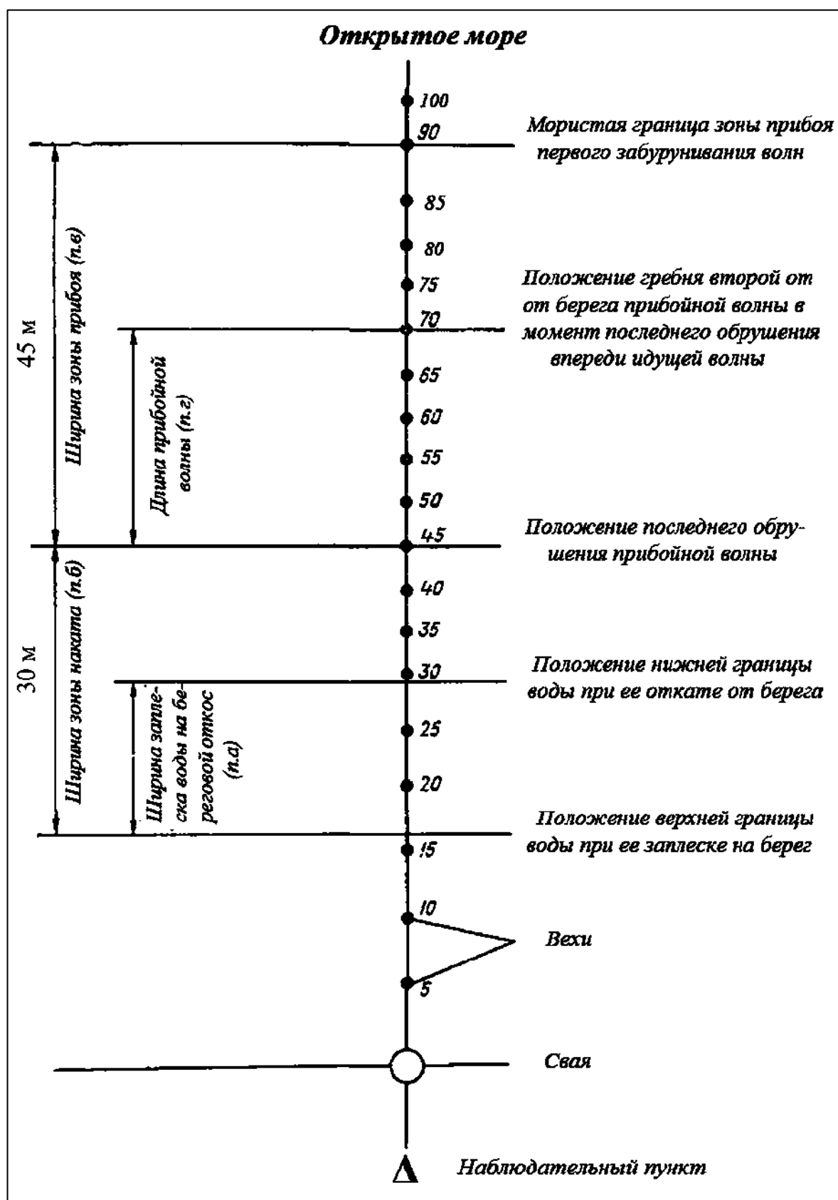
Рисунок 11.1 – Пункт наблюдений за морским прибоем
