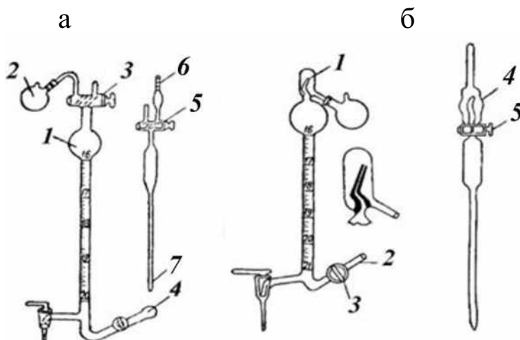
а – бюретка и пипетка Кнудсена; б – бюретка и пипетка ГОИН;
