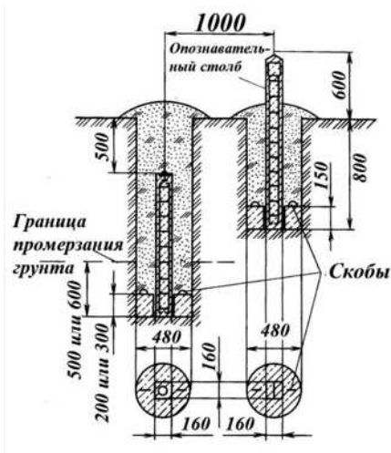
Рисунок 5.2 – Грунтовой репер (тип 160 оп. знак) с опознавательным столбом для районов с сезонным промерзанием грунта (размеры репера даны в мм)
