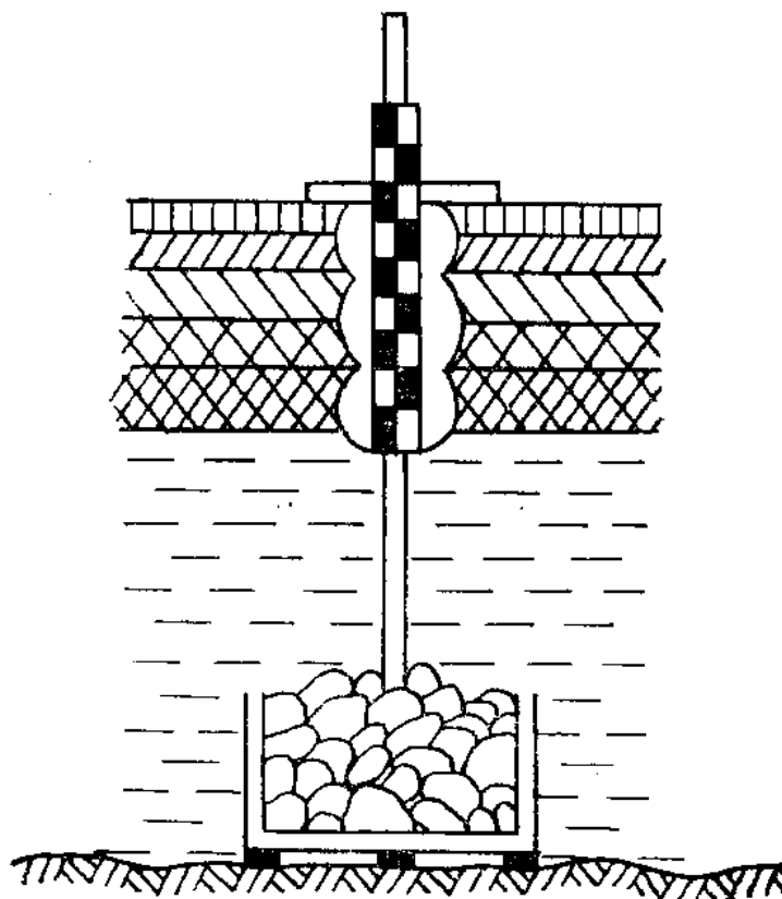
Рисунок 5.20 – Ледовая уровенная рейка в ящике с отоплением
