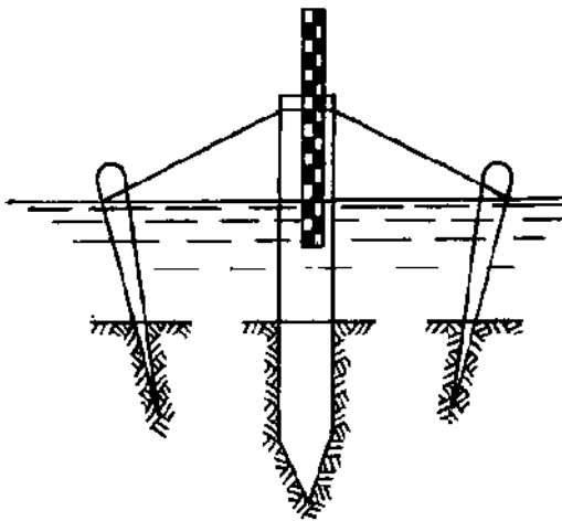
Рисунок 5.23 – Укрепление сваи при помощи растяжек
