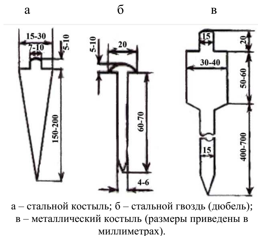
Рисунок 5.10 – Типы костылей, дюбелей, применяемые для установки реек при работе на разных грунтах
