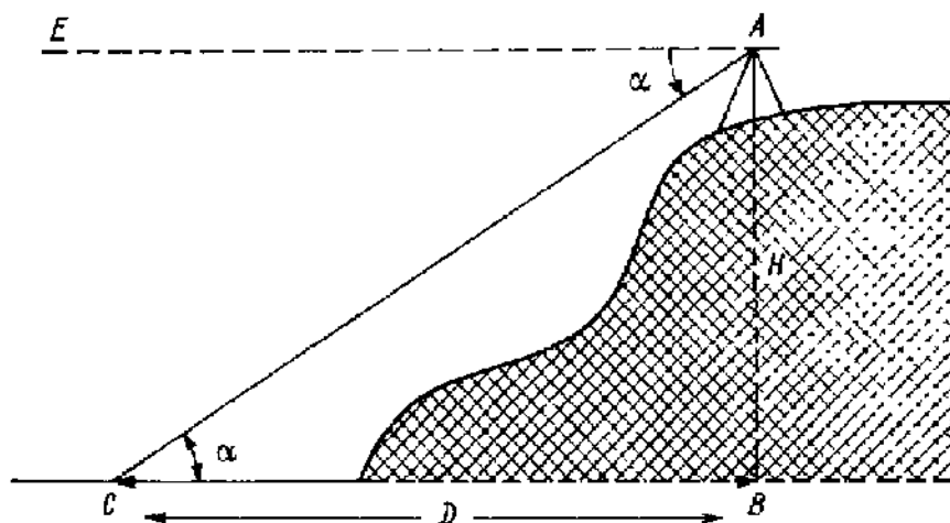
Рисунок 9.14 – Наблюдения за дрейфом льда одним теодолитом
