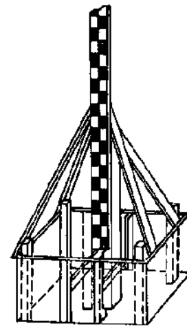
Рисунок 5.24 – Крепление уровенной рейки на ряже
