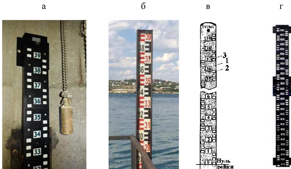
а – Металлическая рейка длиной 4 м; б – Деревянная рейка длиной 4 м; в – Металлические рейки ГМ-3: длиной 4,0 м; г – длиной 2,8 м; 1 – металлическая рейка; 2, 3 – прорези с фарфоровыми вкладышами, размерами соответственно (20X32) и (40X52) мм.
