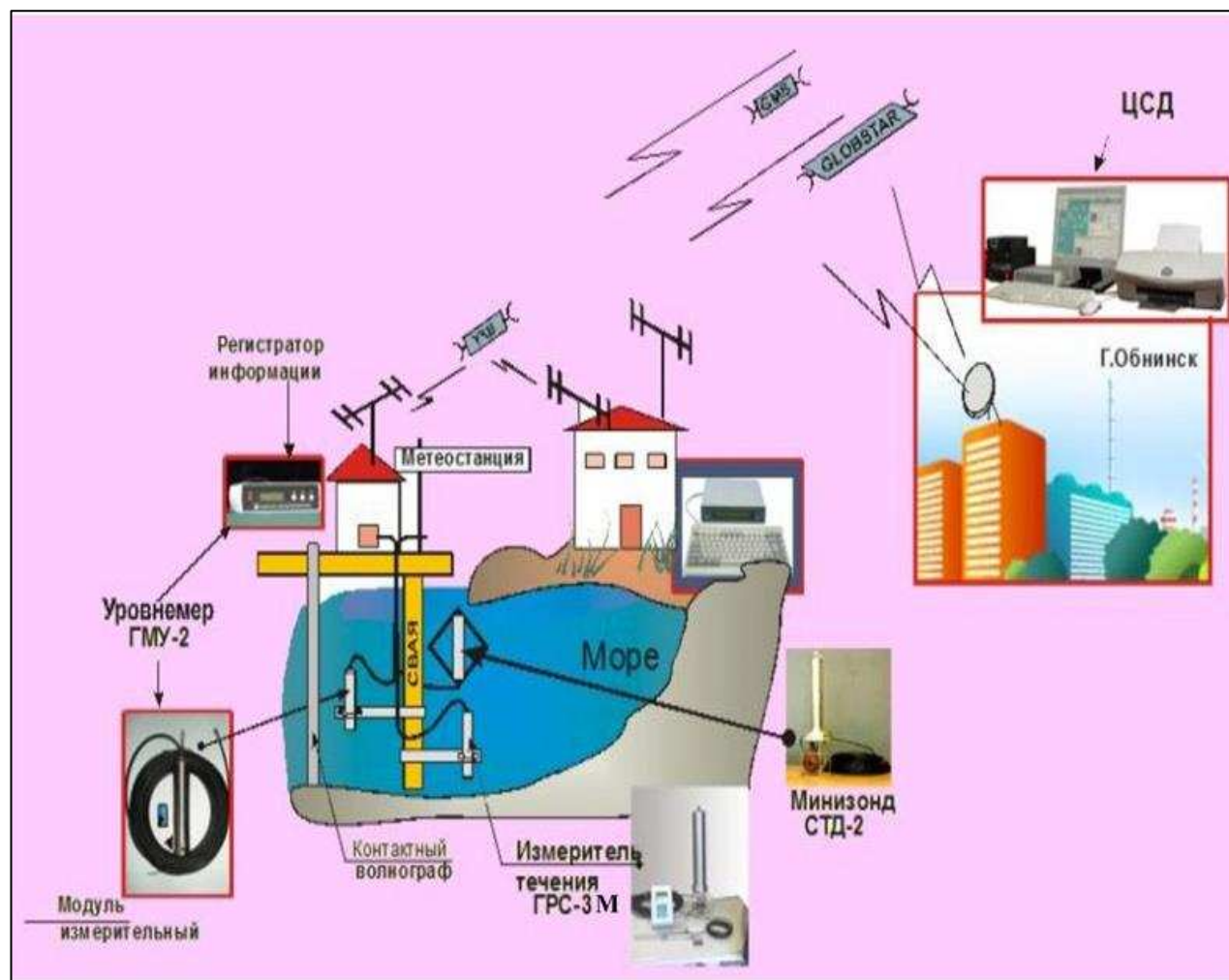
Рисунок 13.1 – Принципиальная схема работы морской автоматизированной гидрометеорологической станций
