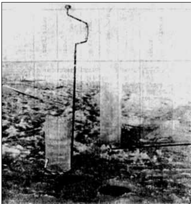
Рисунок 9.18 – Образцы льда – керны, полученные кольцевым буром ПИ-8
