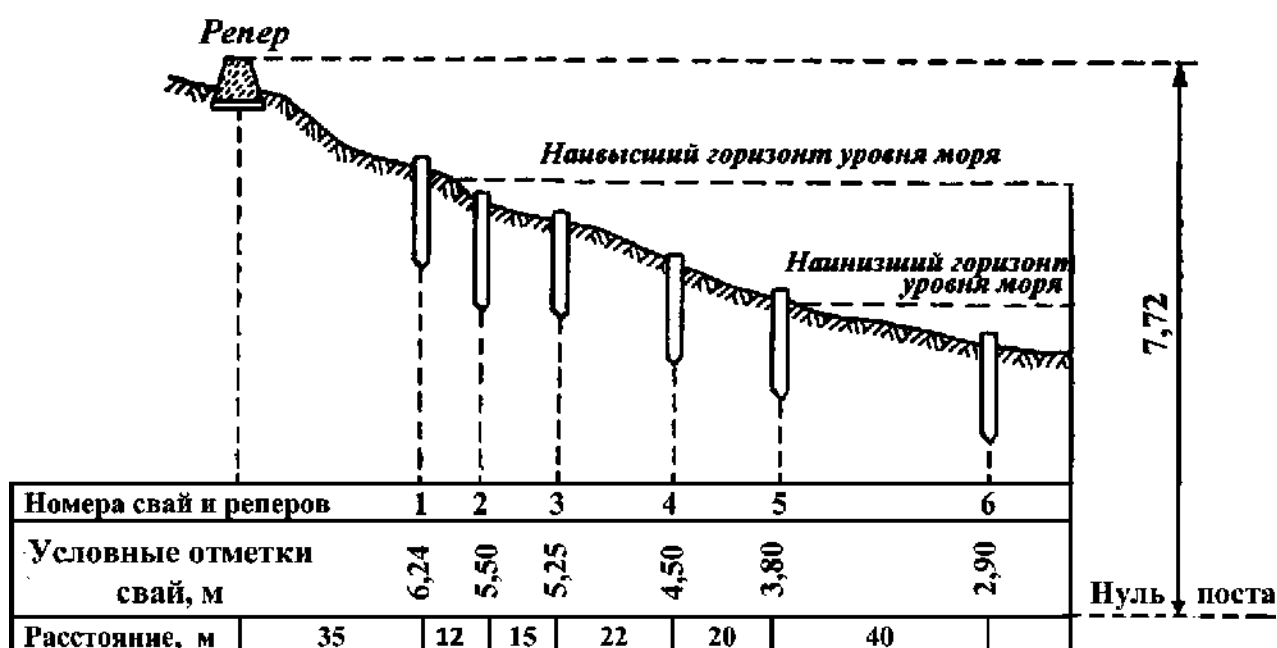
Рисунок 5.25 – Схема свайного морского уровенного поста
