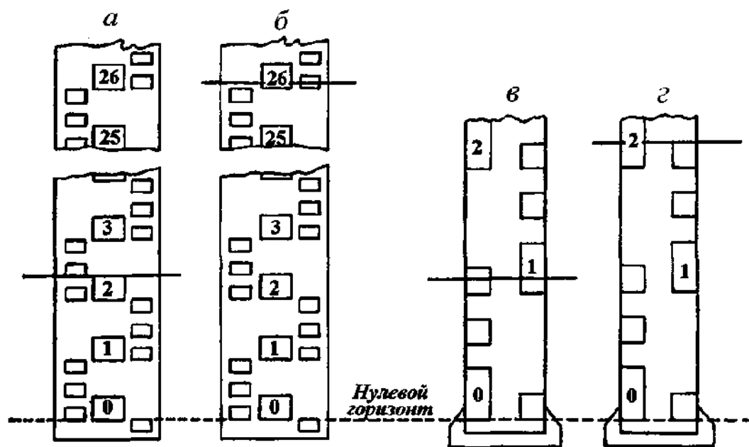
Рисунок 5.27 – Отсчеты по морским металлическим уровенным рейкам
