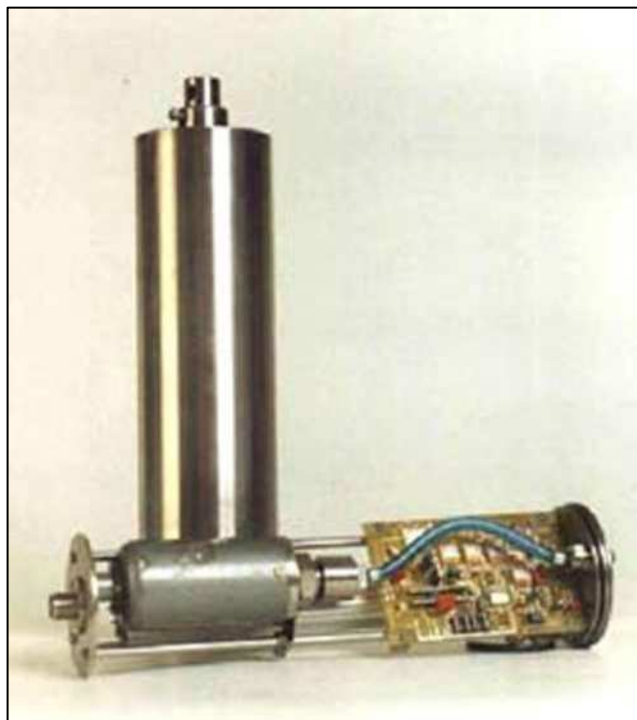
Рисунок 13.3 – Преобразователь гидростатического давления «Прилив-2»
