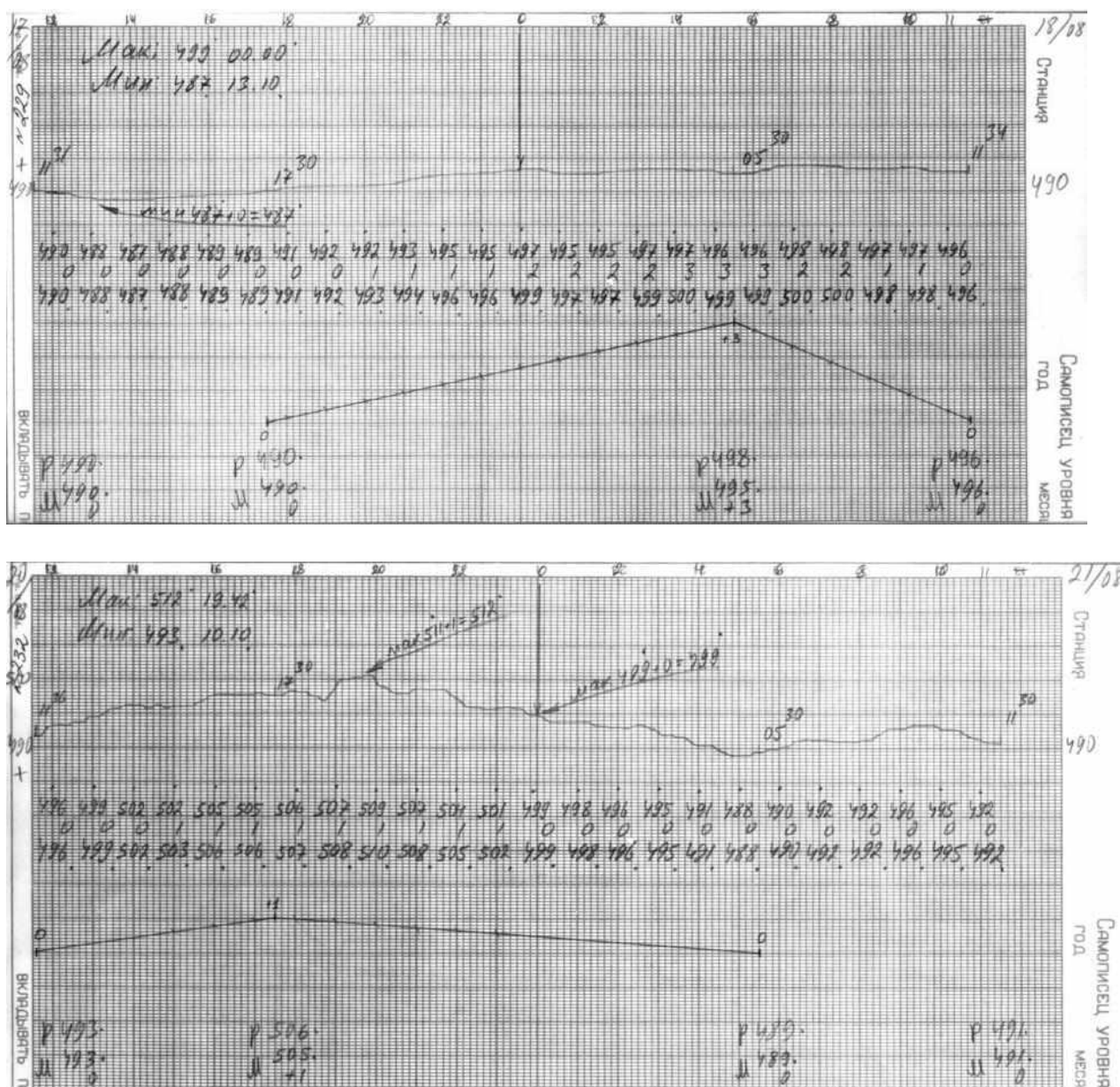
Рисунок 5.38 – Ленты СУМ с графическим методом определения поправок
