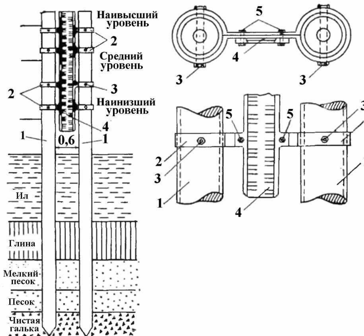
Рисунок 5.21 – Крепление морской уровенной рейки к двум сваям
