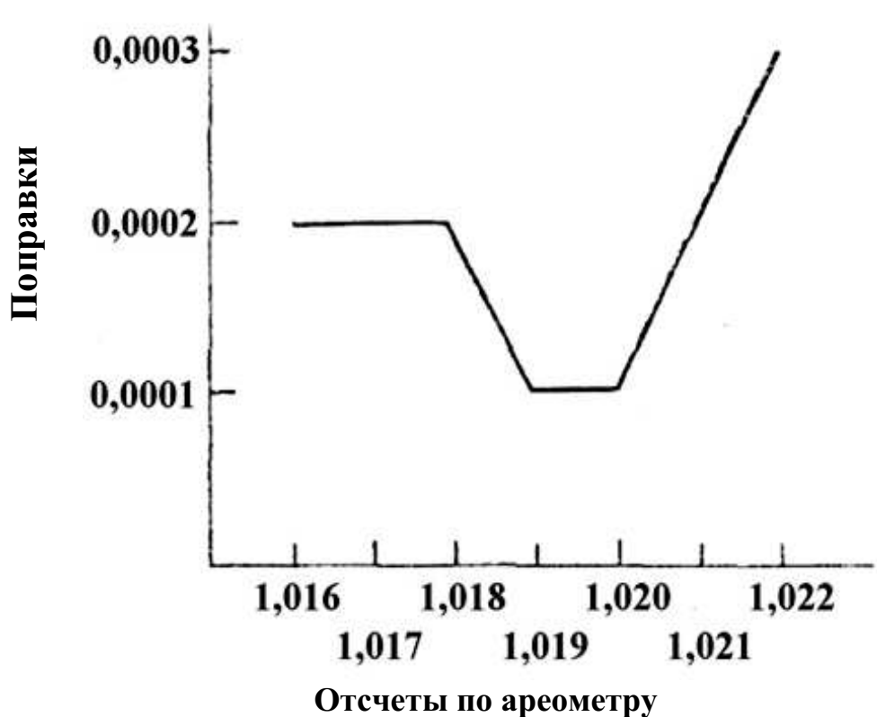
Рисунок 7.5 – График поправок ареометра
