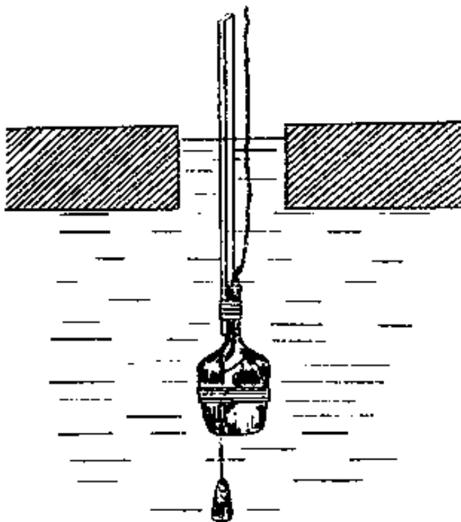
Рисунок 7.2 – Бутылка для отбора проб воды со льда
