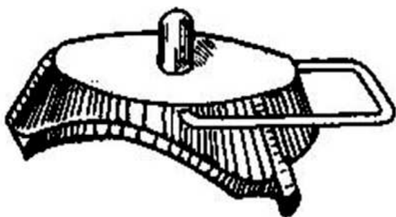
Рисунок 5.7 – Приспособление для установки нивелирных реек – башмак
