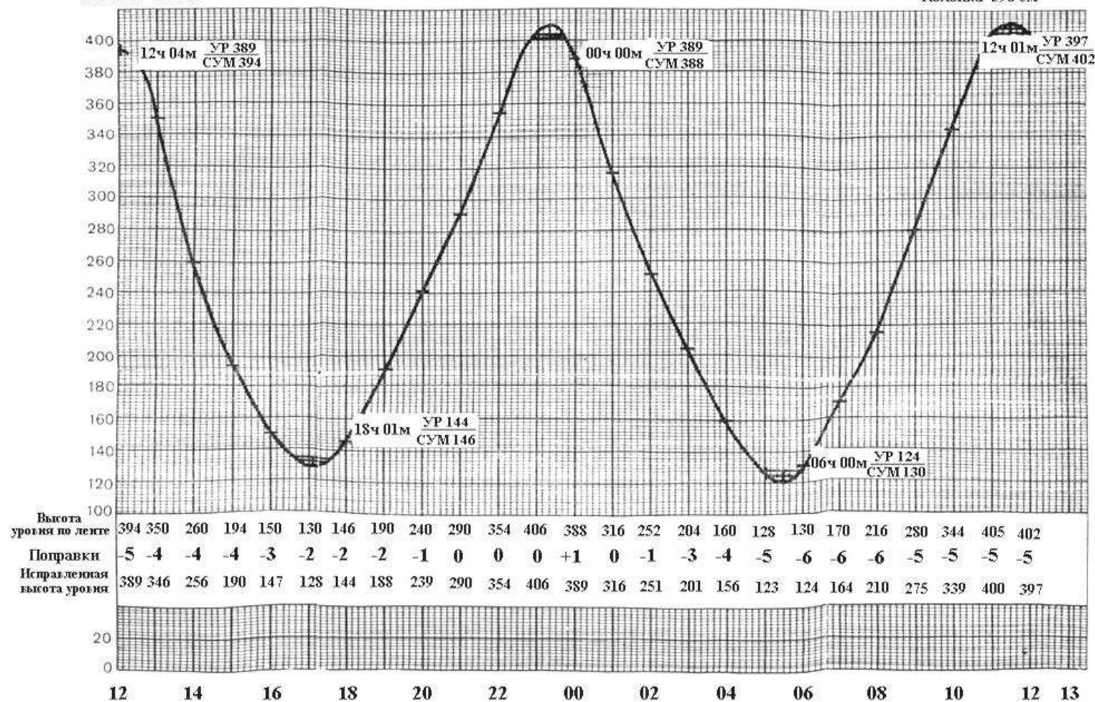
Рисунок 5.37 – Обработка ленты СУМ по отсчетам уровенной рейки
