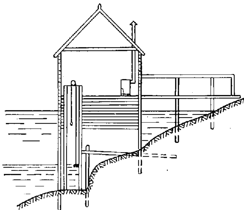
Рисунок 5.33 – Установка СУМ у откоса берега
