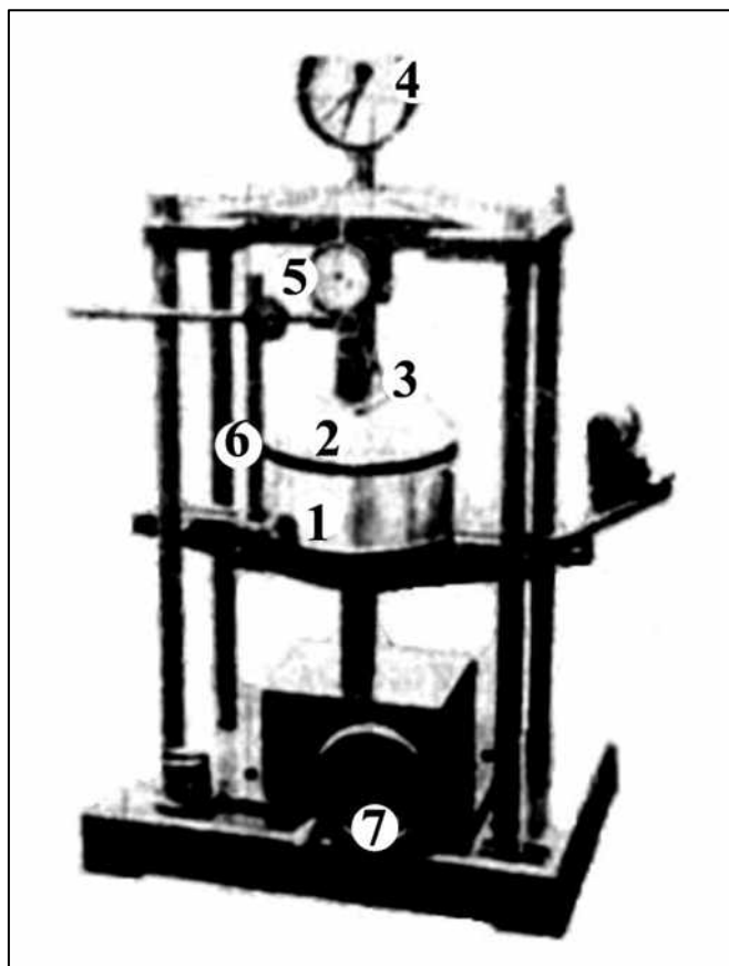
1 – подставка; 2 – ледяной диск; 3 – пуансон; 4 – шкала нагрузки; 5 – индикаторная головка; 6 – штатив для закрепления индикаторной головки; 7 – ручка пресса.
