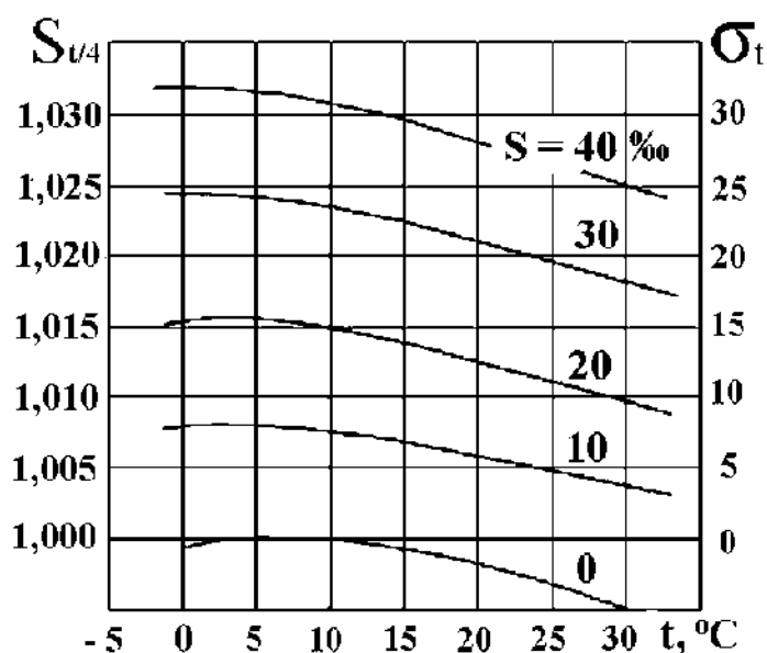
Рисунок 7.1 – Связь условной плотности морской воды ( \sigma_t ) с ее солёностью ( S ) и температурой ( t )
