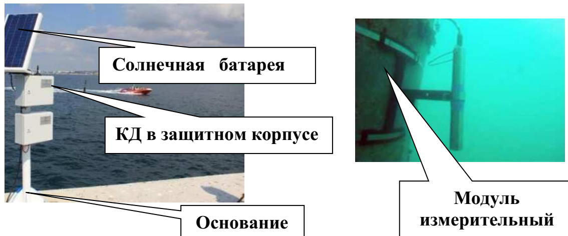
Рисунок 13.4 – Комплекс гидрологический ГМУ-4
