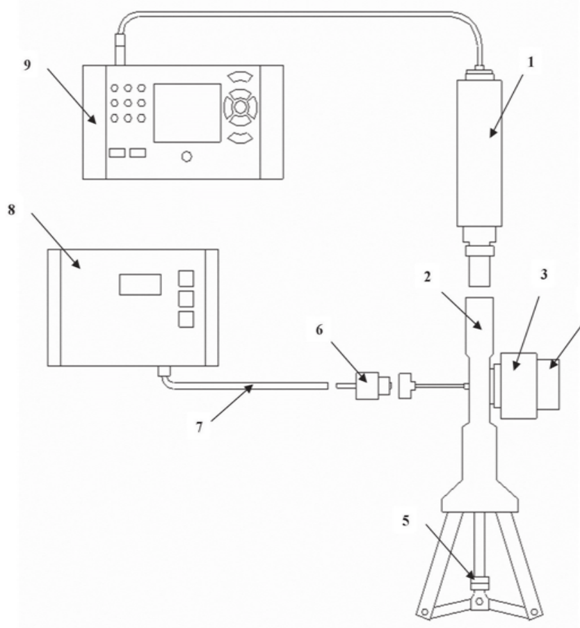
1- эталонный датчик CPT 6000; 2 - насос CPP 30; 3 - вентиль регулировки давления; 4- вентиль спуска/запора давления; 5 - стопорные гайки; 6 – переходник; 7- воздушный шланг для компрессора (вакуумный шланг); 8 - уровнемер PS-LIGHT-II; 9 - калибратор CPH 6000
