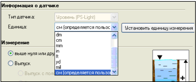
Рисунок 6 – Окно ПО «SEBAConfig: Maintenance Tool» со списком размерностей величины давления
