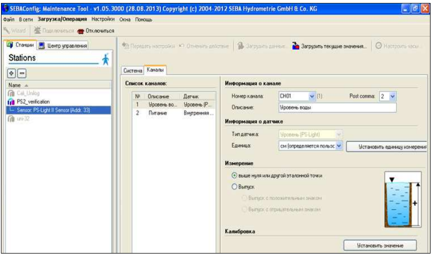
Рисунок 5 – Окно ПО «SEBAConfig: Maintenance Tool»
