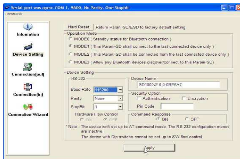
Рисунок Б.17 – Конфигурация соединения
