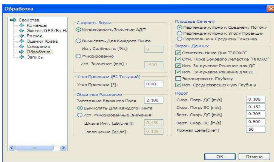
Рисунок 13 – Вид панели «Обработка» при открытии файла «Конфигурации воспроизведения»
