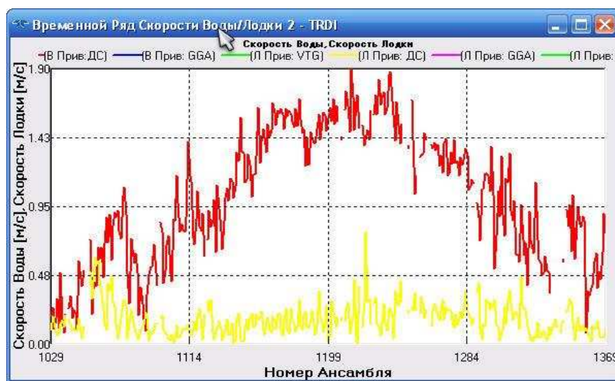
Рисунок 21 – Графики скорости судна и потока
