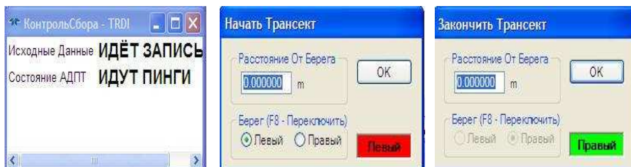
Рисунок 11 – Контроль сбора данных и запись расстояний до урезов в начале и конце пересечения (трансекты)
