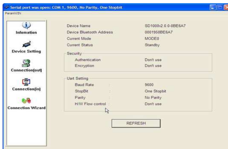
Рисунок Б.14 – Информация о соединении
