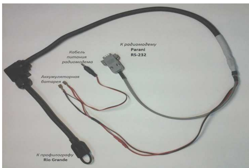
Рисунок Б.3 — Кабель радиомодема
