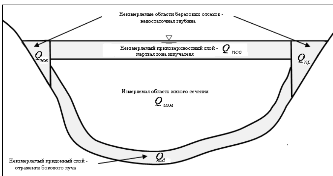
Рисунок 1 – Схема поперечного сечения потока
