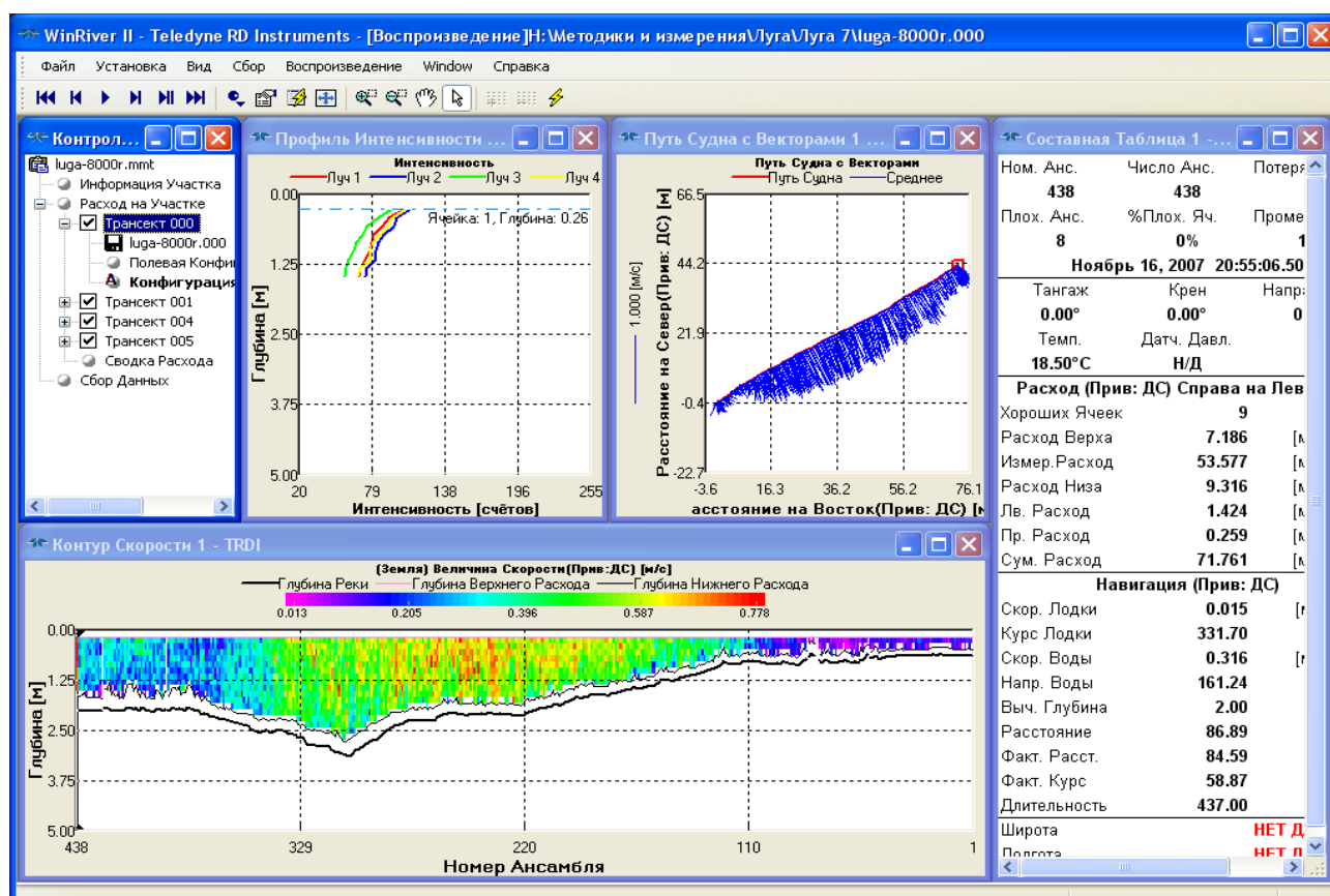
Рисунок 5 – Главный экран программы «WinRiver II»
