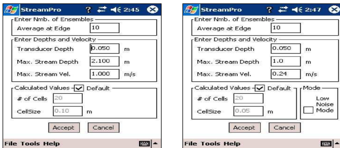
Рисунок 2 – Окна КПК во время изменения значений параметров измерений
