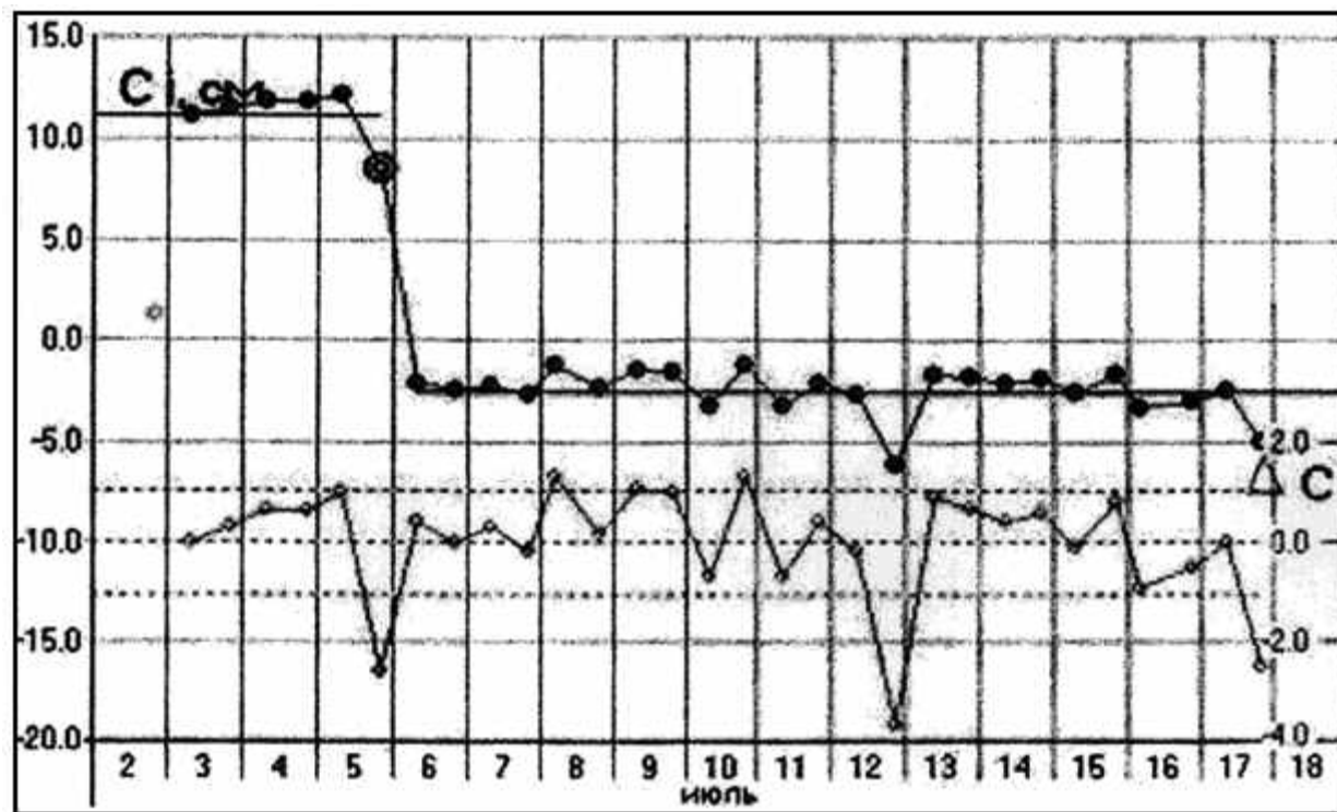
Рисунок 5.7 - Анализ смещений отклонения поправки \Delta C_i . Поиск необратимого смещения
