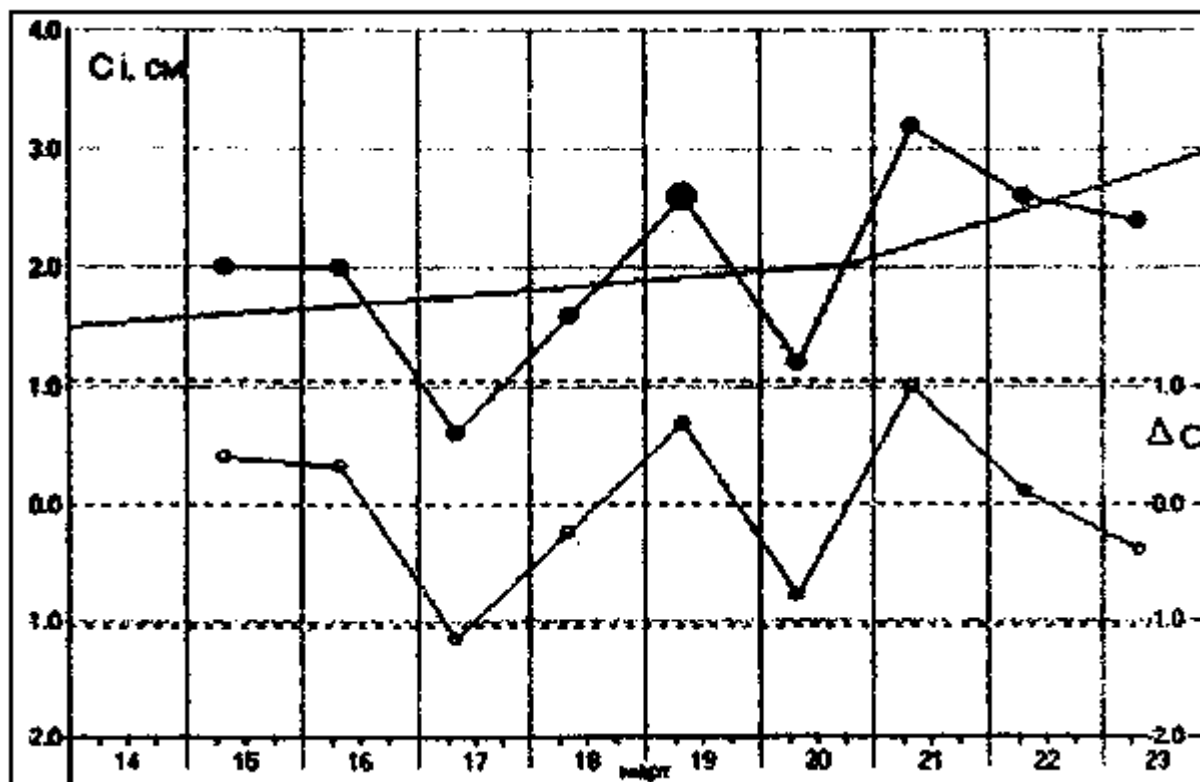
Рисунок 5.9 - Поиск обратимого смещения поправки \Delta C_i
