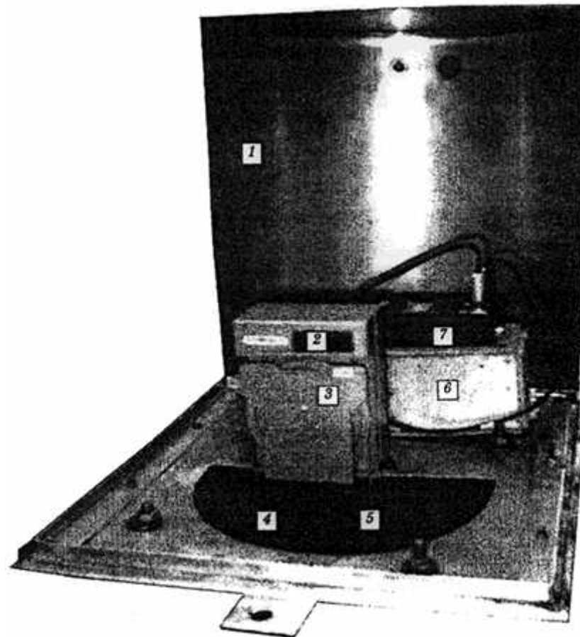
Рисунок А.1 - Уровнемер поплавковый цифровой
