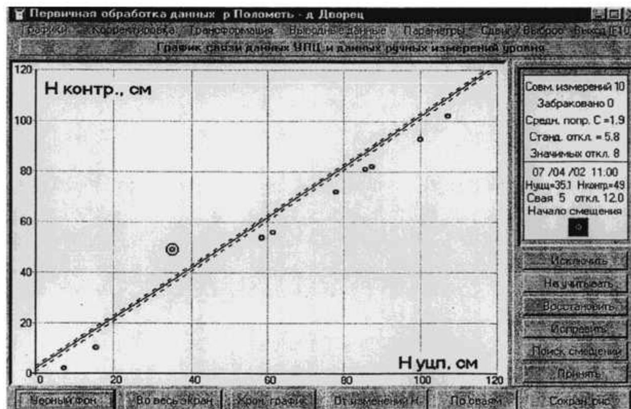
Рисунок 5.5 - График связи H_{\text{контр}} = f(H_{\text{ушп}})
