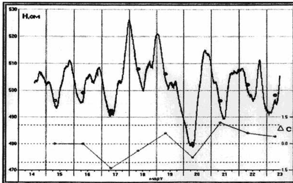
Рисунок 5.6 - Комплексный график хода уровня по данным записи УПЦ и контрольных измерений уровня воды и хода отклонений поправки \Delta C_i
