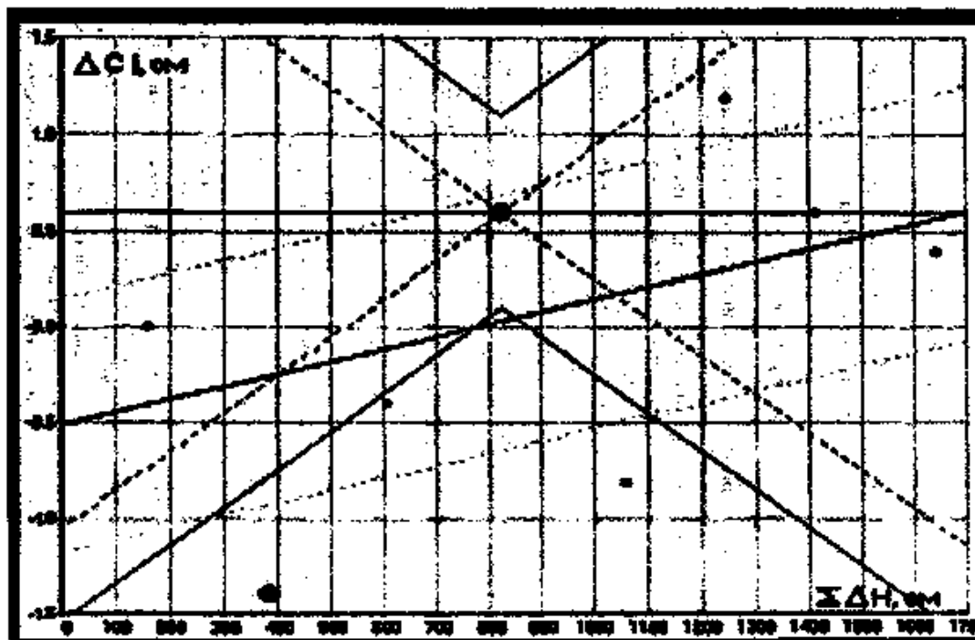
Рисунок Г.1 - Анализ связи поправок с нарастающими суммами изменений уровня воды
