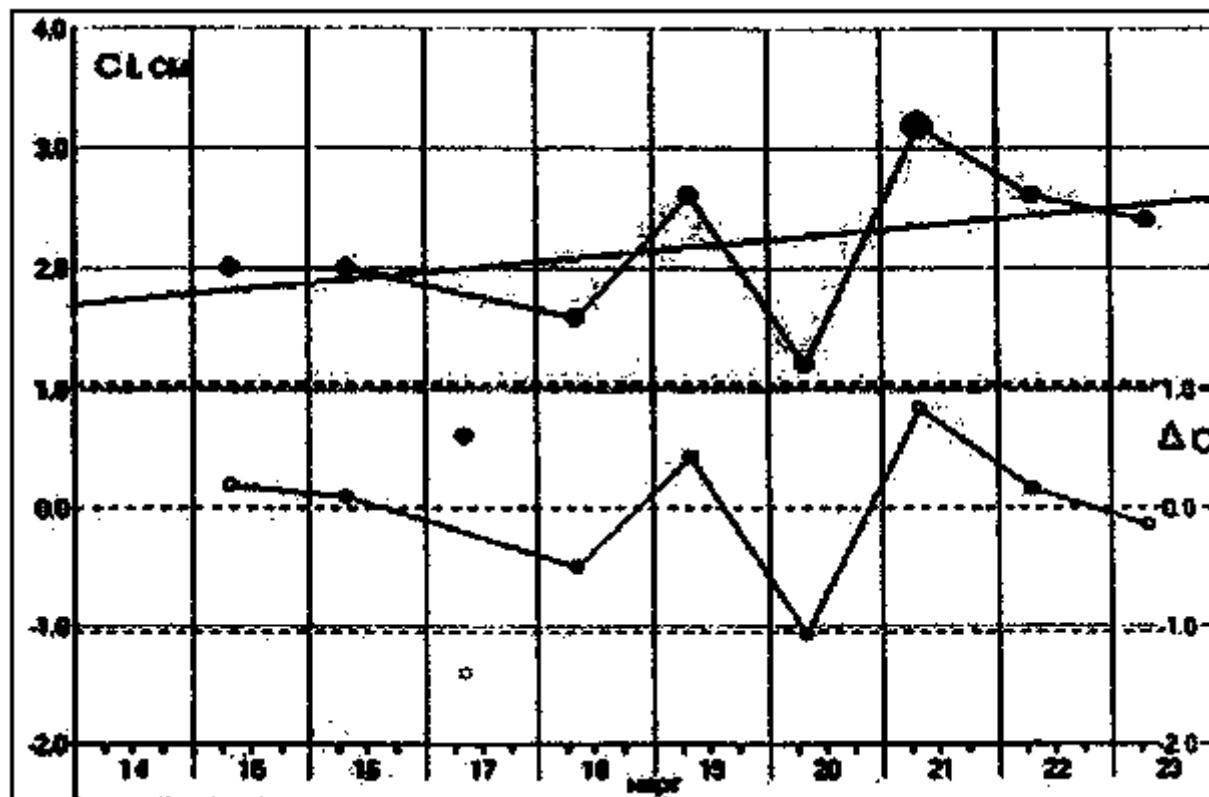
Рисунок 5.8 - Анализ линейного смещения поправки \Delta C_i
