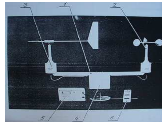
1 — траверса; 2 — анемометр; 3 — румбометр; 4 — БОИ; 5 — БП; 6 — БК
