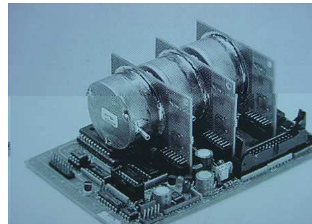
Рисунок А.12 — Датчик атмосферного давления DPA21
