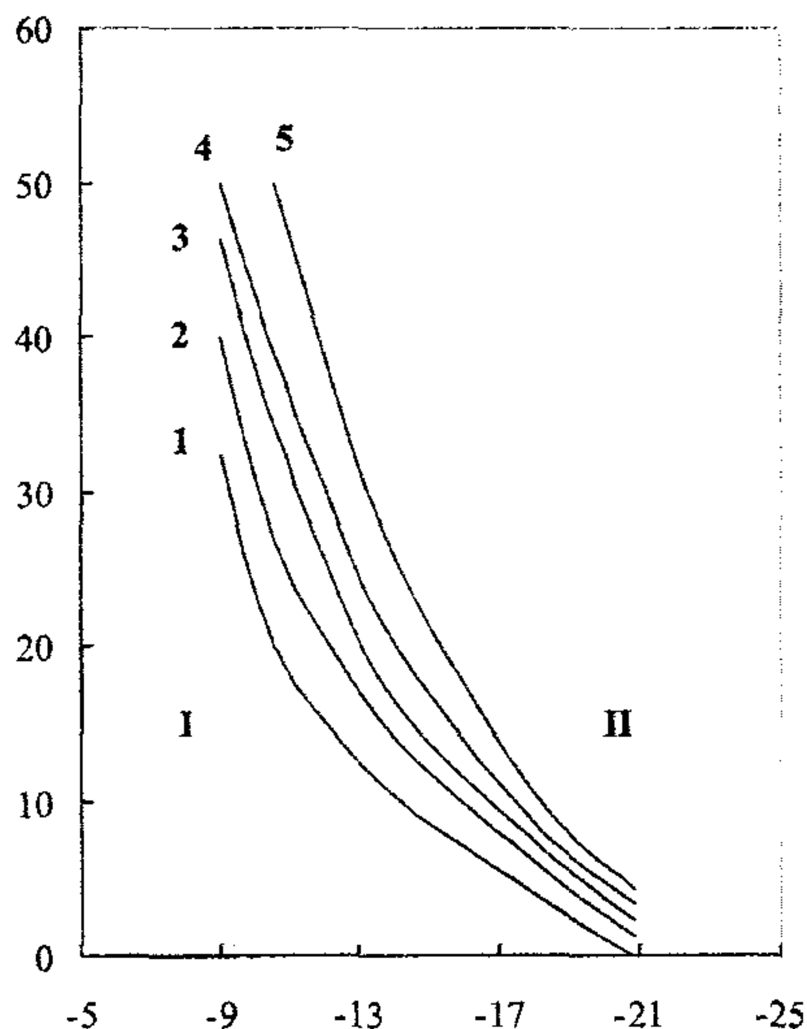
Рис. 8.6 – Номограмма для оценки целесообразности введения реагента в облако по известным t_{вг} и \bar{w} . I – область t_{вг} и \bar{w} , при которых введение реагента целесообразно; II – область t_{вг} и \bar{w} , при которых введение реагента нецелесообразно; 1, 2, 3, 4, 5 – \bar{q} = 0,5; 0,4; 0,3; 0,2; 0,1 г/м 3 соответственно
