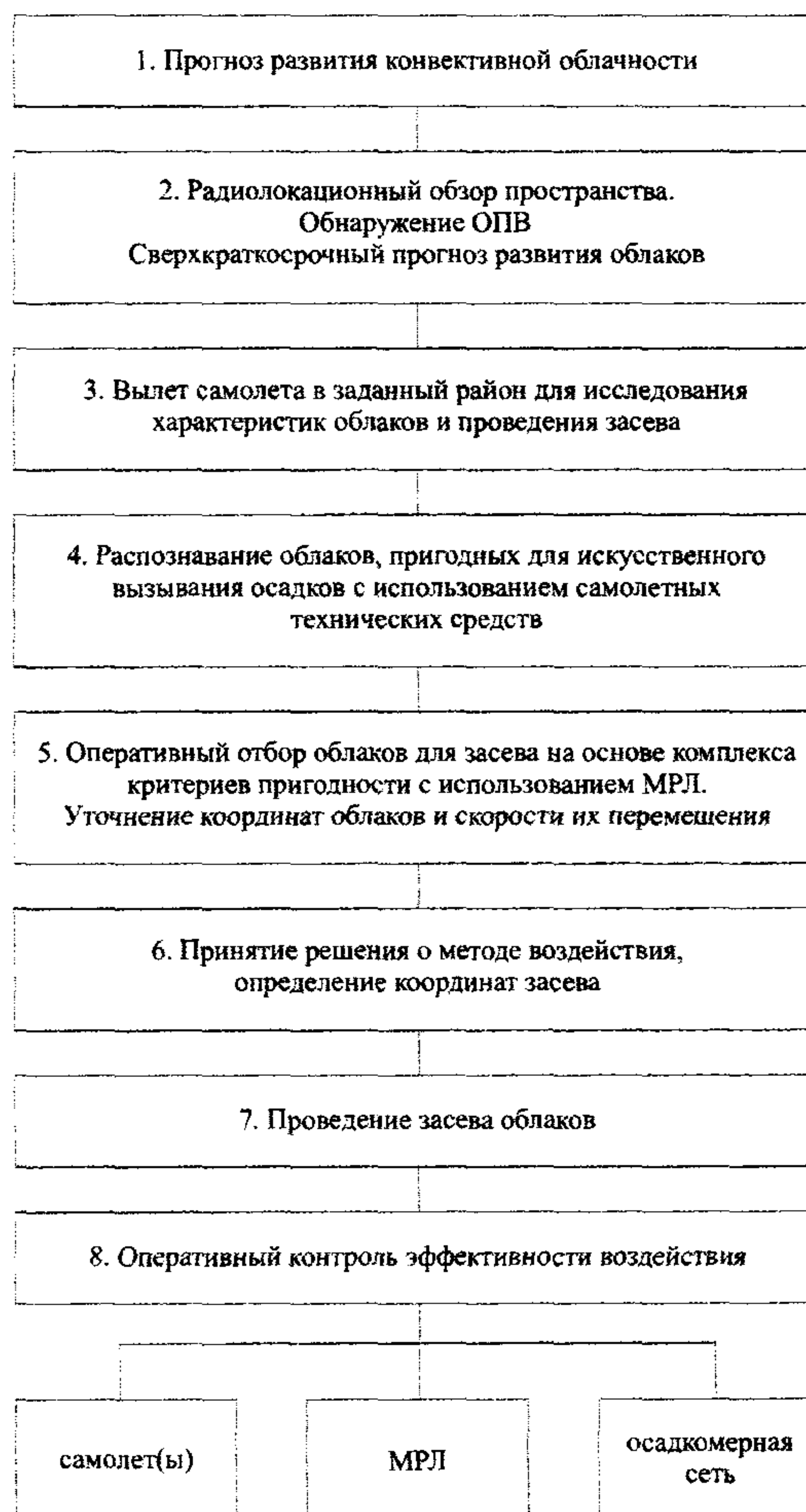
Рис. 8.11 – Блок-схема операций по воздействию на конвективные облака.
