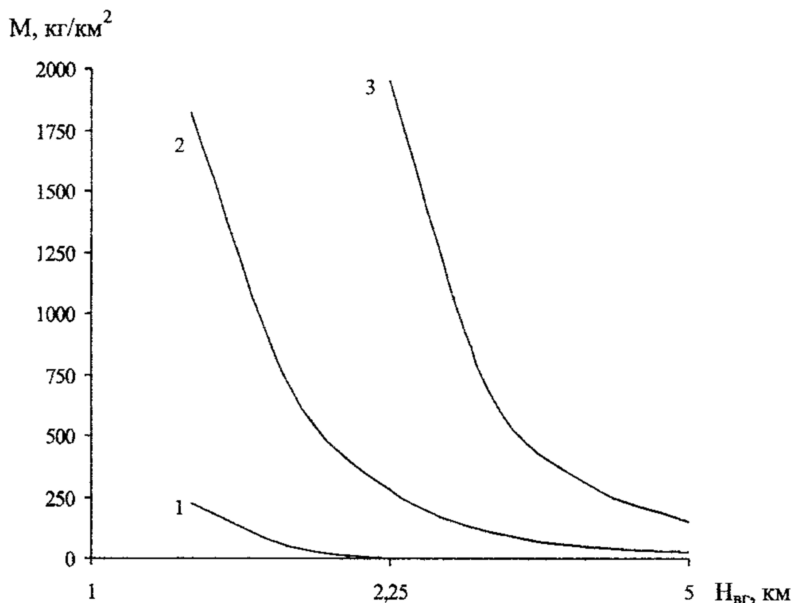
Рис. 8.2 — Зависимость оптимального количества реагента M от H_{\text{вг}} и r_0 . 1 — r_0 = 30 мкм, 2 — r_0 = 60 мкм, 3 — r_0 = 100 мкм
