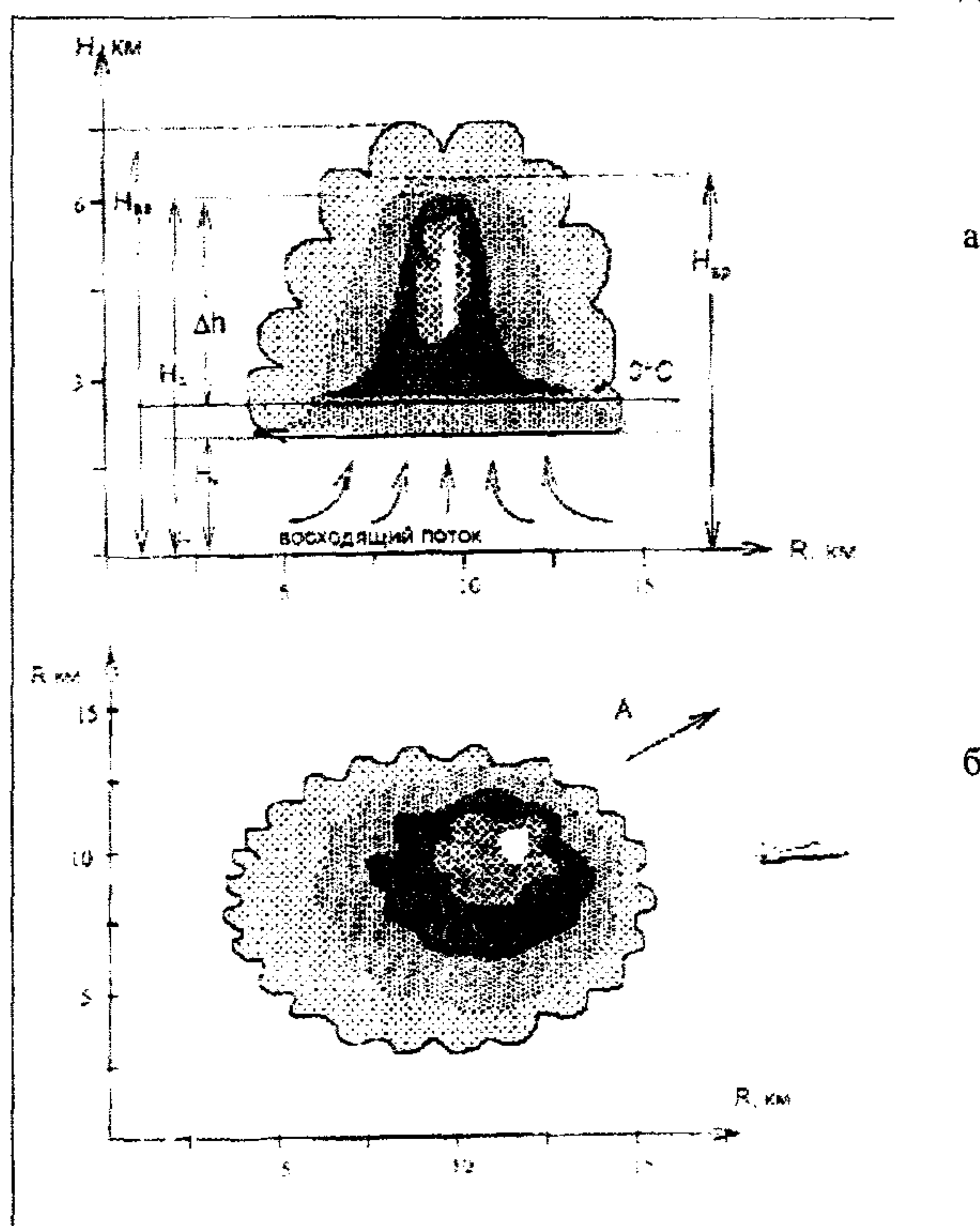
Рис. 8.12 – Схема засева одноячейкового мощно-кучевого облака (Cu Cong) а – вертикальный разрез облака, б – горизонтальный разрез облака.
