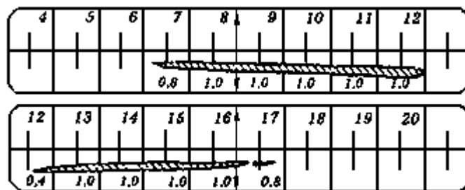
Рисунок 7 - Запись на ленте гелиографа при неправильной установке прибора по широте
