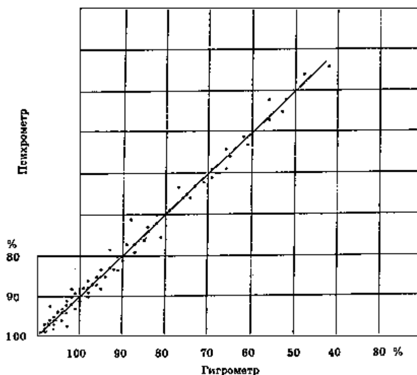
Рисунок 3 - График сравнения гигрометра и психрометра (ТМ-9) при выходе стрелки за отметку 100% шкалы гигрометра
