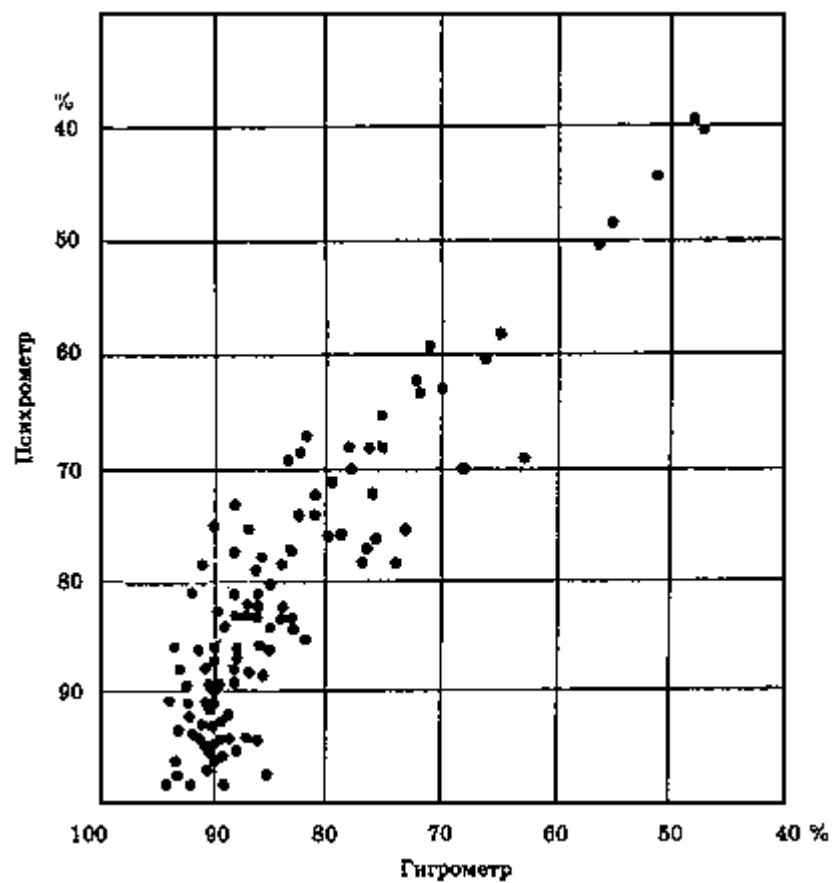
Рисунок 1 - График сравнения гигрометра и психрометра (ТМ-9) при пониженной чувствительности волоса гигрометра
