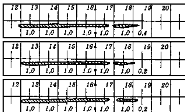
Рисунок 8 - Запись на лентах гелиографа при затенении прибора в промежутке времени 16-17 ч
