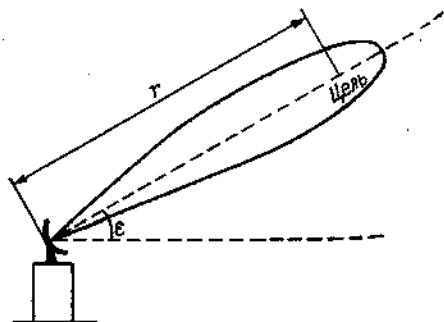
Черт. 1.4. Координаты цели. r — наклонная дальность; \varepsilon — угол возвышения антенны.
