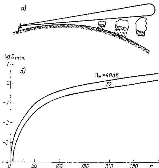
Черт. 1.15. Ограничения радиолокационного метода наблюдений: за счет подъема диаграммы направленности антенны над сферической Землей (а) и за счет увеличения минимально обнаружимой отражаемости при заданном потенциале (б).
