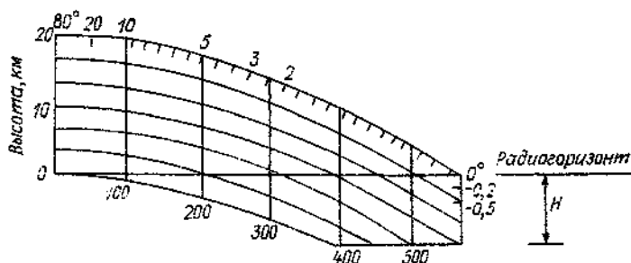
Черт. 1.7. Радиолуч над сферической Землей при нормальной рефракции и антенне, расположенной на поверхности Земли ( h^* = 0 ).
