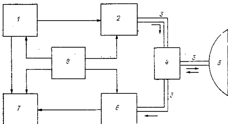
Черт. 1.1. Функциональная схема импульсной радиолокационной станции.
