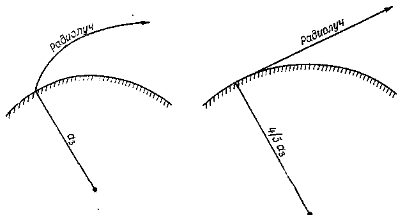
Черт. 1.6. Увеличение радиуса Земли в 4/3 раза позволяет изобразить траекторию радиоволн в виде прямой линии.
