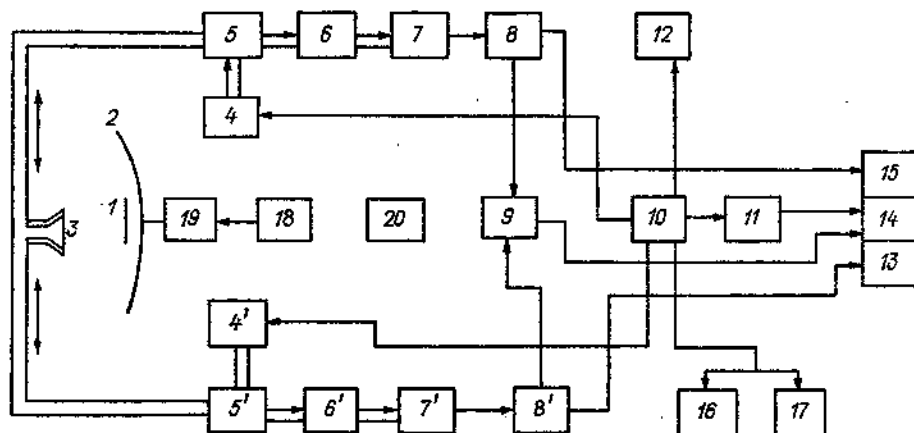
Черт. 6.8. Структурная схема радиолокатора МРЛ-5.
