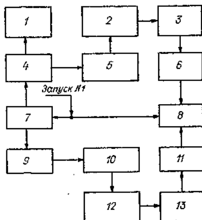
Черт. 7.3. Структурная схема подключения аппаратуры для измерения чувствительности приемных устройств, градуировки СВЧ-аттенюаторов, блока обработки видео и системы коррекции на квадрат расстояния.
