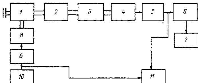
Черт. 7.2. Схема подключения приборов для измерения чувствительности и градуировки системы ступенчатого изохза МРЛ-2.
