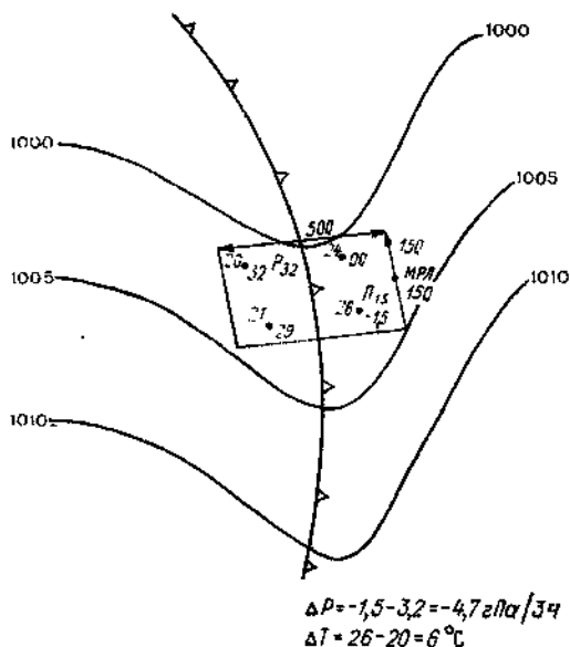
Черт. 5.14. Пример определения разности тенденций давления для уточненного синоптико-радиолокационного варианта метода прогноза шквалов.
