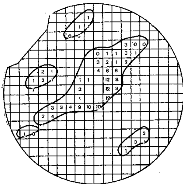
Черт. 3.1. Пример записи углов возвышения антенны \epsilon на прозрачном шаблоне с координатной сеткой.
