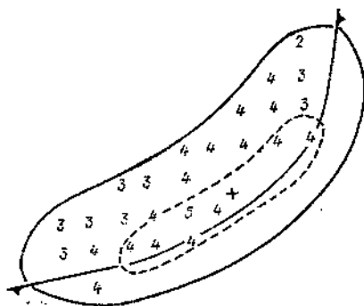
Черт. 5.4. Типичная конфигурация радиоэха облачности и осадков холодного фронта первого рода.
