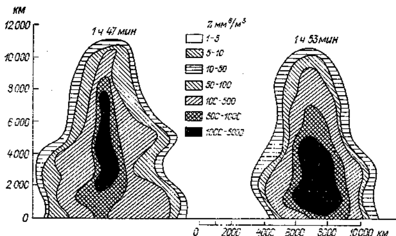
Черт. 2.8. Изменение отражаемости во времени в грозовом облаке по данным за 17 августа 1954 г. (по данным Е. М. Сальмана).
