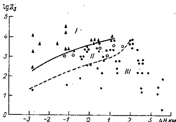
Черт. 5.10. График индикации пикаристых усиления ветра по данным измерений МРЛ.
