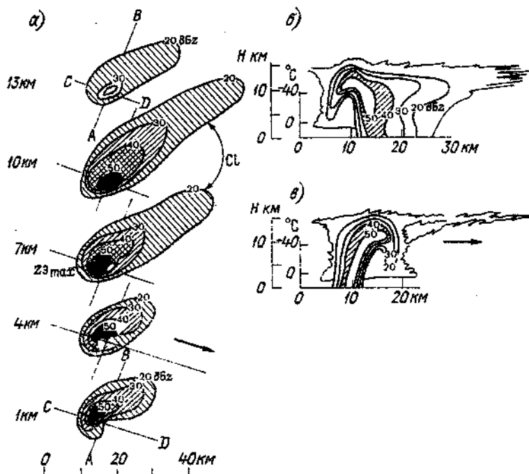
Черт. 2.4. Схематическое изображение структуры суперячейки по данным МРЛ.
