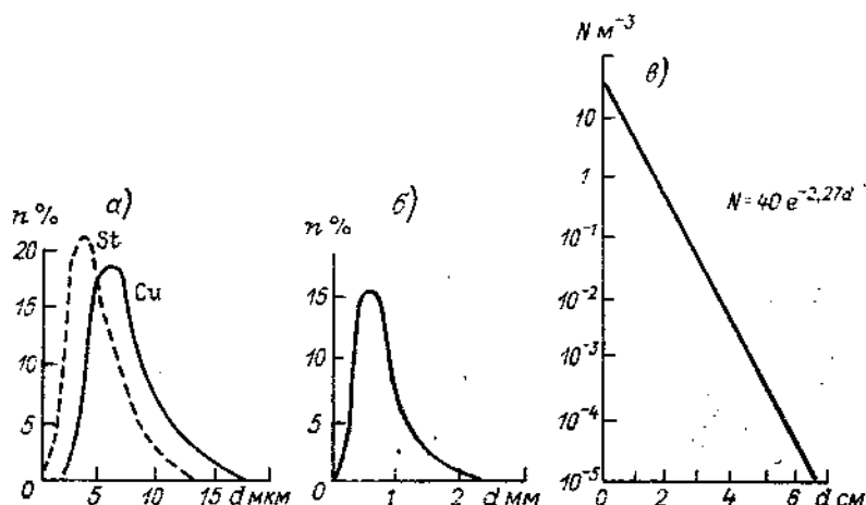
Черт. 1.12. Гистограммы капель по размерам в облаках, осадках и граде.
