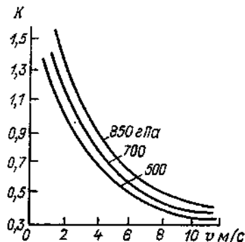
Черт. 4.4. Зависимость коэффициента K от скорости ветра v на изобарических поверхностях 850, 700 и 500 гПа.
