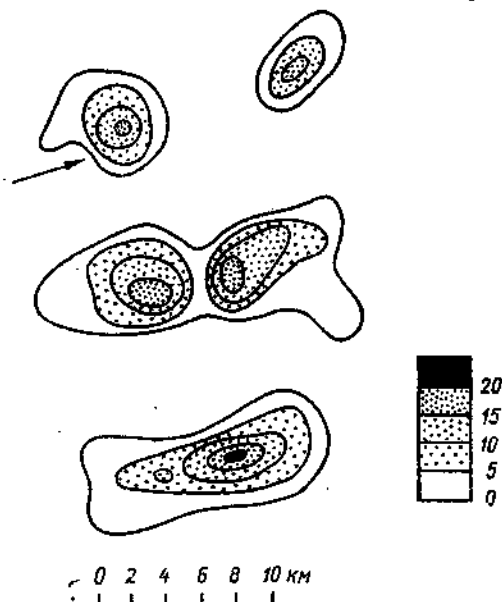
Черт. 2.2. Слияние радиоэха двух ячеек.
