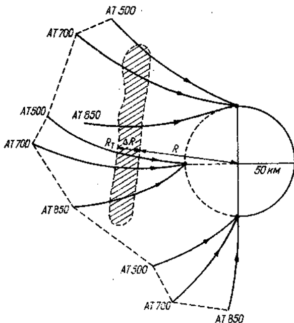
Черт. 5.11. Схематическое определение границ области предполагаемой адвекции облачных элементов и параметров РОЗО (заштрихованная полоса) в район прогноза ( R = 50 км от МРЛ) по данным МРЛ при заблаговременности T = 12 ч.
