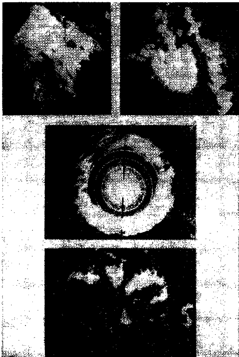
Черт. 2.17. Картины радиоэха различных облачных систем, наблюдаемые на ИКО.
