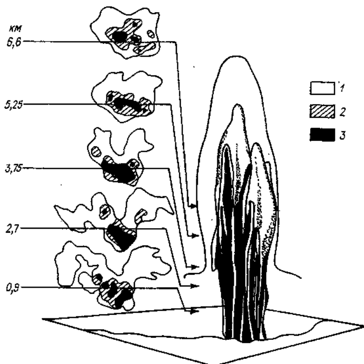
Черт. 2.9. Трехмерное распределение отражаемости в градовом облаке (по Стауту и Уилку).
