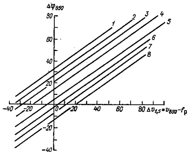
Черт. 4.5. Номограмма для определения угла отклонения \Delta\varphi_{850} для ячеек радиоэха и малых мезомасштабных площадей в зависимости от разности скорости ветра и скорости радиоэха ( v_{850} - f_p ), а также величины поворота ветра в вертикальном слое 5,5—1,5 км \Delta d_1 = (d_{d500} - d_{d850}) .
