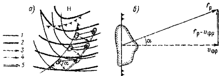
Черт. 4.2. Схематическое изображение холодного фронта (а) и векторная диаграмма движения ячейки радиоэха и фронта (б).
