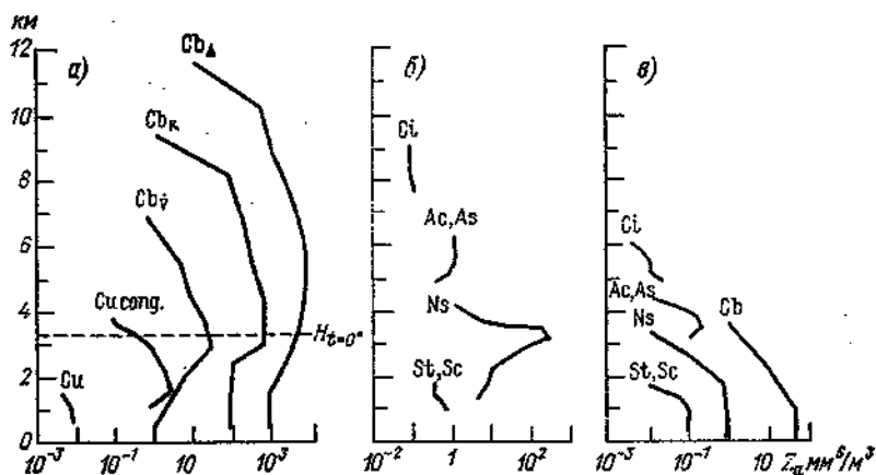
Черт. 2.16. Вертикальное распределение отражаемости Z_a в облаках.
