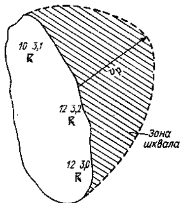
Черт. 5.16. Расположение зоны шквала относительно РКО.
