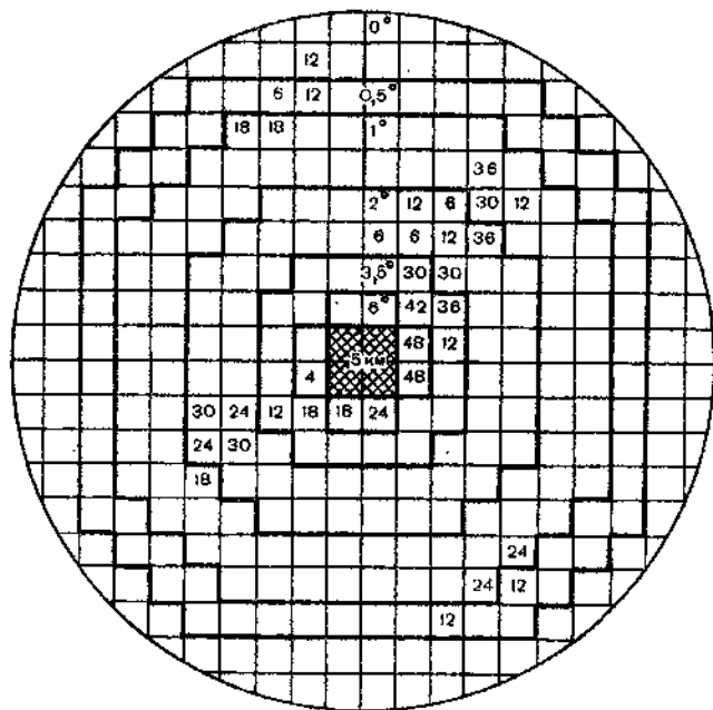
Черт. 3.2. Пример записи значений P_{\text{пр}}/P_0 на шаблоне для высоты 5 км.
