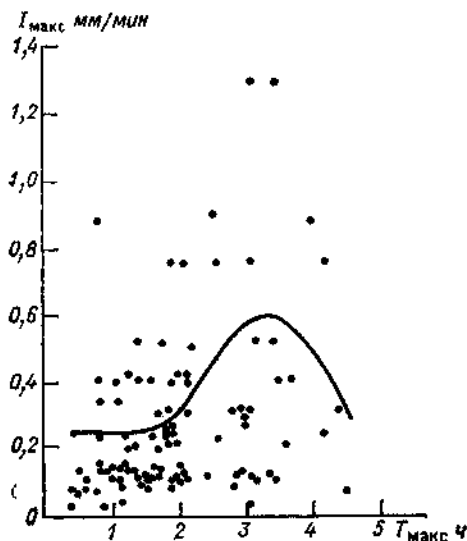
Черт. 2.5. Осредненная зависимость между максимальной интенсивностью осадков I_{\max} и продолжительностью существования очага T_{\max} .
