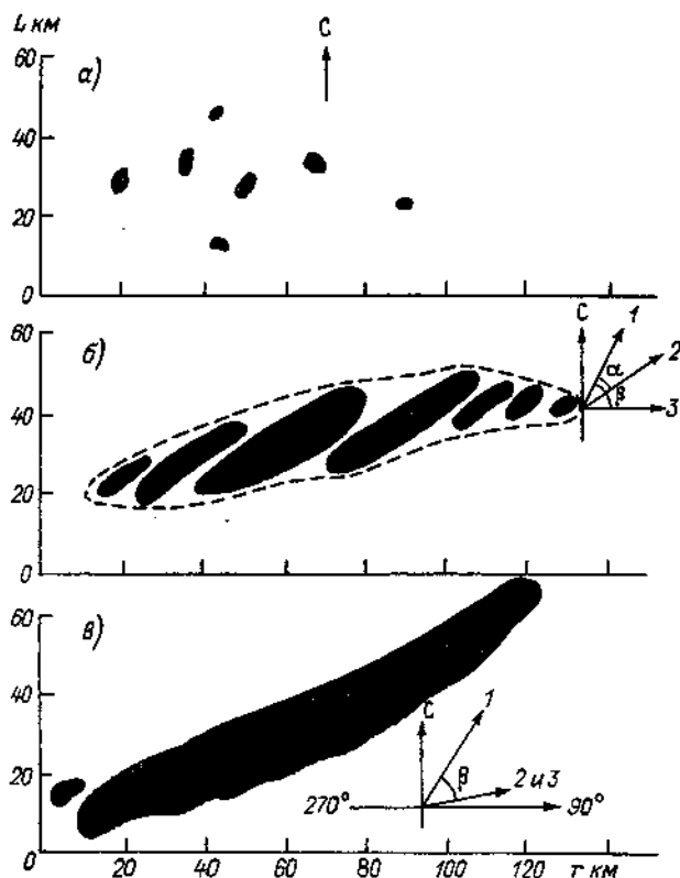
Черт. 2.11. Схема карты градобитий при одноячейковых (а), многоячейковых (б), суперячейковых (в) процессах.
