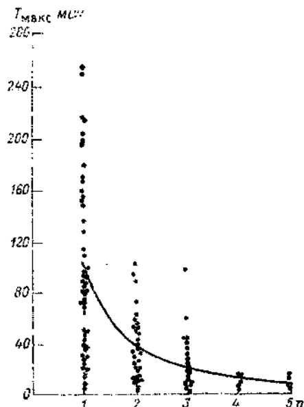
Черт. 2.7. Осредненная зависимость между временем существования очага T_{\max} и степенью его раздробленности.
