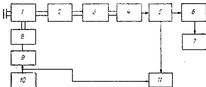
Черт. 7.1. Схема подключения приборов для измерения чувствительности и градуировки системы ступенчатого изюха МРЛ-1.
