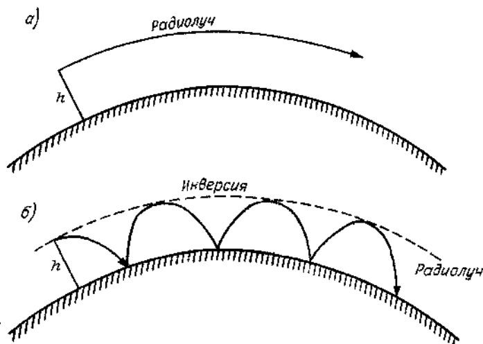
Черт. 1.8. Радиолуч над поверхностью Земли.
