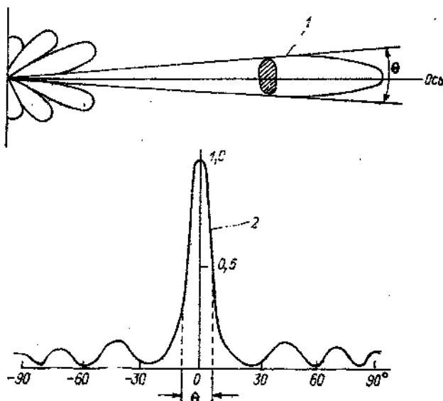
Черт. 1.3. Диаграмма направленности антенны.
