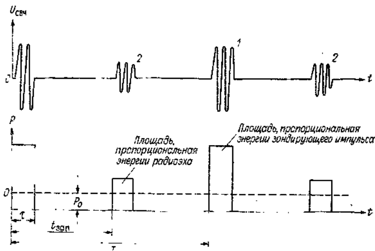
Черт. 1.2. Иллюстрация импульсного метода работы радиолокатора.
