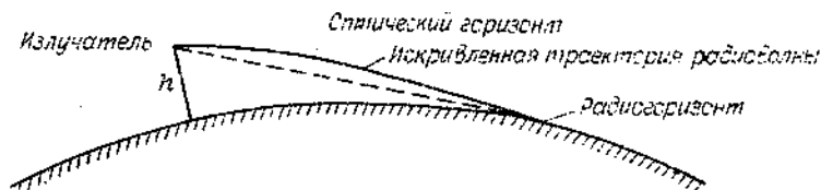
Черт. 1.5. Радиогоризонт и оптический горизонт.
