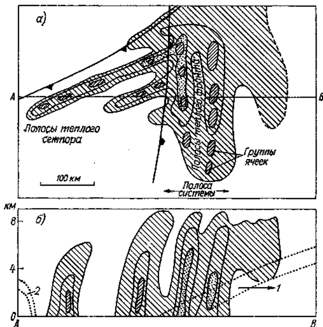
Черт. 5.2. Типизированное изображение зон радиозахвата синоптического масштаба в окклюдированном циклоне и связанных с осадками систем теплового и холодного фронтов.
