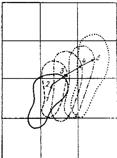
Черт. 4.3. Определение параметров движения отдельной ячейки (по смещению условного центра оконтуренной зоны).
