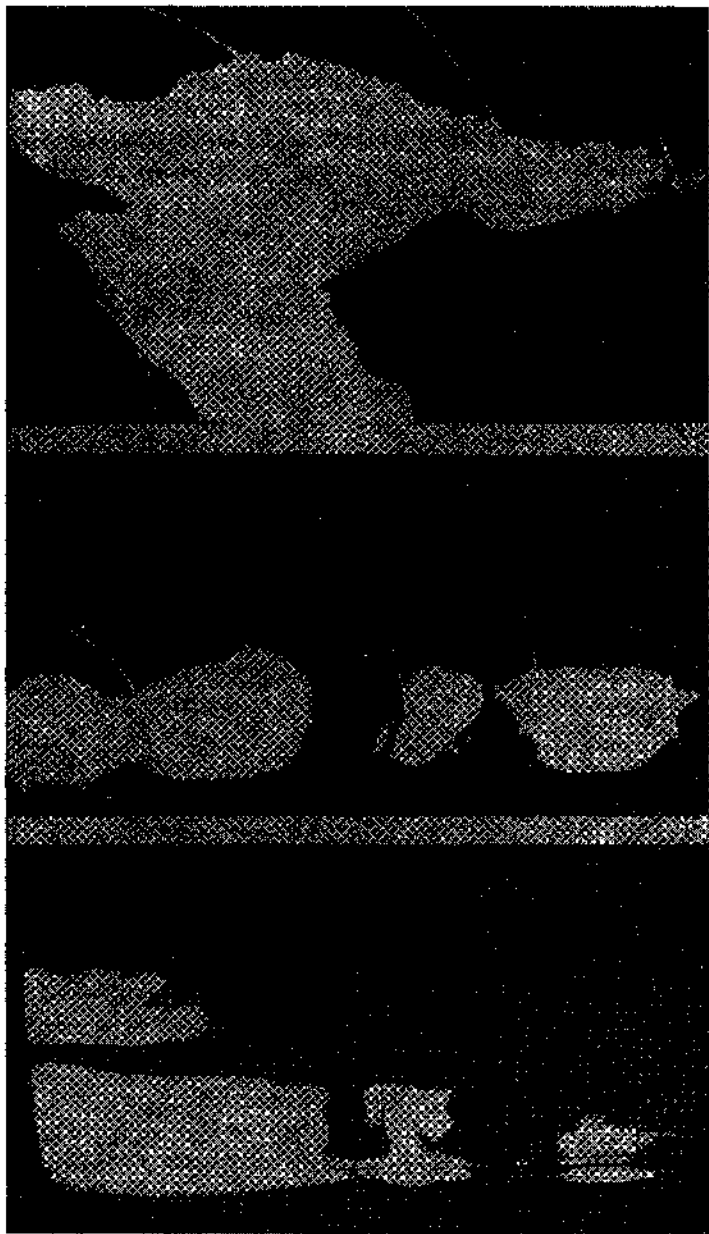
Черт. 2.14. Типичные картины радиоза различных форм облаков в летний период года (верхние фото) и зимний период (нижнее фото).
