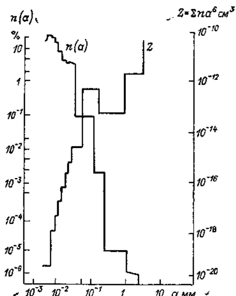
Черт. 1.13. Распределение отражаемости Z и размеров капель в облаках и осадках.
