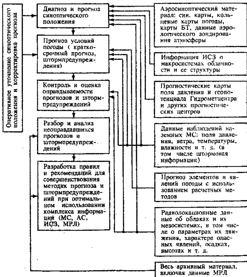
Черт. 5.12. Схема использования наземной, спутниковой и радиолокационной информации в синоптическом анализе при разработке и контроле оправданности прогнозов погоды.
