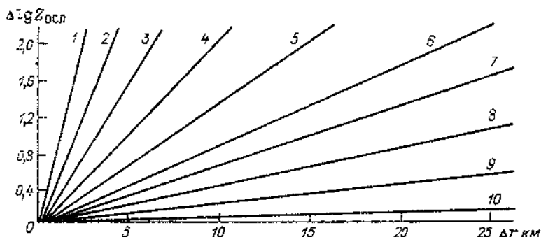
Черт. 1.16. График для расчета поправок отражаемости ( \Delta \lg Z ) осл в зависимости от интенсивности экранирующих осадков I (мм/ч) и протяженности зоны осадков \Delta r (км).
