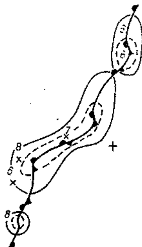
Черт. 5.7. Волны на холодном фронте при несплошном радиоэхе. Район Балхаша.
