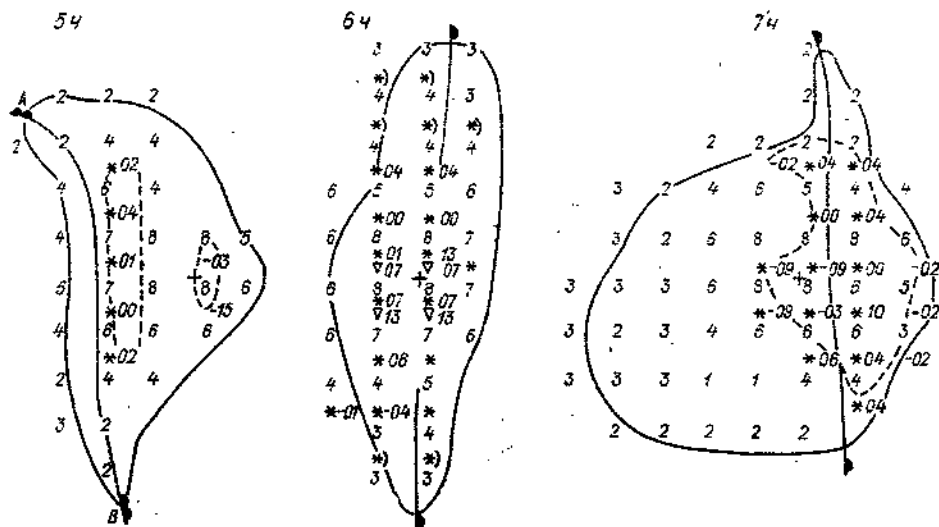
Черт. 5.3. Радиоэхо облачности и осадков теплого фронта, перемещающегося к востоку, за 28 января 1987 г.
