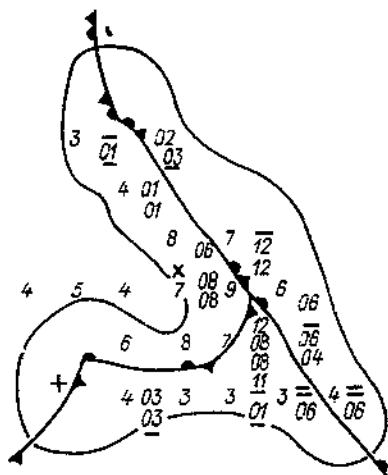
Черт. 5.9. Радиоэхо облачности и осадков за 03 ч 19 июля 1980 г. Район Актыюбанска.
