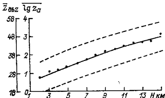
Черт. 9.3. Экспериментальная зависимость между средним арифметическим значением \lg Z и высотой радиоэха гроз и ливней.
