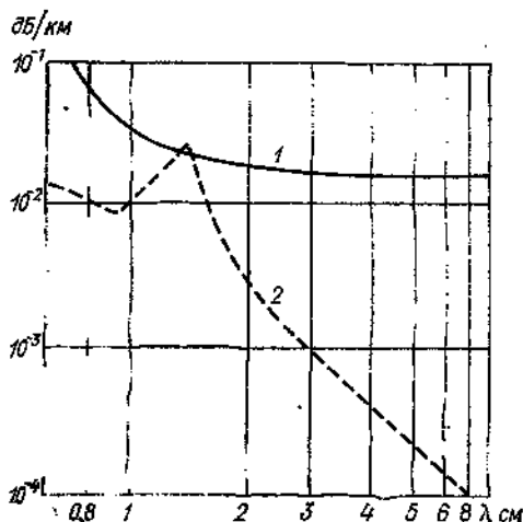
Черт. 1.14. Ослабление (дБ/км) радиоволн сантиметрового диапазона кислородом (1) и водяным паром (2) при t = 20^\circ\text{C} для различных \lambda (по Ганну и Исту).
