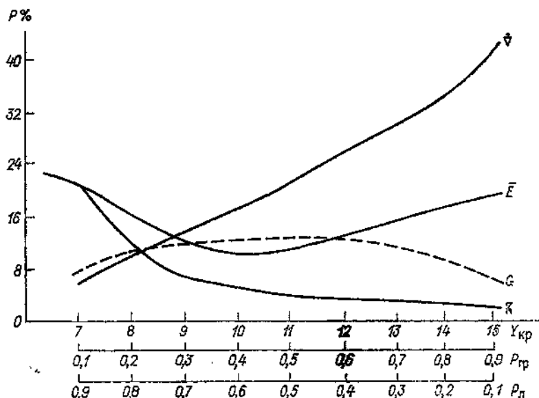
Черт. 2.19. Зависимости средних ошибок распознавания P (%) гроз ( \nabla ), ливней ( \nabla ) и суммарной ошибки распознавания для критерия грозоопасности Y_{кр} ( E ) и единой обучающей выборки ( G ) от априорной вероятности появления гроз P_{гр} и ливней P_{л} .
