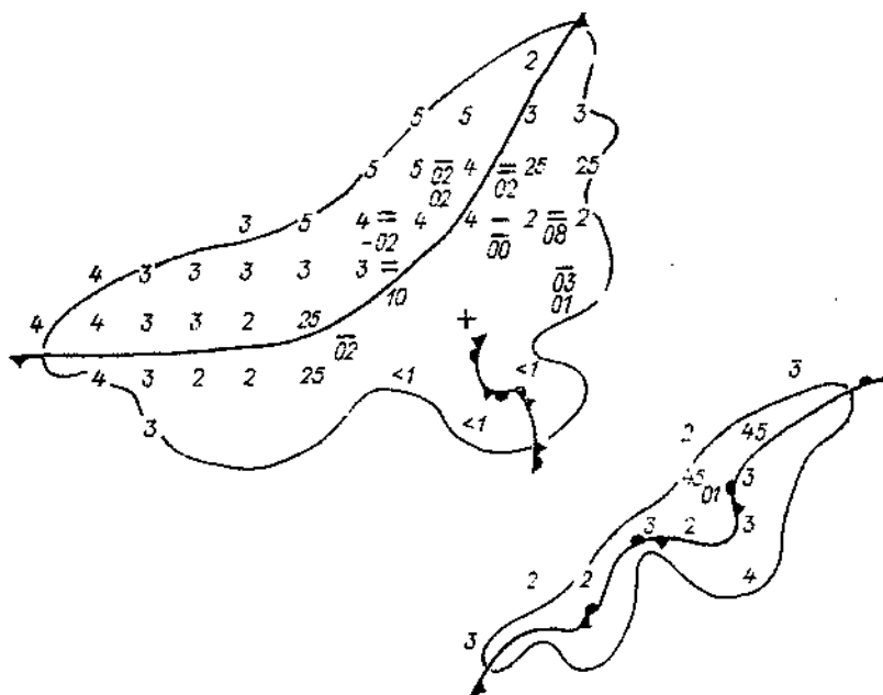
Черт. 5.8. Радиоэхо облачности и осадков за 09 час 20 апреля 1981 г. Район Балахша.
