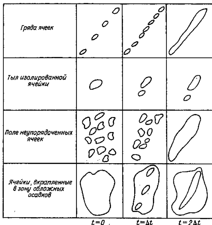
Черт. 2.12. Классификация процесса формирования линий шквалов.
