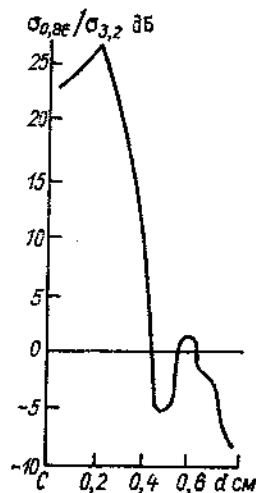
Черт. 1.11. Отношение \sigma_{0,86}/\sigma_{3,2} в зависимости от диаметра водяной сферы.
