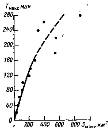
Черт. 2.6. Осредненная зависимость между временем существования очага T_{\max} и максимальным значением занимаемой им площади S_{\max} .
