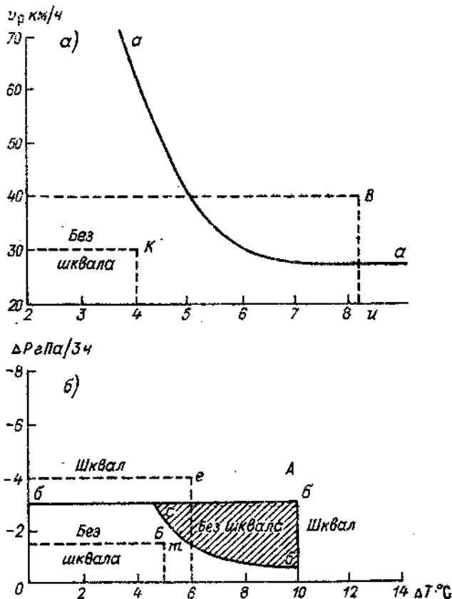
Черт. 5.13. Графики для диагноза шквала со скоростью более 25 м/с по уточненному синоптико-радиолокационному варианту метода прогноза шквалов.
