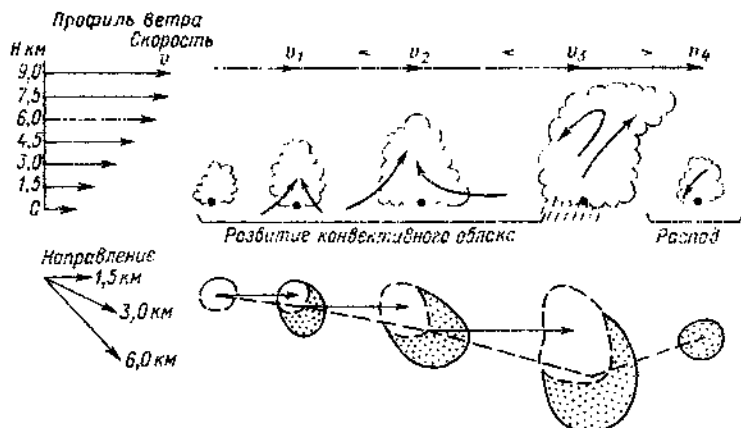
Черт. 4.1. Условная модель взаимодействия облака и потока окружающей среды для случая переменного по вертикали ветра и трансформирующегося Сб.
