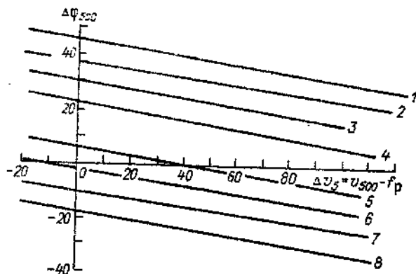
Черт. 4.6. Номограмма для определения угла отклонения \Delta\varphi_{500} радиоэха БМП в зависимости от разности скорости ветра и скорости движения зоны радиоэха ( v_{500} - f_p ), а также величины поворота ветра в вертикальном слое 5,5—1,5 км
