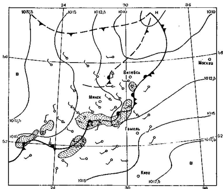
Черт. 5.1. Схематическое изображение малоподвижного холодного фронта с волнами и данных МРЛ (зоны, обозначенные точками) по кольцовке БТГМЦ (М 1:2 500 000) за 06 (09) ч 8 мая 1972 г.
