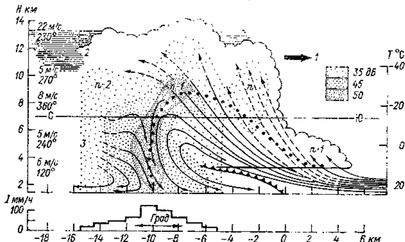
Черт. 2.3. Схематическое изображение мультячейковой грозы с градом 9 июля 1973 г. Раймер, штат Колорадо: вертикальный разрез вдоль направления движения грозы.
