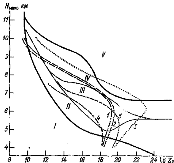
Черт. 2.18. Соотношение гроз и ливней в пространстве параметров H_{\text{макс}} , \lg Z_3 по зонам I—V (сплошные линии — границы зон); зависимость квадратичной дискриминантной функции u(H_{\text{макс}}, \lg Z_3, H_{-22}^{\circ}\text{C}) единой обучающей выборки от H_{-22}^{\circ}\text{C} .
