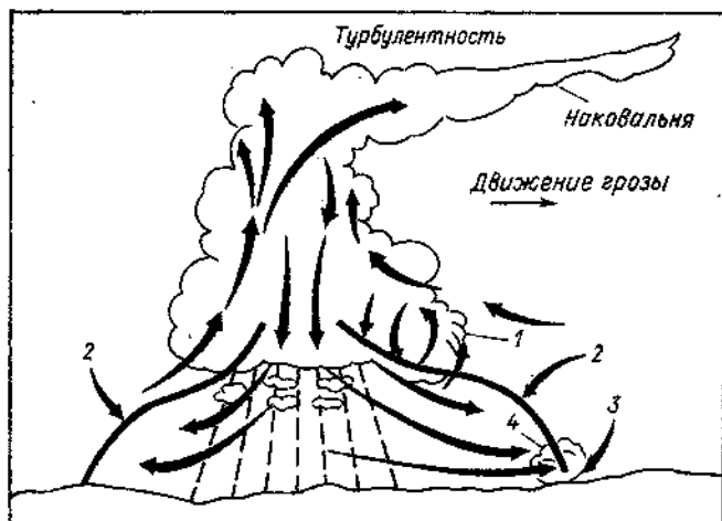
Черт. 2.1. Грозовое кучево-дождевое облаков в стадии развития с сопровождающими его опасными явлениями.
