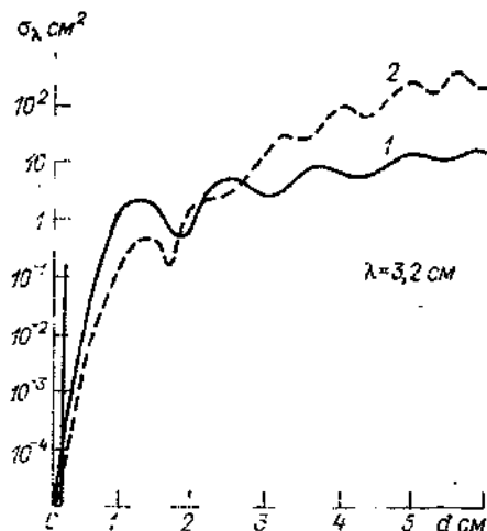
Черт. 1.9. Изменение эффективной площади рассеяния \sigma_\lambda водяной (1) и ледяной (2) сферических частиц на длине волны 3,2 см.
