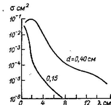
Черт. 1.10. Зависимость эффективной площади рассеяния \sigma водяных сфер разного диаметра от длины волны.
