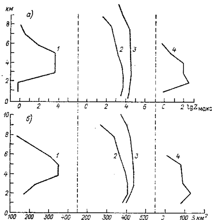
Черт. 2.10. Типичные профили отражаемости ( \lg Z ) и площади, занятой радиоэхом S(H) , в стадии развития (1), зрелости (2, 3) и распада (4) кучево-дождевого облака.
