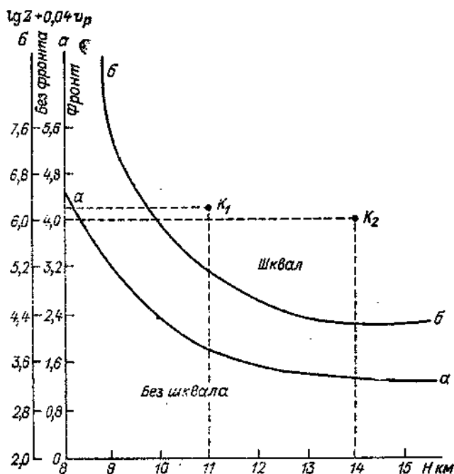
Черт. 5.15. График для определения ситуации без шквала.
