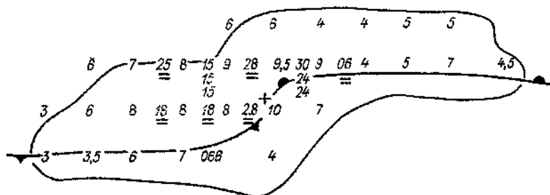
Черт. 5.6. Волна на холодном фронте. Район Алма-Аты.
