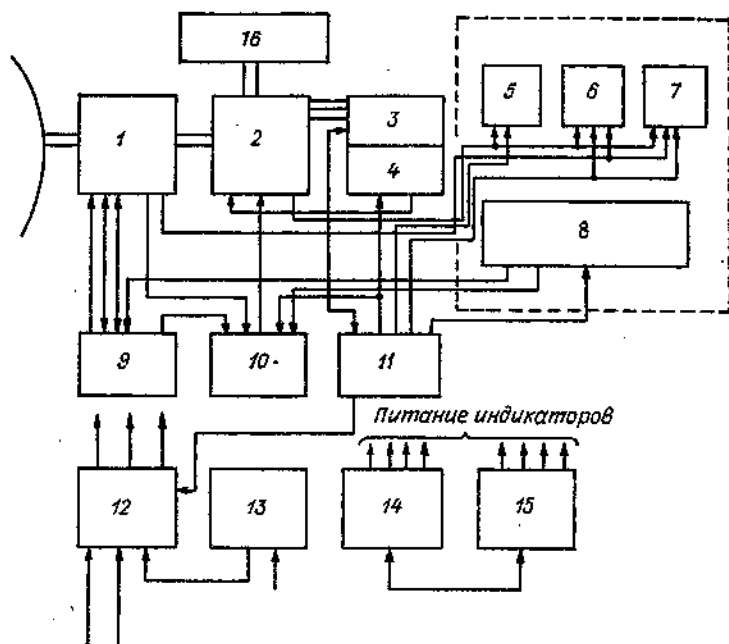
Черт. 6.5. Функциональная схема МРЛ-2.
