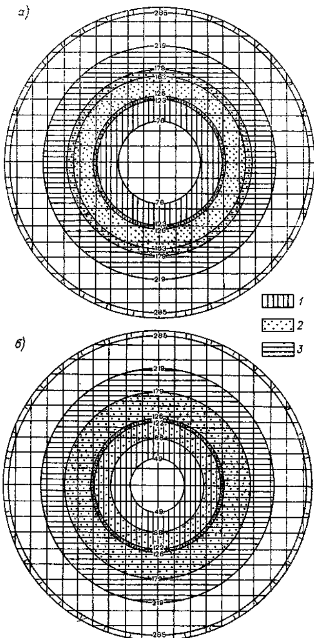
Черт. 2.23. Зоны пересечения диаграмм направленности антенны угла возвышения антенны
