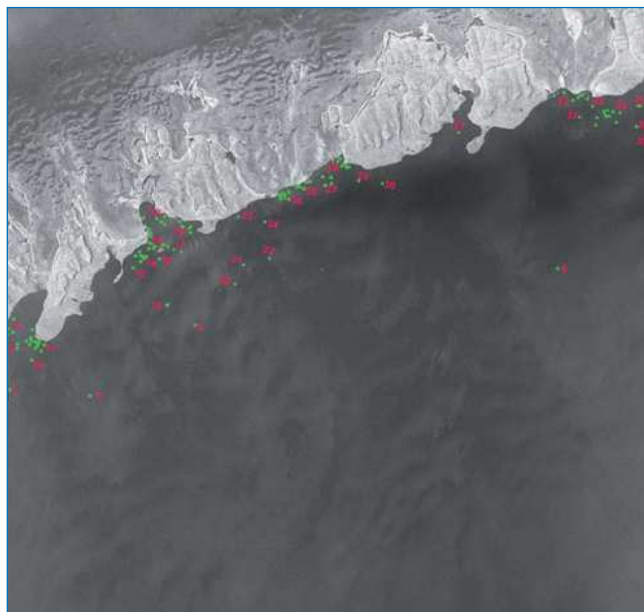
Расположение обнаруженных обломков айсбергов в прибрежной зоне Новой Земли 8 августа 2012 г. по данным IC3 Radarsat-2, режим S, размер кадра 100×100 км.
