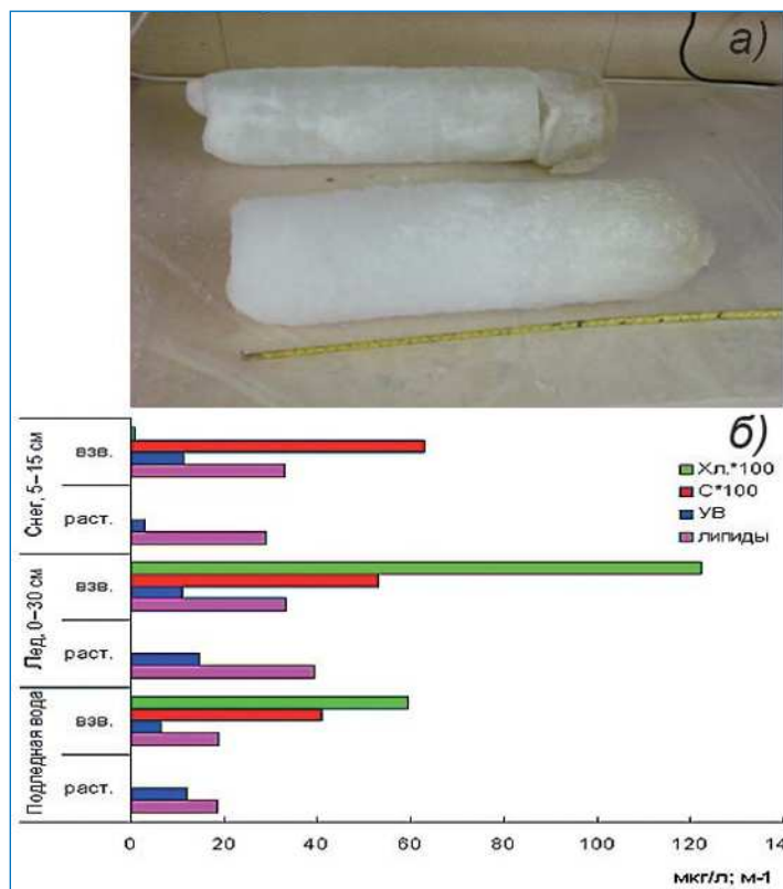
Рис. 5. Фотография кернов льда (а) и концентрации органических соединений и взвеси (б) в снежно-ледяном покрове оз. Степпед в 2012 г.
