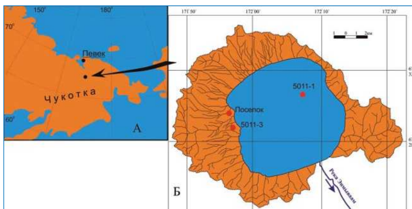
Расположение (А) и схема бассейна (Б) озера Эльгыгытгын с указанными местами расположения буровых скважин и бурового поселка.
