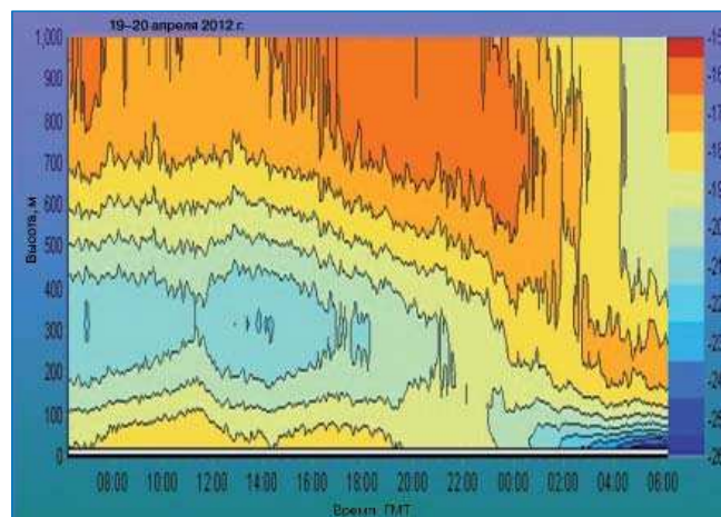
Рис. 2. Временная изменчивость термической структуры нижнего слоя атмосферы на СП-39 по данным профилера МТП-5РЕ.
