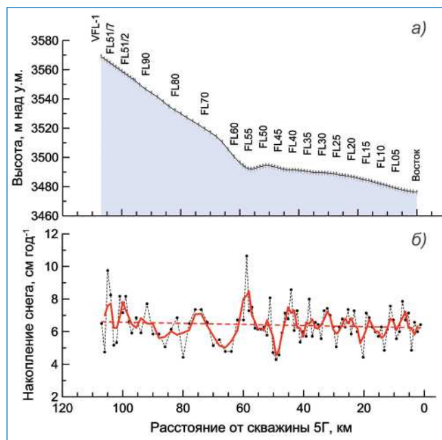
Рис. 3. Результаты походовых гляциологических исследований: а – высота поверхности ледника по профилю VFL; б – пространственное распределение снегонакопления.
