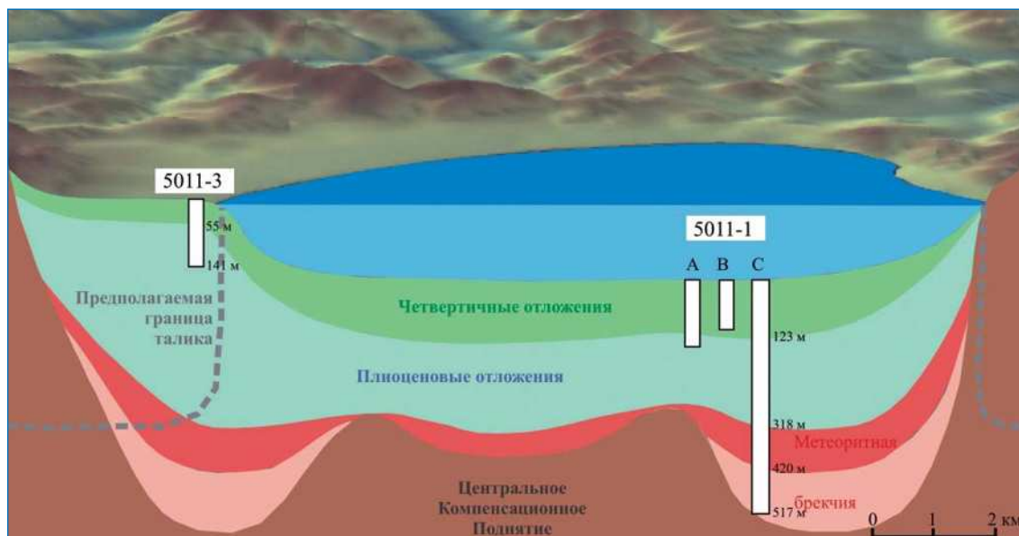
Схематический разрез через котловину озера Эльгыгитгын.
