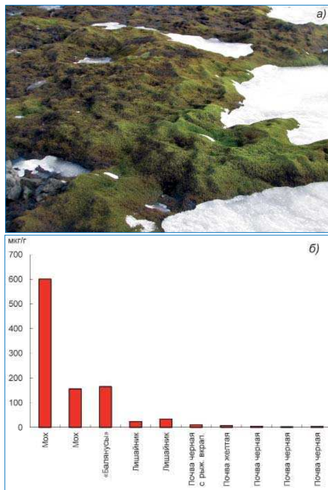
Рис. 7. Фотография мхов (а) и концентрации УВ в мхах, лишайниках и почвах (б) на берегу озера Китеж, ст. Беллингаузен.
