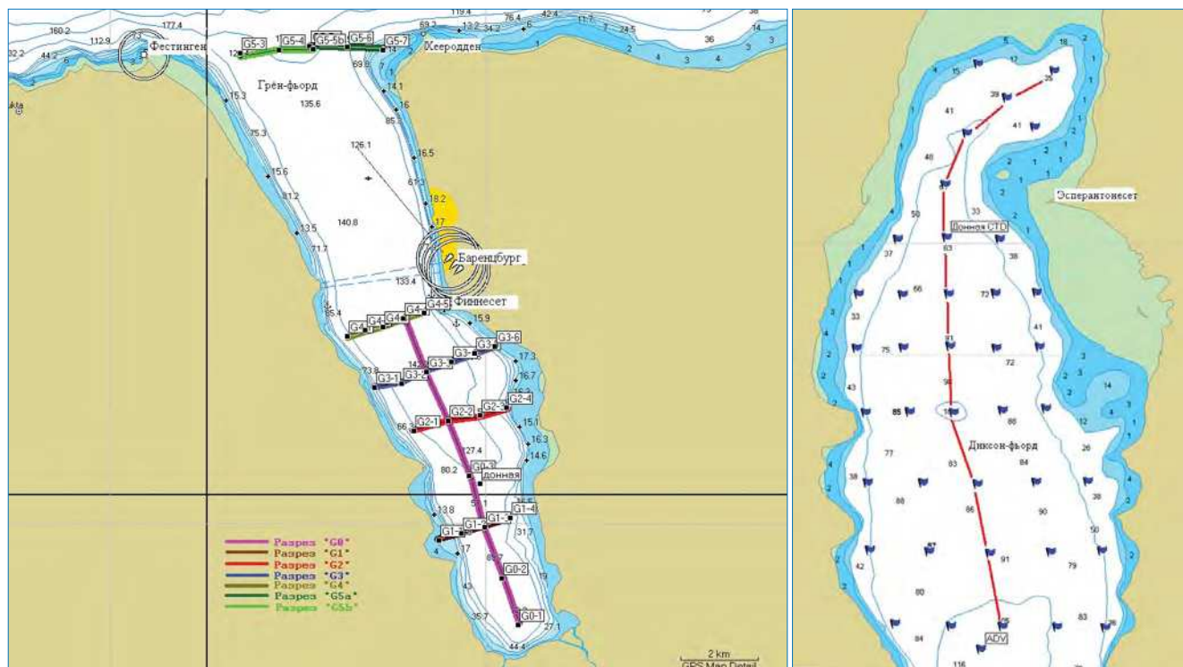
Положение океанографических станций и ориентация разрезов в заливе Грэн-фьорд (слева) и в заливе Диксон-фьорд (справа).
