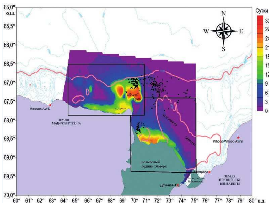
Рис. 1. Повторяемость существования полыней (областей открытой воды) в заливе Прюдс в июне (в сутках) за 2009–2021 годы по данным микроволнового спектрометрического AMSR-2. Точками показаны места всплытия морских млекопитающих в июне за весь период реализации программы МЕОР
