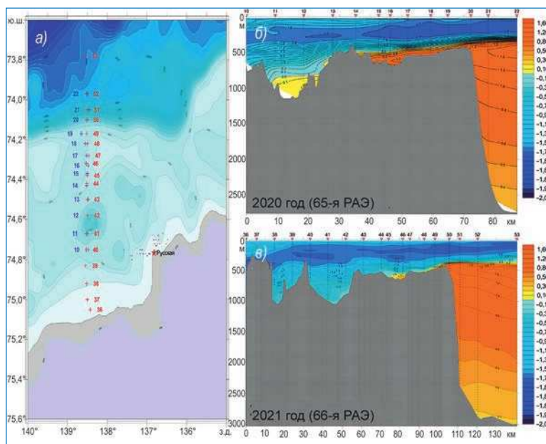
Рис. 3. Схема работ в районе станции Русская: а) расположение станций в 2020 (синие значки) и в 2021 (красные значки) годах; потенциальная температура на разрезе 138^{\circ}30' з. д. в 2020 (б) и 2021 (в) годах
