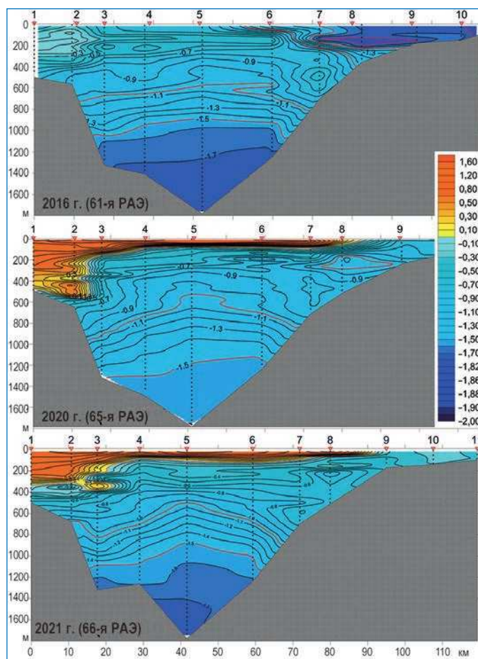
Рис. 5. Потенциальная температура на разрезе в проливе Брансфилд в период работ 61-й, 65-й и 66-й РАЭ
