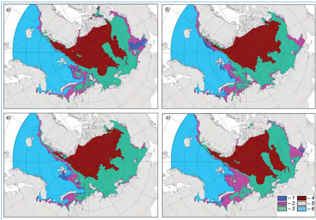
Рис. 3. Распределение морских льдов разного возраста по данным картирования ААНИИ ( http://wdc.aari.ru/datasets/ssmi/data/north/extent/ ):
