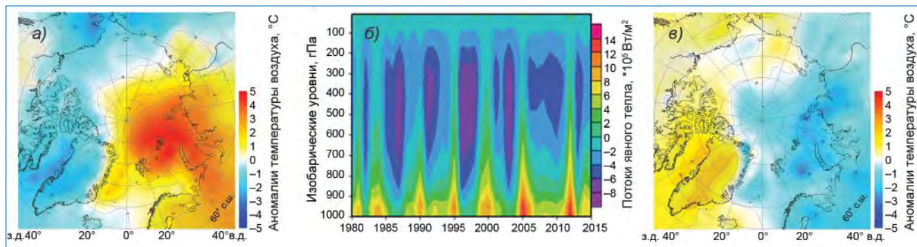
Рис. 2. Влияние меридиональных атмосферных переносов тепла (МАПТ) на аномалии зимней приповерхностной температуры воздуха (ПТВ) в Арктике: а — средние аномалии зимней ПТВ в годы больших значений МАПТ; б — средние за зиму МАПТ через 0 – 80^\circ в.д. на изобарических уровнях за 1980–2015 гг. (Алексеев Г.В., Кузмина С.И., Уразгильдеева А.В., Бобылев Л.П. Влияние атмосферных переносов тепла и влаги на усиление потепления в Арктике в зимний период // Фундаментальная и прикладная климатология. 2016. Т. 1. С. 43–63); в — средние аномалии зимней ПТВ в годы с малыми значениями МАПТ. Аномалии ПТВ рассчитаны по данным реанализа Interim ( www.ecmwf.int/en/research/climate-reanalysis/era-interim ) относительно среднего за 1979–2015 гг.
