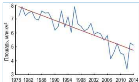
Среднесуточное изменение площади арктического морского льда в сентябре 1979–2014 годов.
