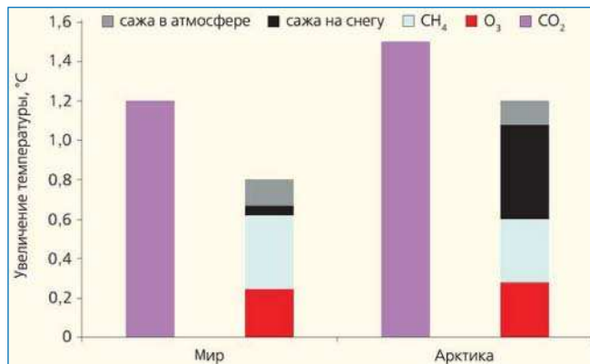
Увеличение температуры приземного воздуха относительно доиндустриального периода, обусловленное изменениями содержания CO 2 и короткоживущих климатических загрязнителей во всем мире и отдельно в Арктике.
