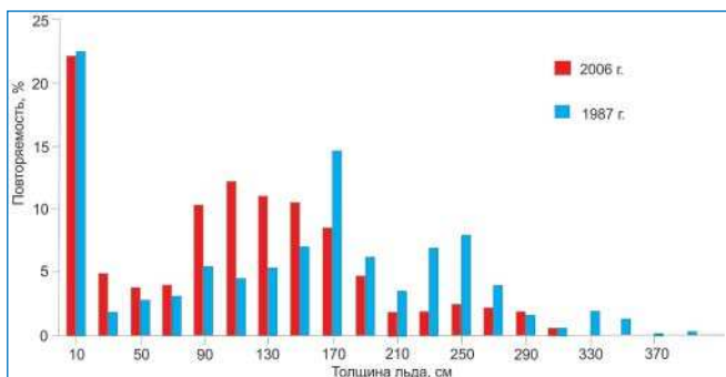
Распределение толщины ровного льда в мае на пути плавания атомных ледоколов «Ямал» в 2006 году и «Сибирь» в 1987 году. Из Второго оценочного доклада Росгидромета об изменении климата и их последствиях на территории Российской Федерации http://downloads.igce.ru/publications/OD_2_2014/v2014/htm/ .
