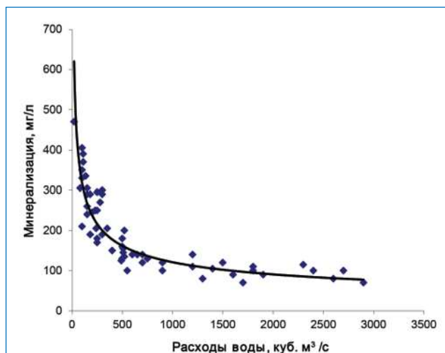
Рис. 1. Связь минерализации и расхода воды для р. Онега (с. Порог).
