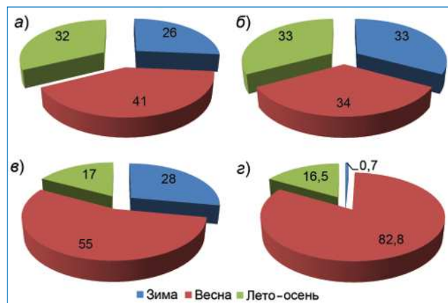
Рис. 6. Внутригодовое распределение в процентах ионного стока в замыкающих створах рек Оби (а), Печоры (б), Оби (в) и Яны (г).
