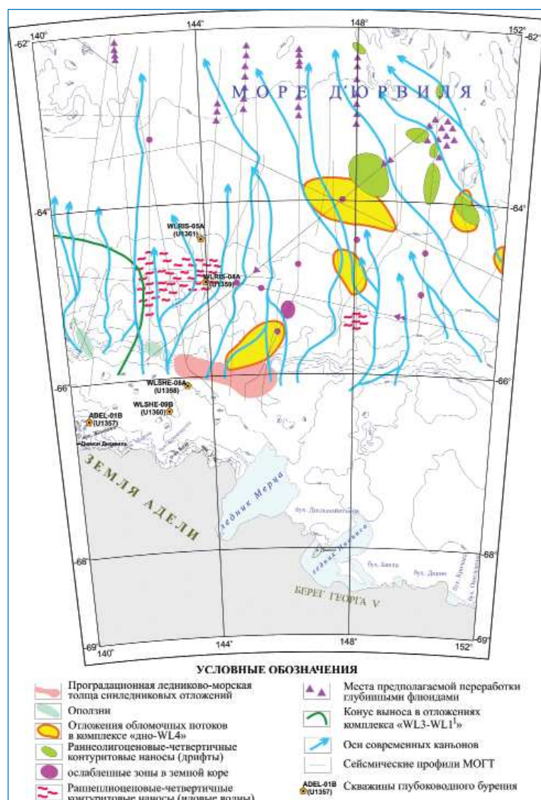
Рис. 2. Схема распространения осадочных фаций в доледниковых и синледниковых осадках бассейна моря Д'Юрвиля
