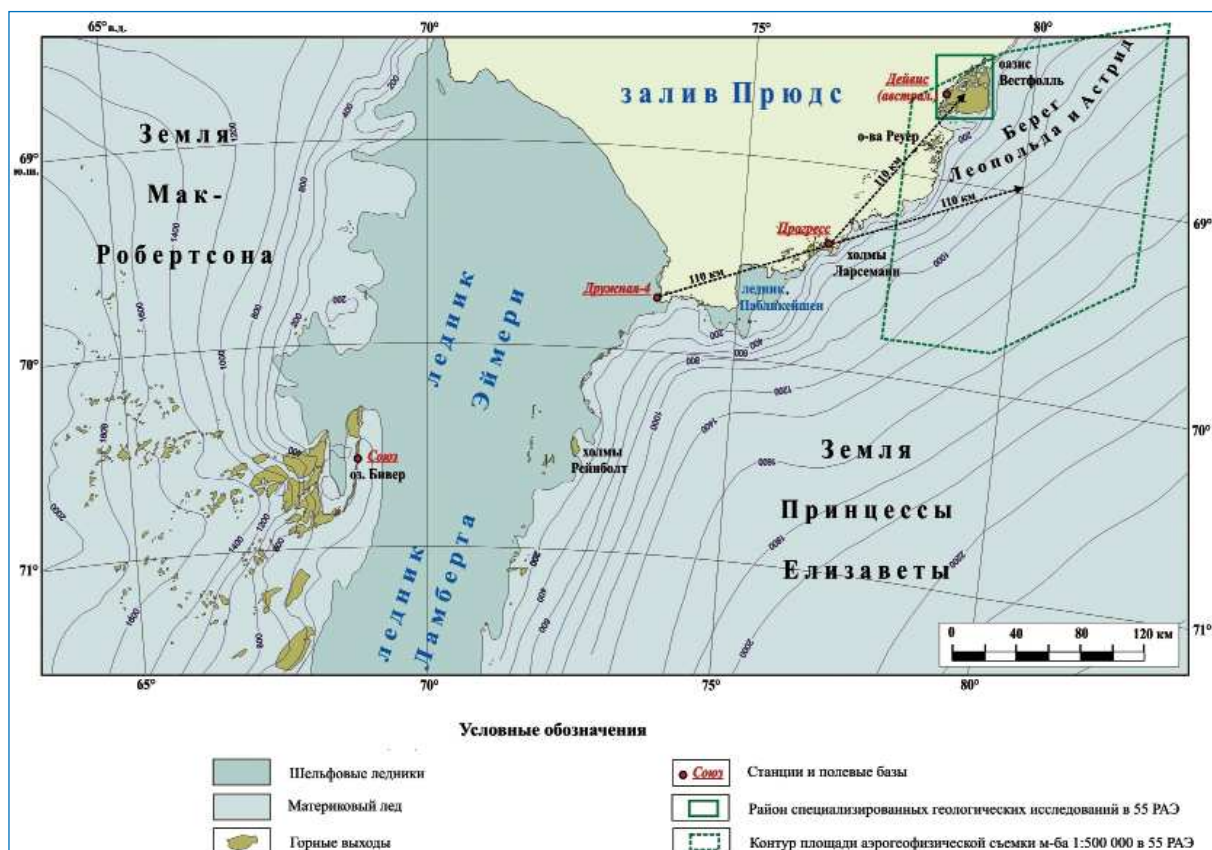
Схема расположения районов геолого-геофизических работ в 55-й РАЭ на Земле Принцессы Елизаветы
